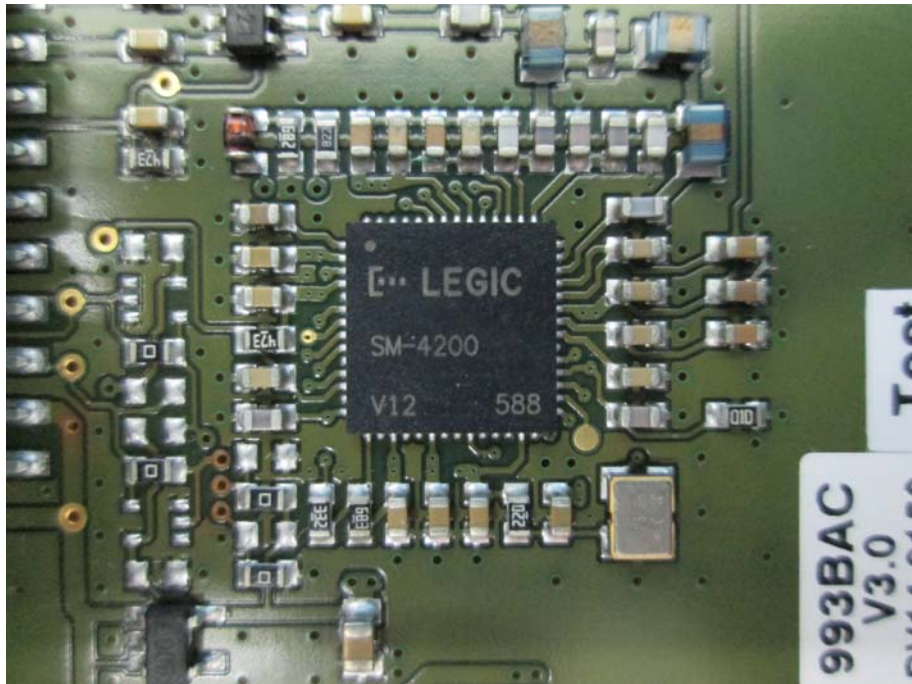
NFC Module
