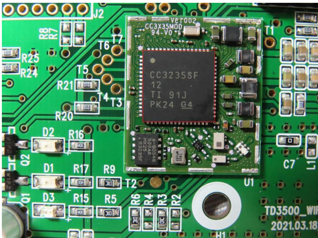
WLAN Module
