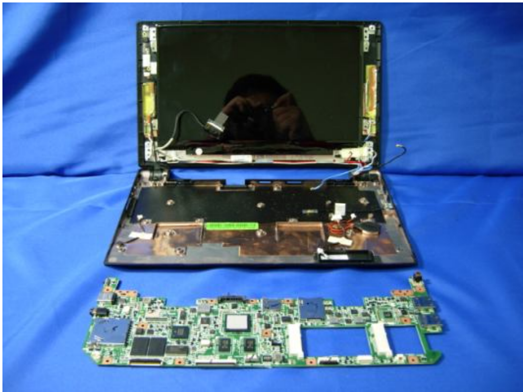
(36) EUT Photo
