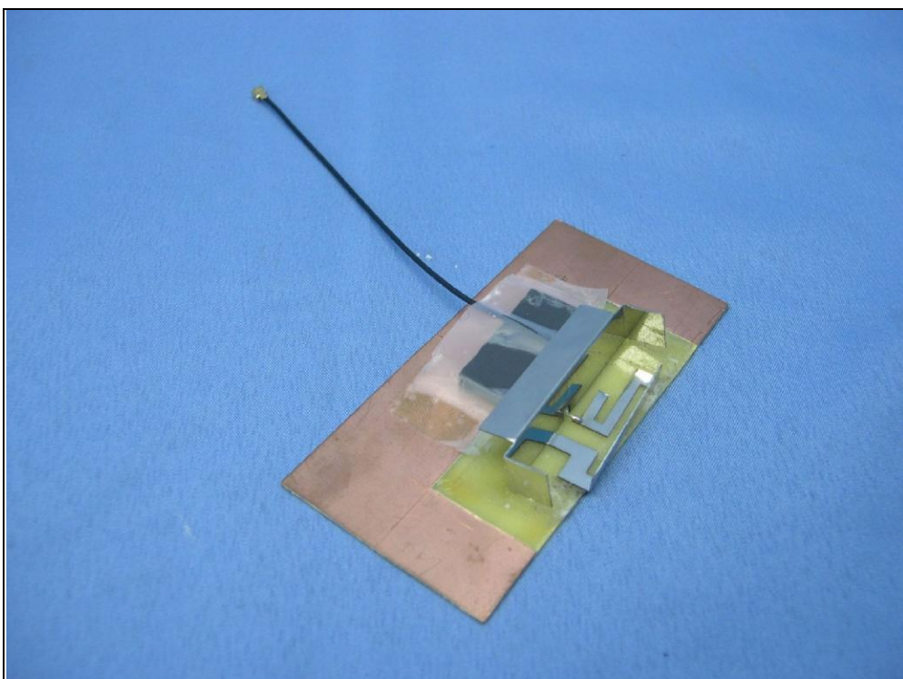
Antenna: MSA-4008-25GC1-A1
