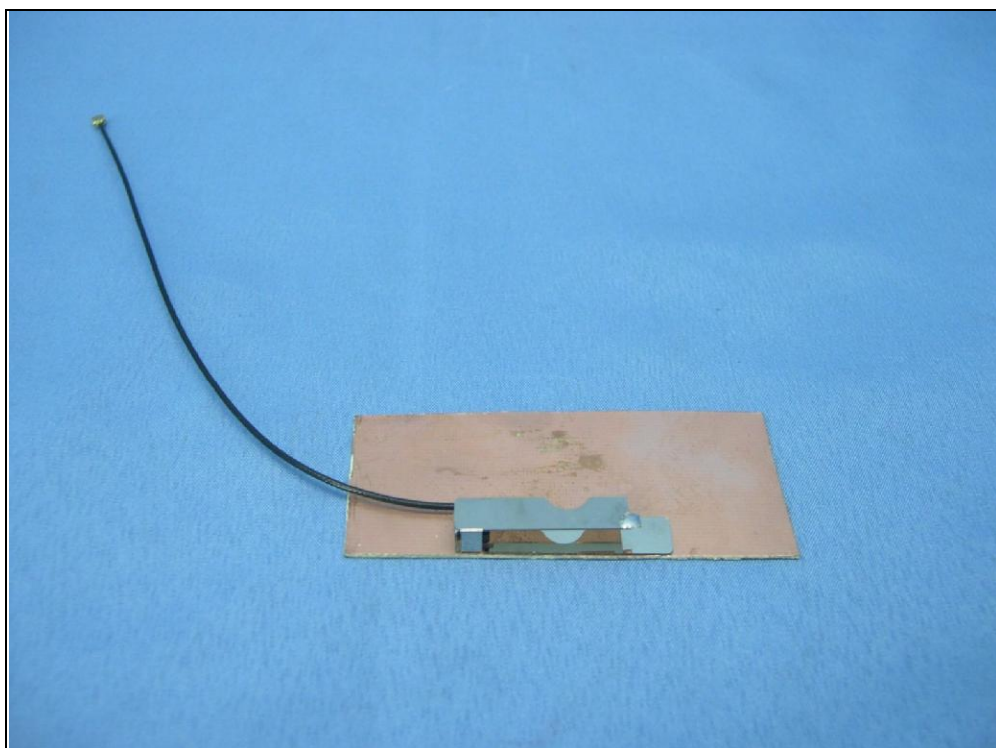
Antenna: MSA-3305-2G4C1-A1
