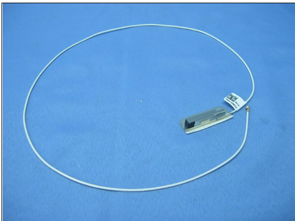
Antenna: 81XCAE15.G07
