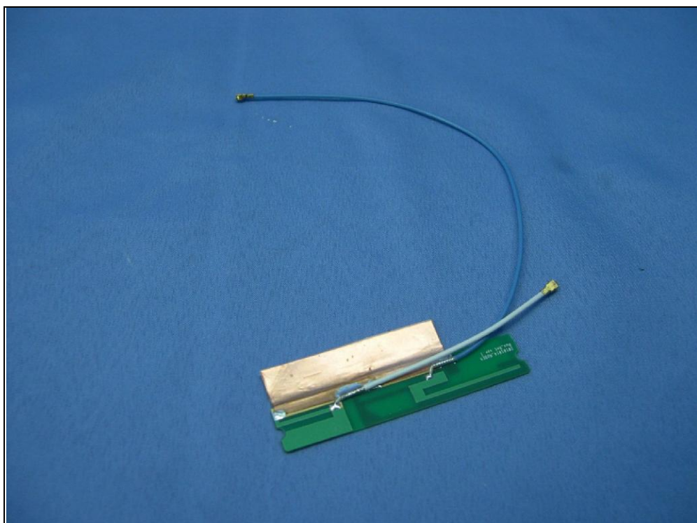
Antenna: 150872-30
