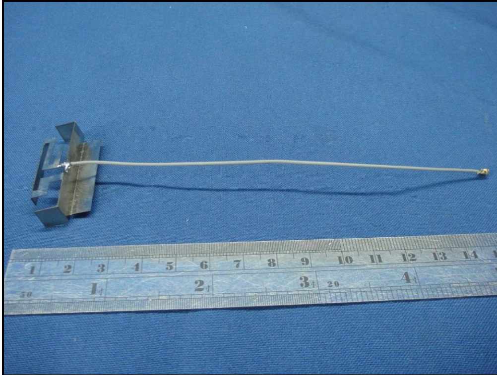
Antenna: MS-A4008-25GC1-A1
