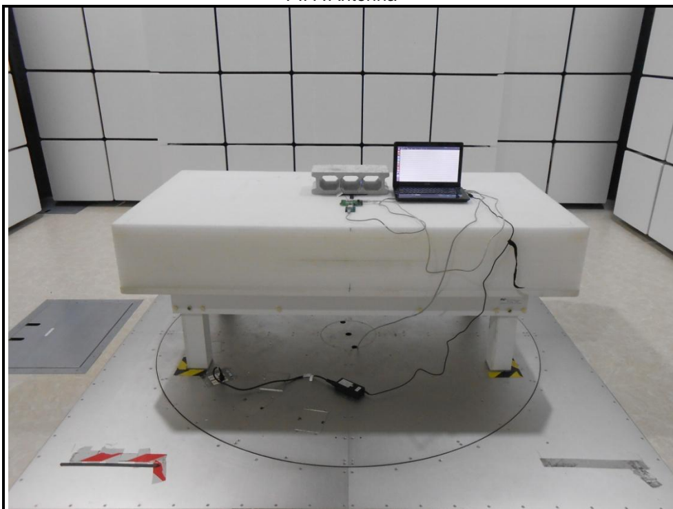
PIFA Antenna
