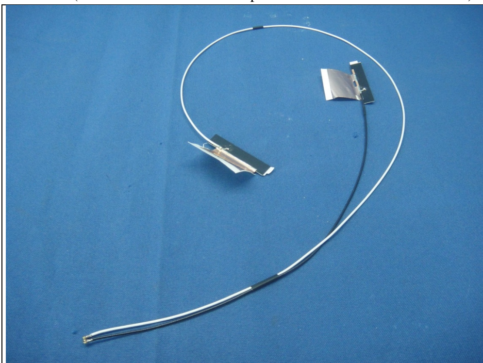
Antenna (Brand: Wistron NeWeb Corporation / Model: 81EAAX15.G12)
