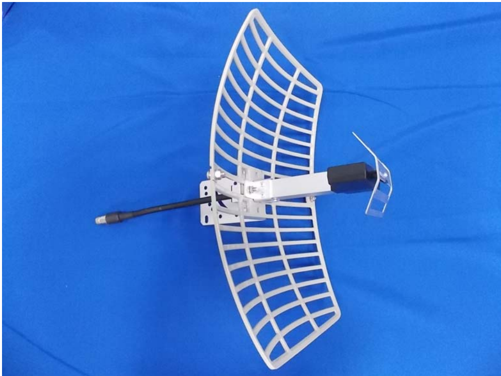
(4) EUT Photo (Antenna AG-24015)
