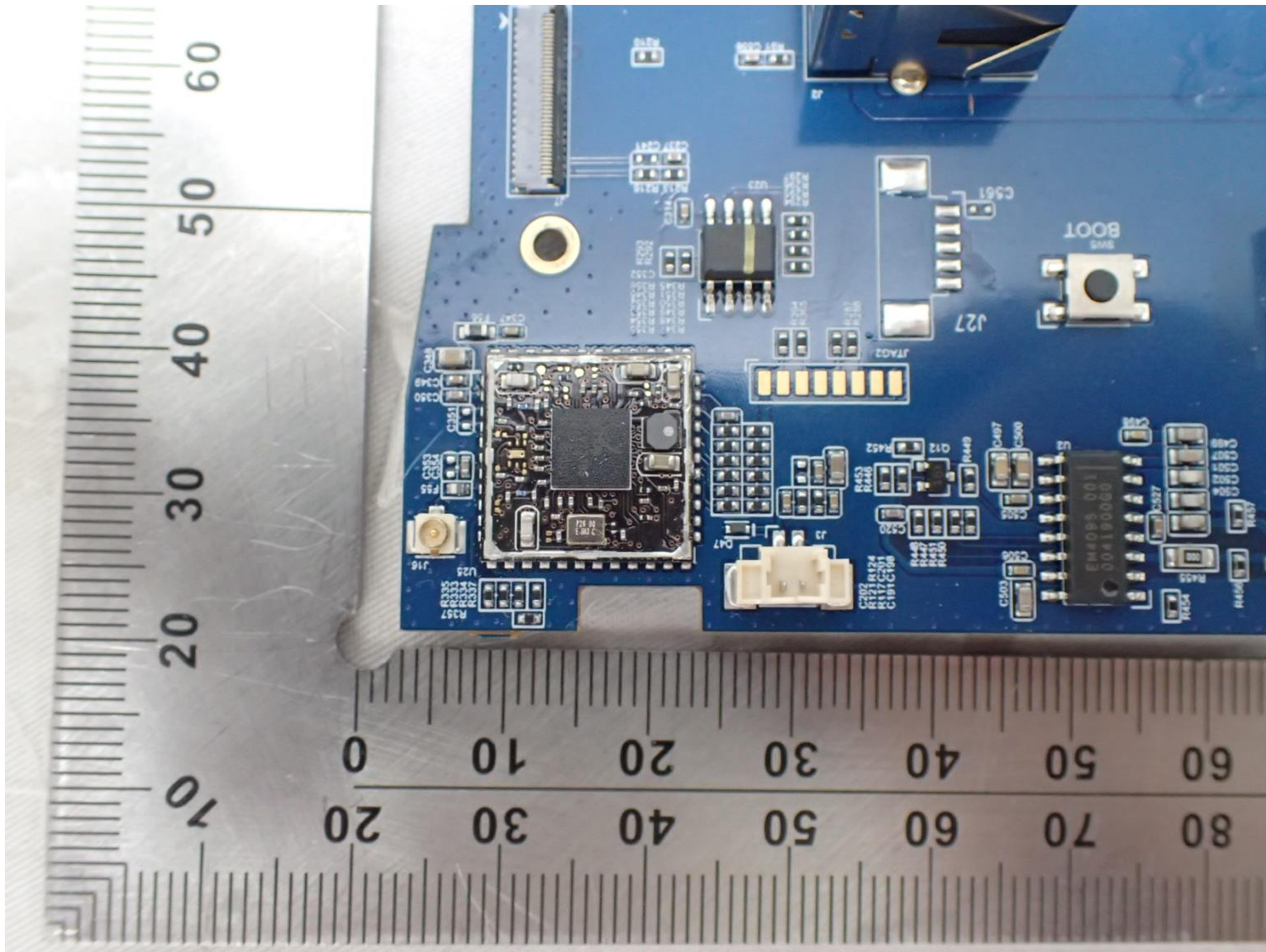
RF Module(WLAN)
