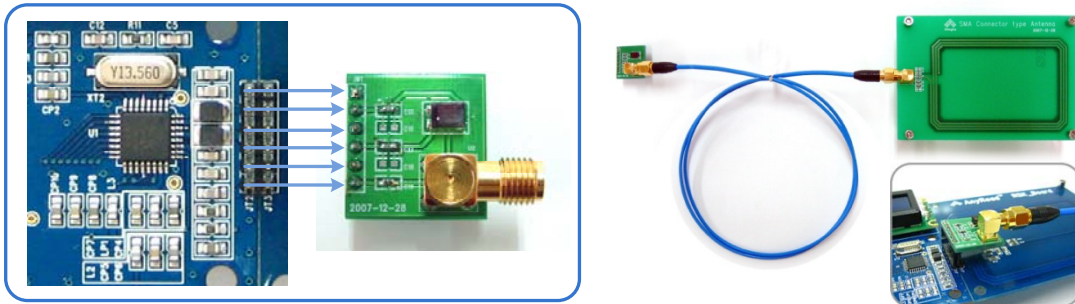
『 RFLEVK01 - 50ohm matching system 』
