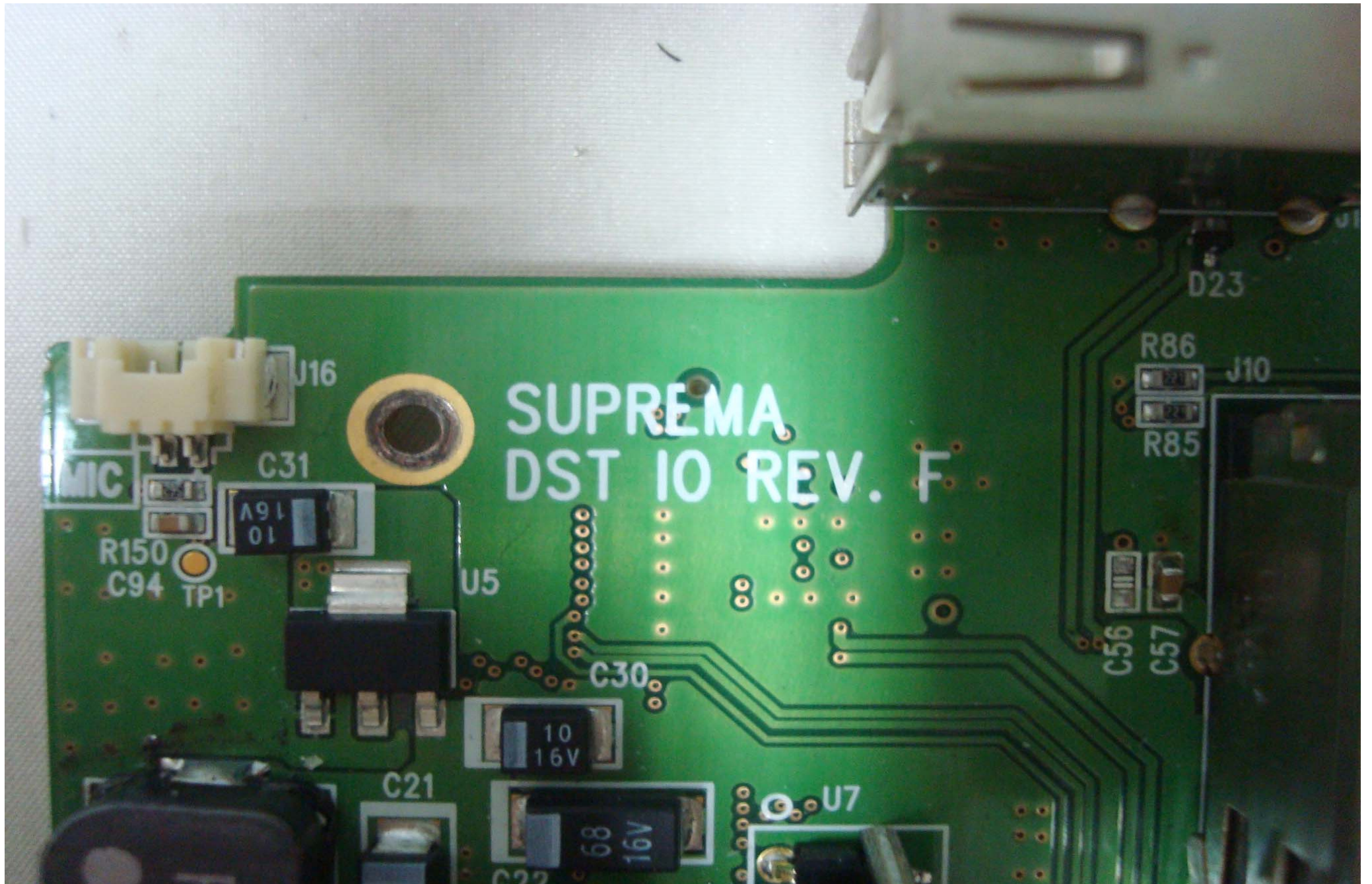
IO BOARD 라벨면
