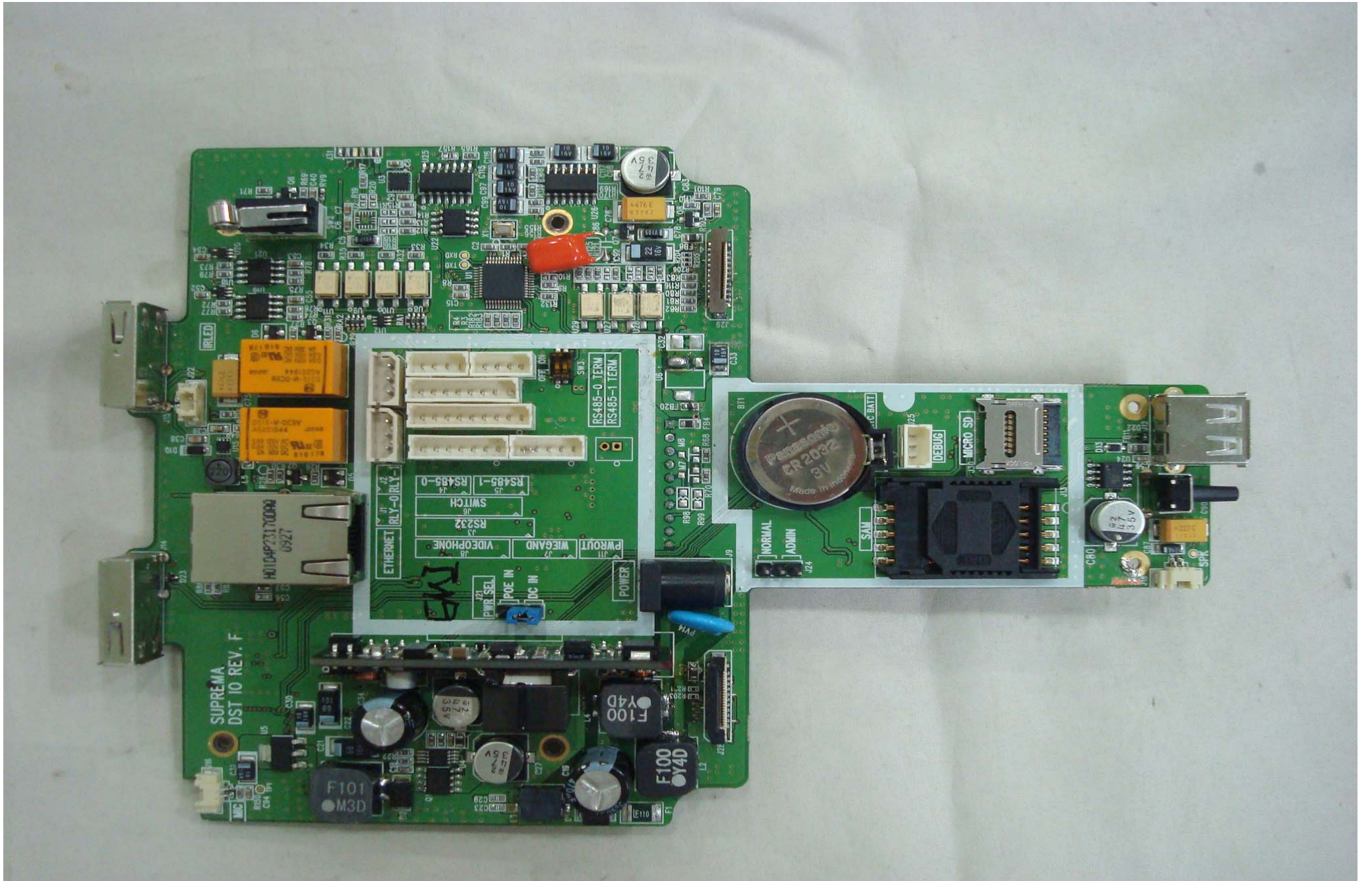
IO BOARD 전면
