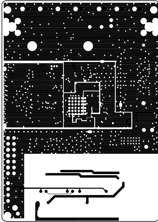
Layer 3 VCC
