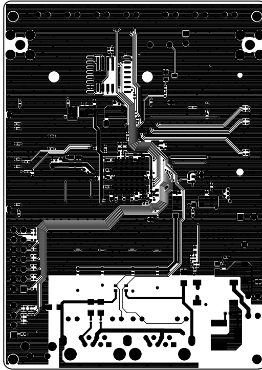
Layer 4 Bottom layer
