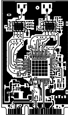
Layer 1 Top layer
