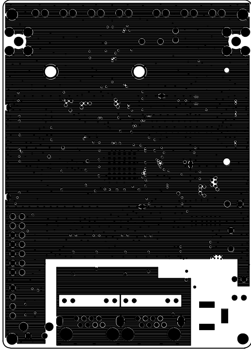
Layer 2 GND
