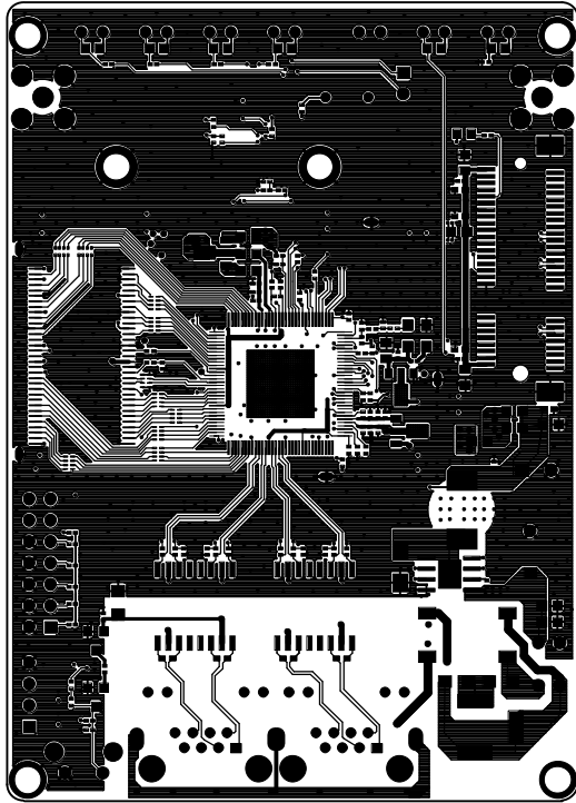
Layer 1 Top layer
