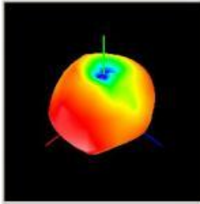
5.15GHz
