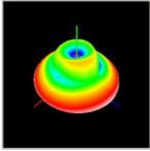
2.5GHz
