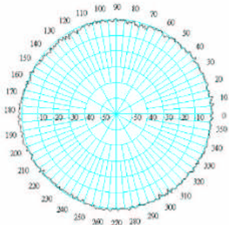
5.15-H-PLANE
