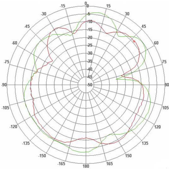
Elevation ZY
