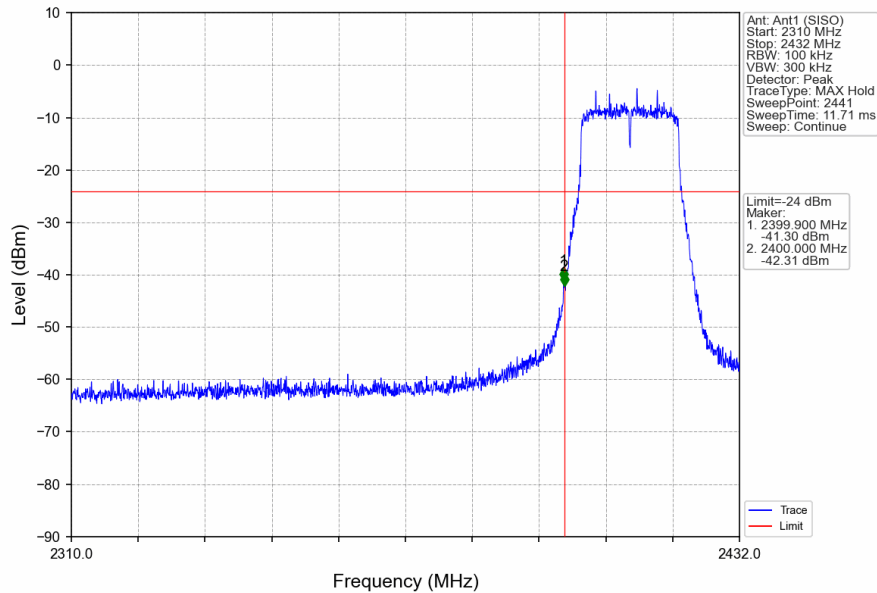
802.11n(HT20)_LCH_2412MHz_Ant1 (SISO)_NTNV
