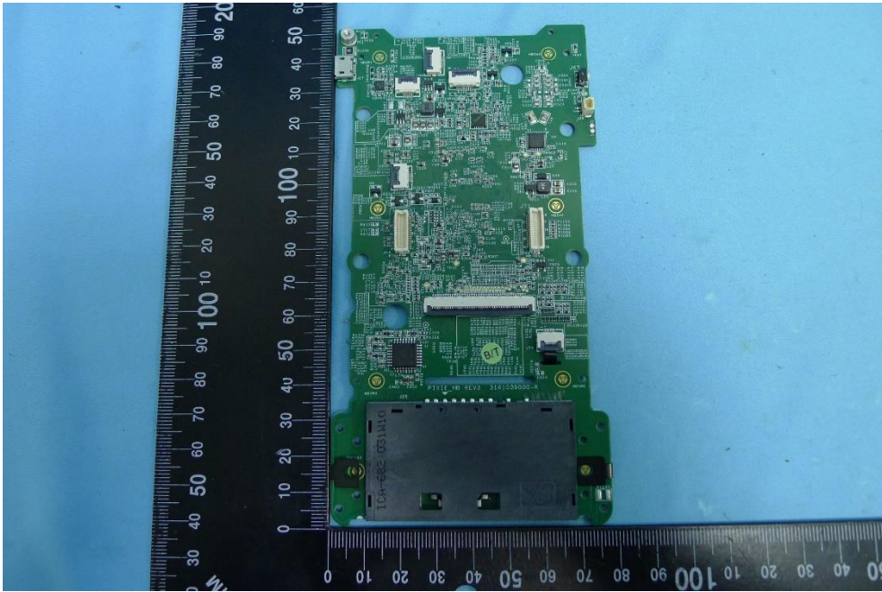
(15) EUT Photos
