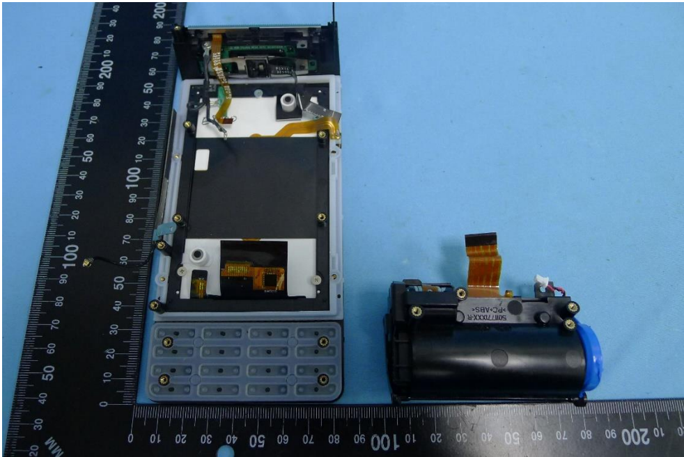
(19) EUT Photos
