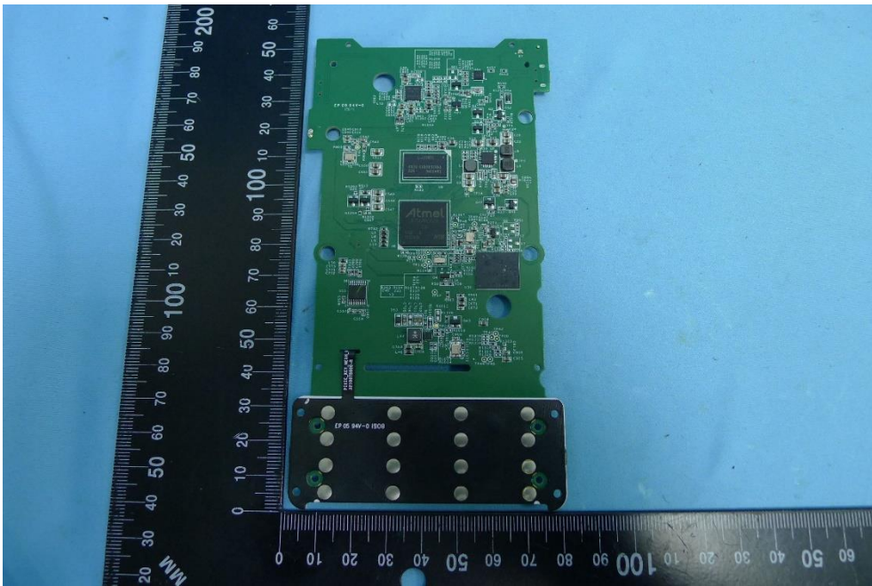
(16) EUT Photos
