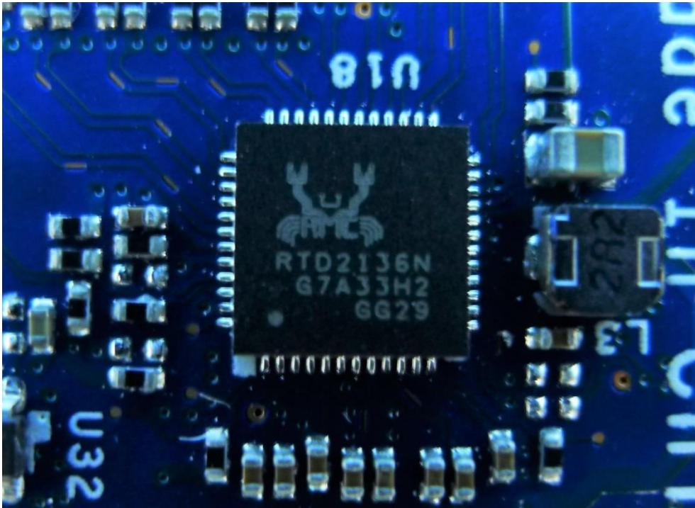
(19) EUT Photo
