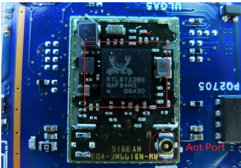
(18) EUT Photo
