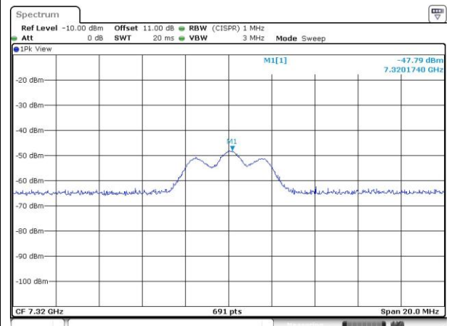
7320MHz - PK
