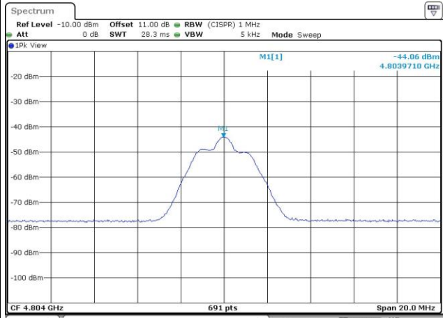
4804MHz - AV
