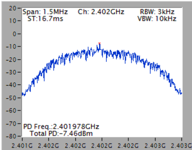
1Mbps
