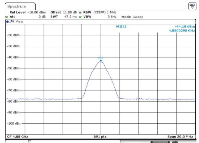
4880MHz - AV
