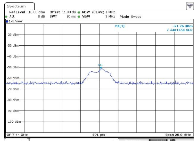
7440MHz - PK
