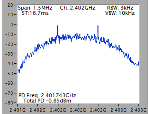
2Mbps
