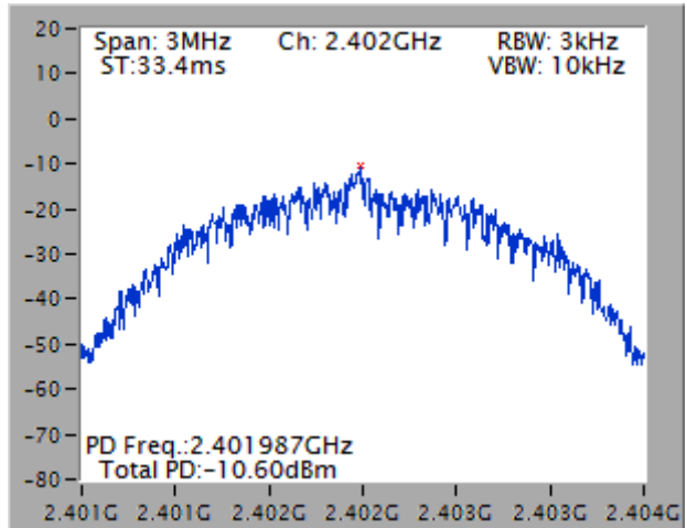
2Mbps
