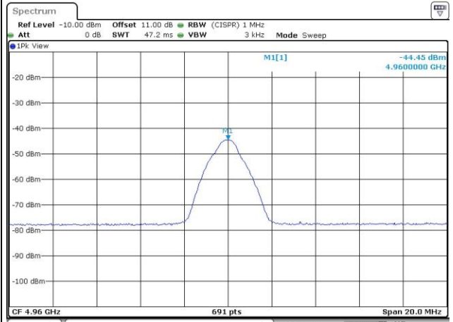
4960MHz - AV
