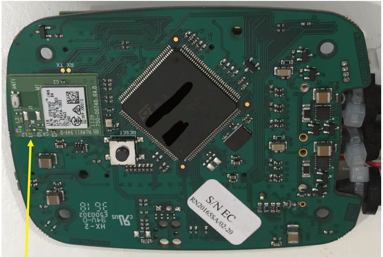
Laird 450-015 module
