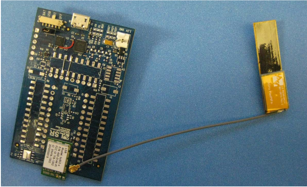
FlexPIFA Antenna
