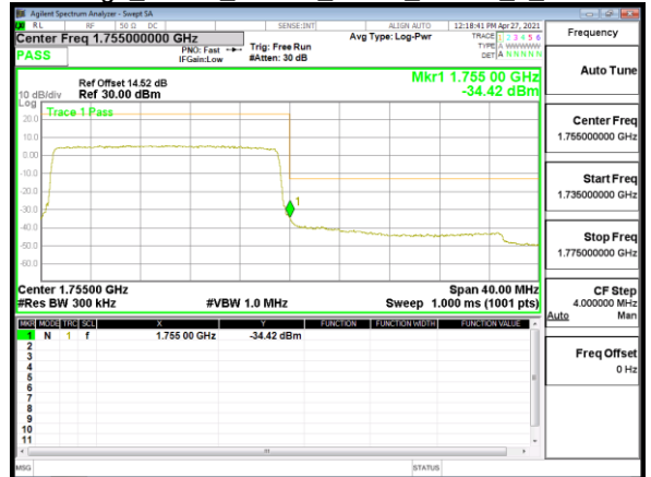
Band Edge_Band4_20MHz_QPSK_RB100_0_CH20300
