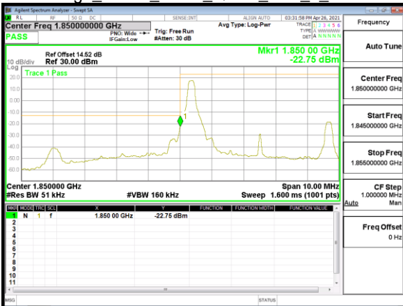
Band Edge_Band2_5MHz_QPSK_RB1_0_CH18625
