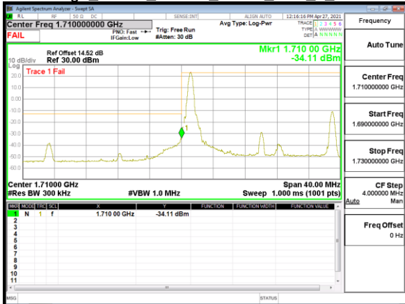
Band Edge_Band4_20MHz_QPSK_RB1_0_CH20050
