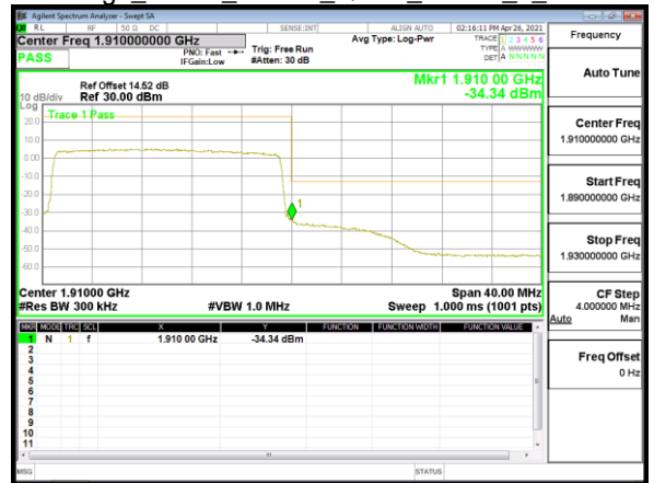
Band Edge_Band2_20MHz_QPSK_RB100_0_CH19100
