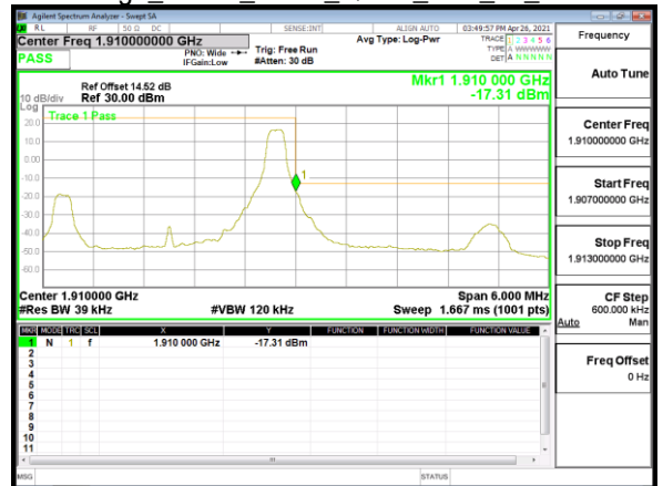
Band Edge_Band2_3MHz_QPSK_RB1_14_CH19185
