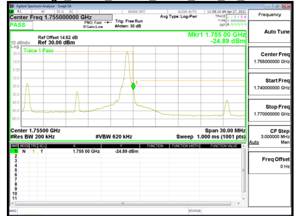
Band Edge_Band4_15MHz_QPSK_RB1_74_CH20325
