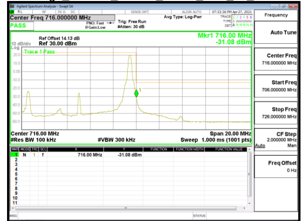
Band Edge_Band12_10MHz_QPSK_RB1_49_CH23130
