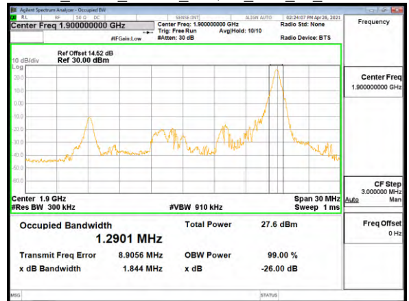
OBW_Band2_20MHz_16QAM_RB1_99_CH19100
