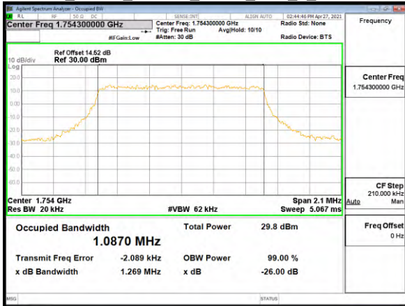
OBW_Band4_1.4MHz_QPSK_RB6_0_CH20393
