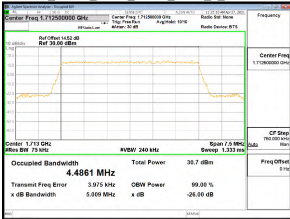
OBW_Band4_5MHz_QPSK_RB25_0_CH20175
