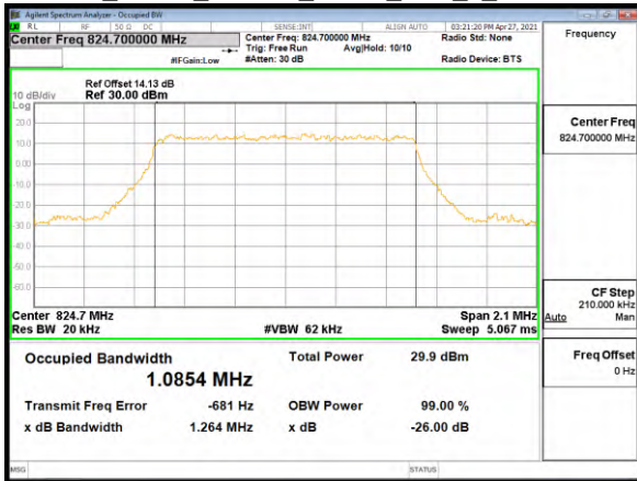
OBW_Band5_1.4MHz_QPSK_RB6_0_CH20525
