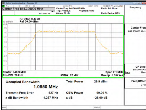
OBW_Band5_1.4MHz_QPSK_RB6_0_CH20643
