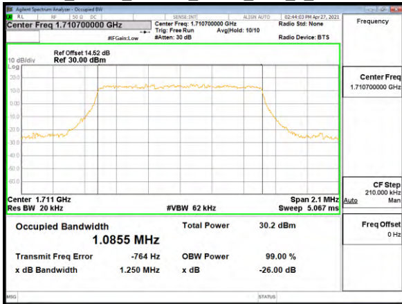
OBW_Band4_1.4MHz_QPSK_RB6_0_CH20175
