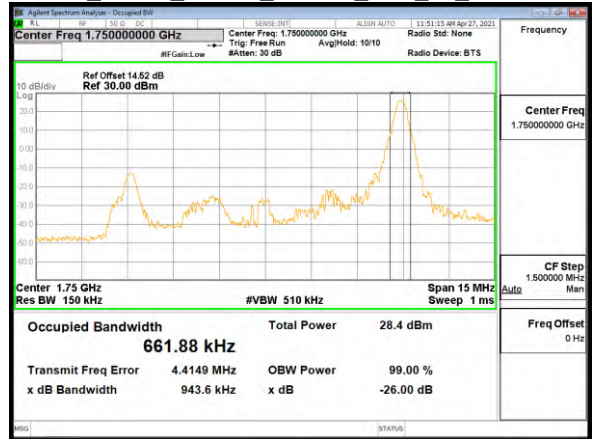
OBW_Band4_10MHz_16QAM_RB1_49_CH20350
