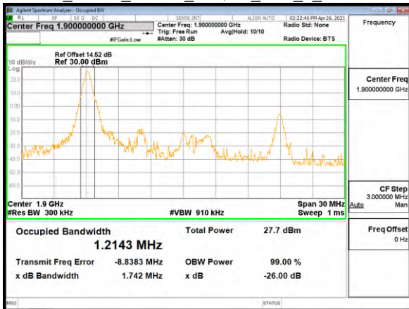
OBW_Band2_20MHz_16QAM_RB1_0_CH19100
