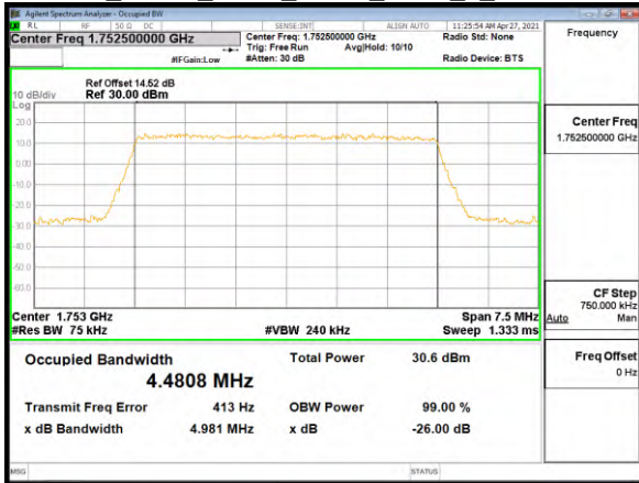
OBW_Band4_5MHz_QPSK_RB25_0_CH20375
