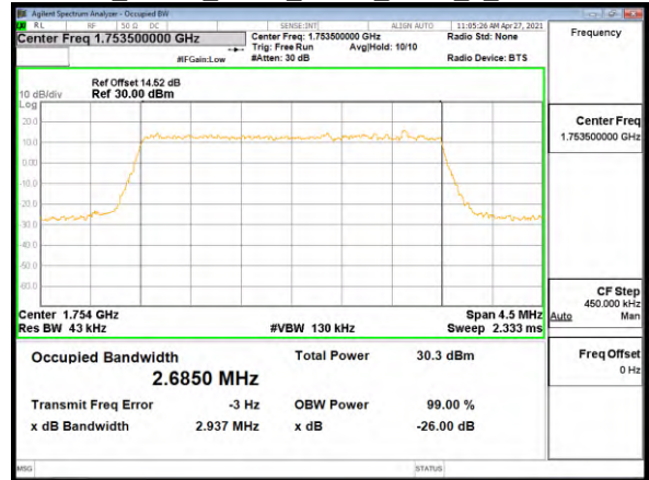
OBW_Band4_3MHz_QPSK_RB15_0_CH20385
