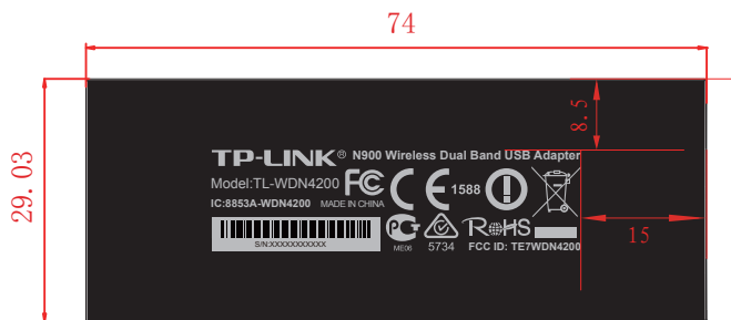
尺寸效果图
