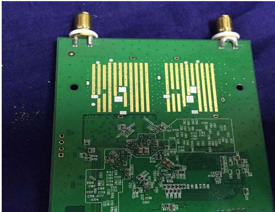
(6) EUT Photo
