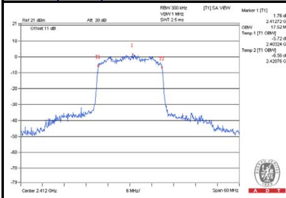
802.11n (20MHz)
