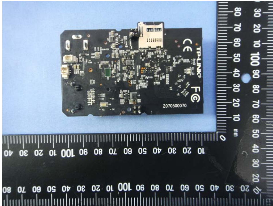
EUT Photo 10 )
