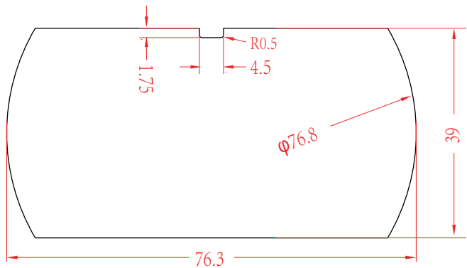
结构尺寸图
