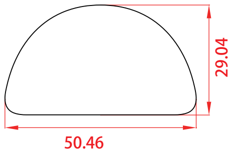
尺寸图
