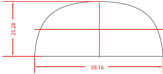
结构尺寸图
