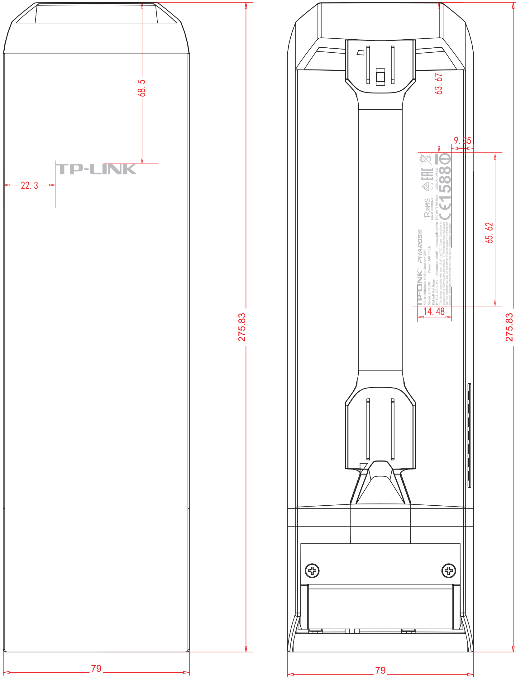
尺寸图
