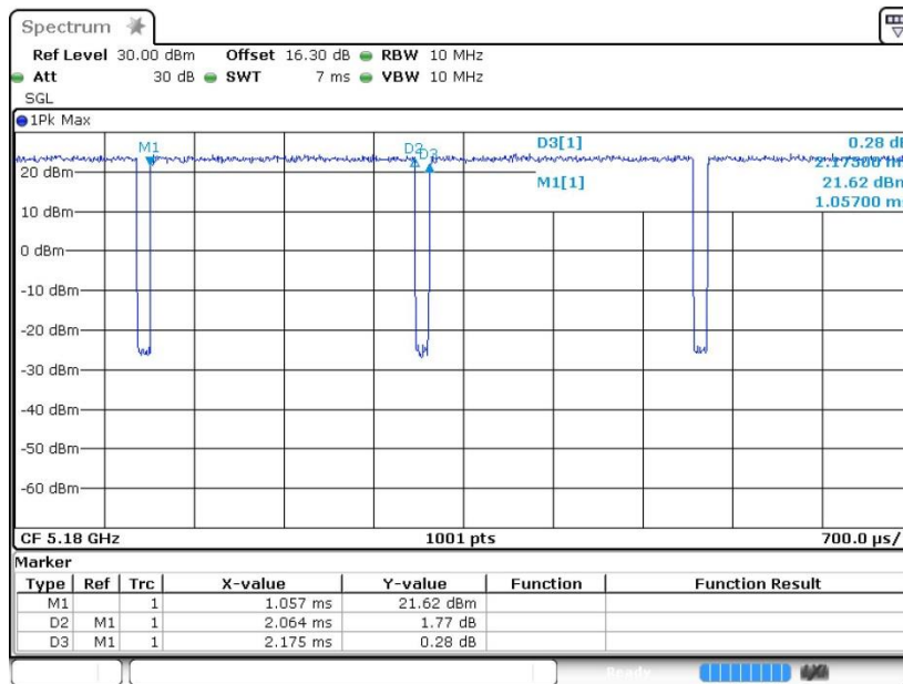
802.11a Antenna 1+2+3
