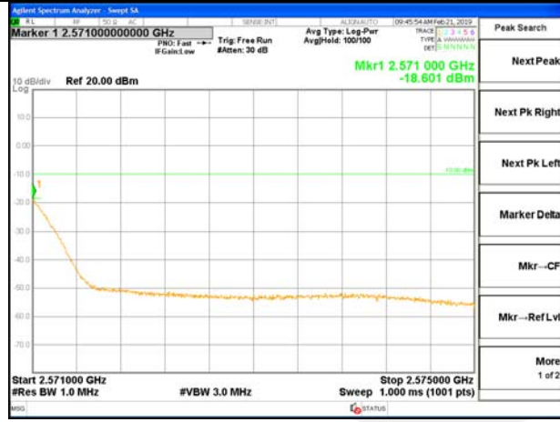
2571-2575MHz
