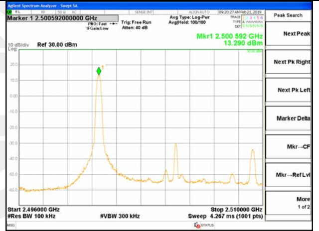
2496-2510MHz
