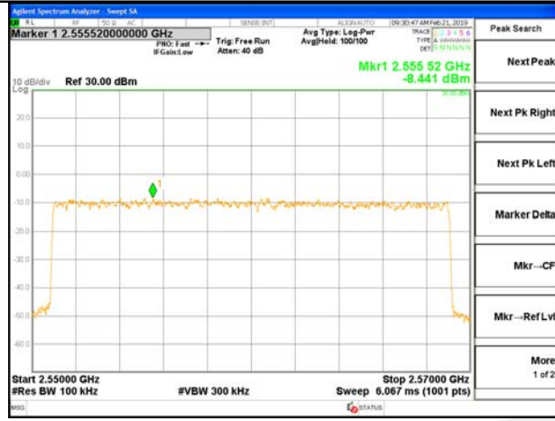
2550-2570MHz
