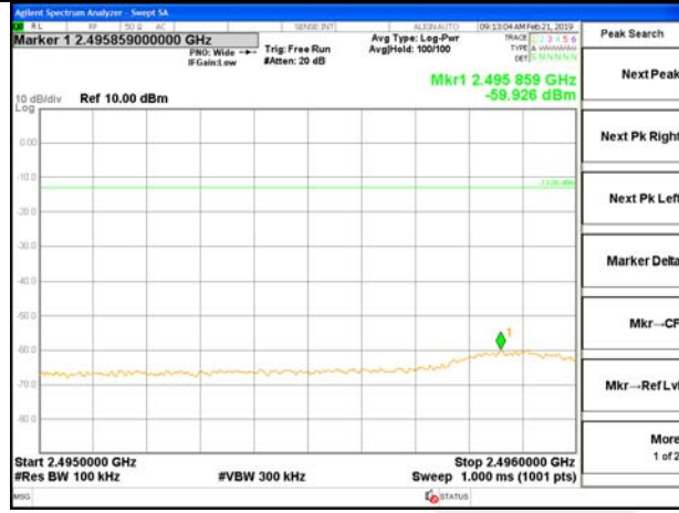
2495-2496MHz
