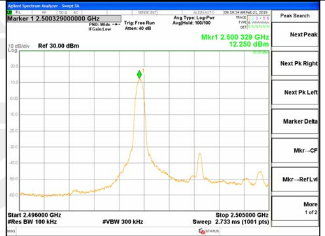
2496-2505MHz
