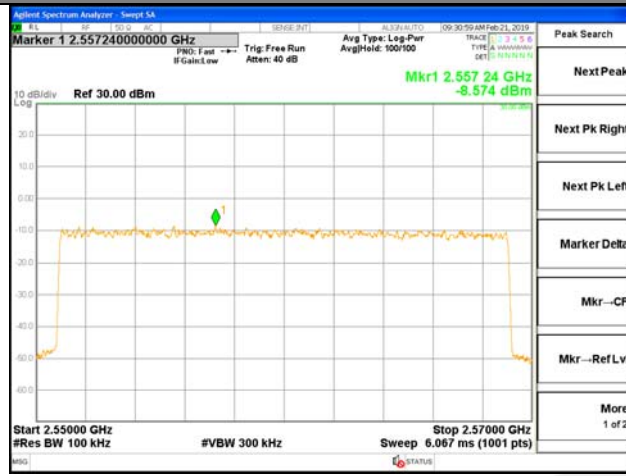
2550-2570MHz
