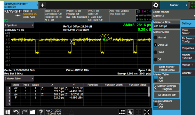
802.11ax-HE40 (T=771.2us)
