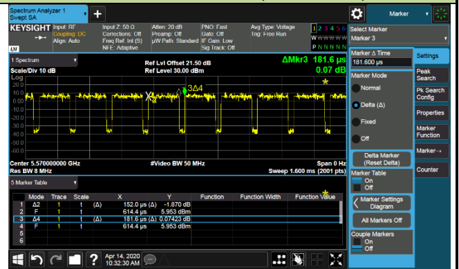
802.11ax-HE40 (T=421.7us)
