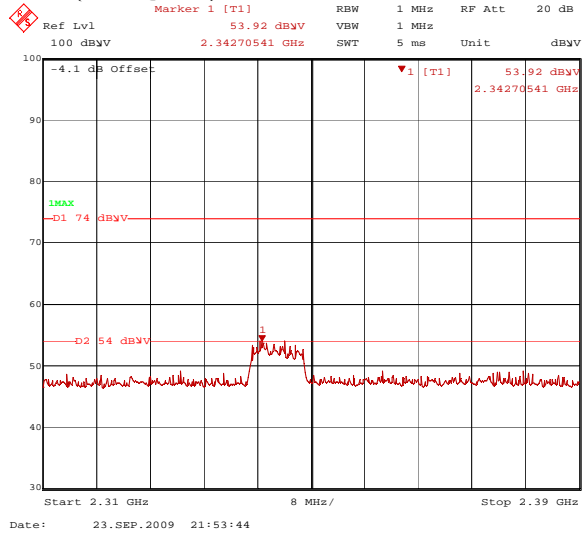
EDR (8DPSK)
