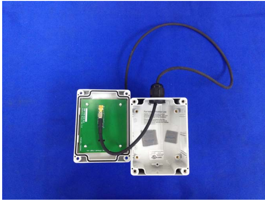
(5) EUT Photo (Antenna 1a)
