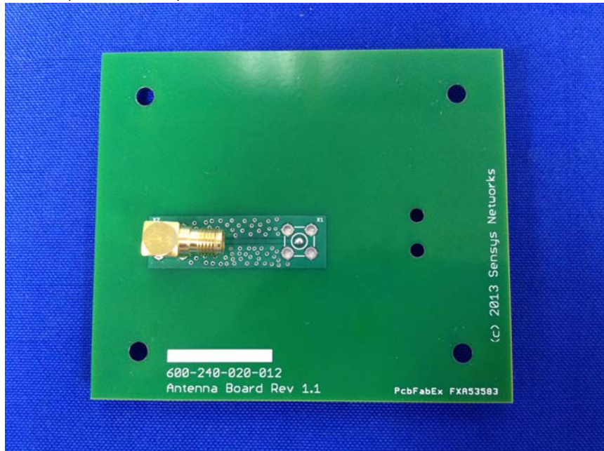
(6) EUT Photo (Antenna 1a)
