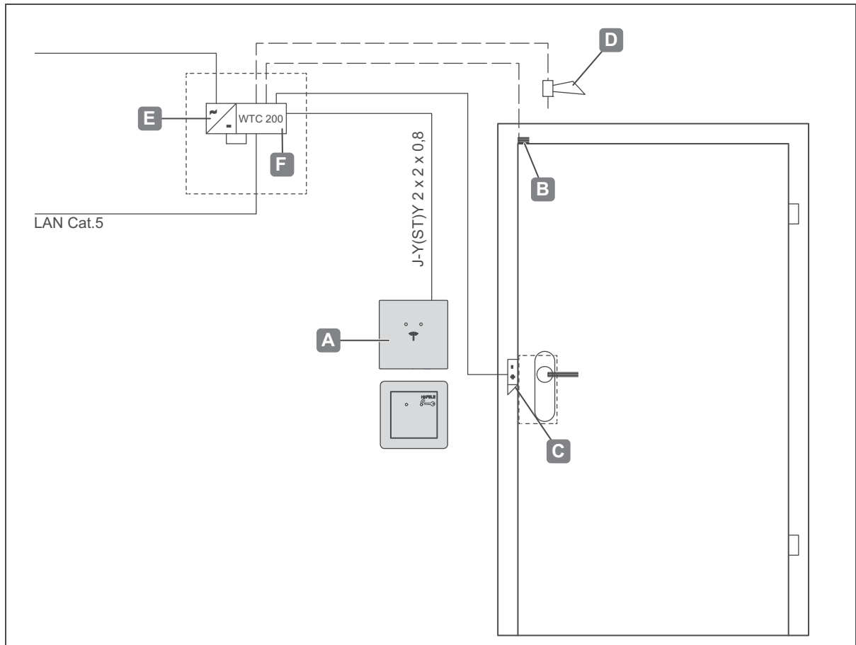
Fig. 23: Exemplo de instalação 1 – porta com um leitor, contacto de sinalização de porta, testa elétrica, gerador de sinal e controlador
