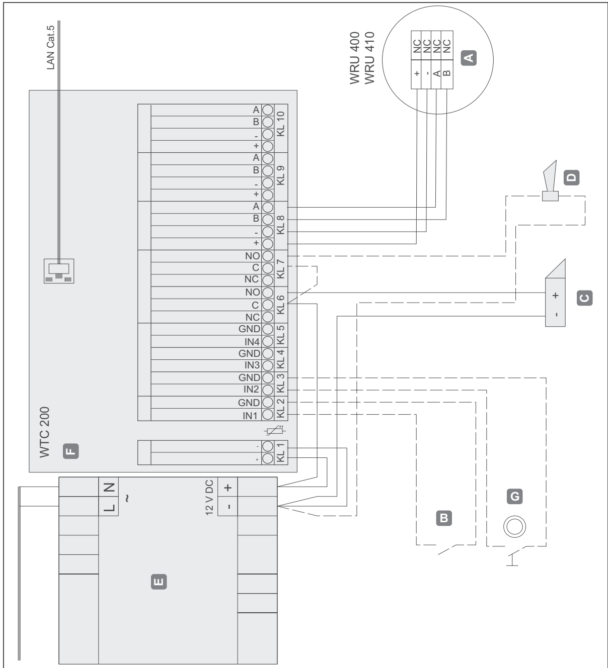
Fig. 26: Schema elettrico per esempio di installazione 2
