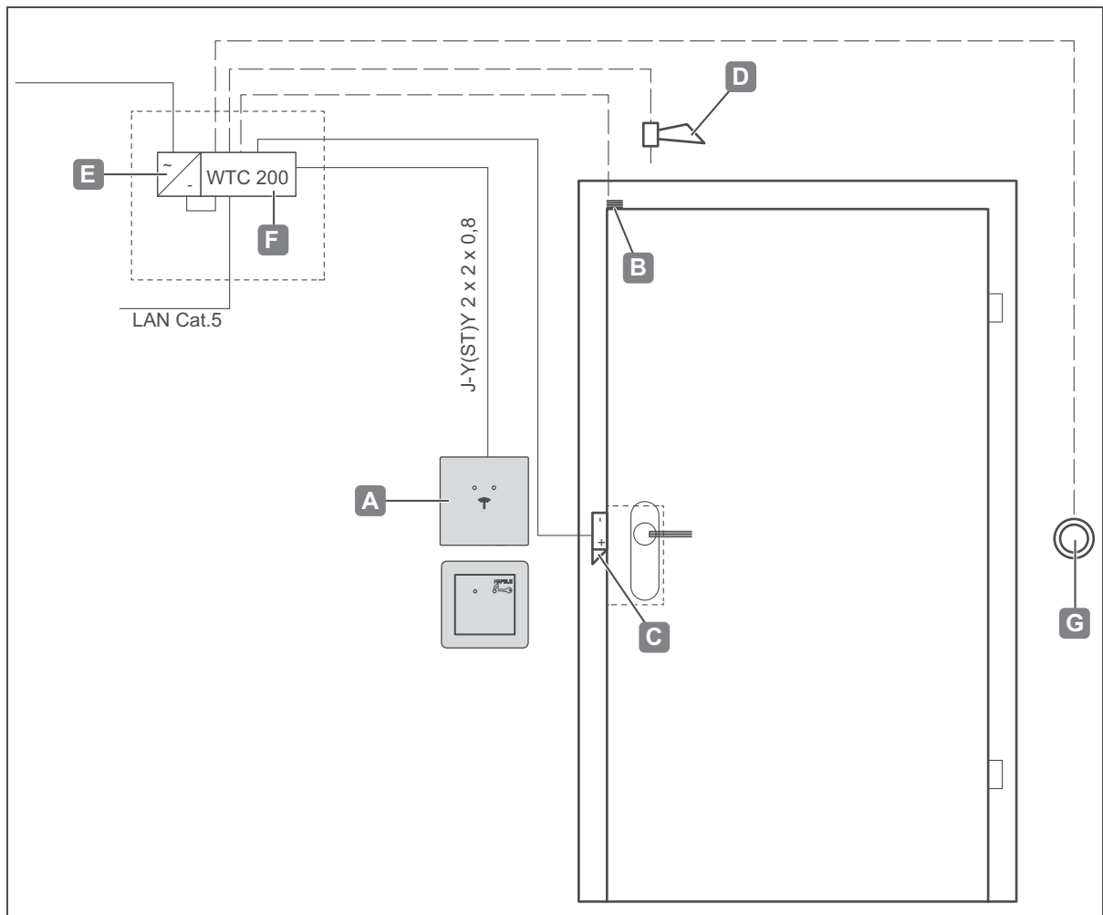
Fig. 25: Exemplo de montagem 2 – porta com um leitor, contacto de sinalização de porta, testa elétrica, gerador de sinal, botão de desbloqueio da porta e controlador
