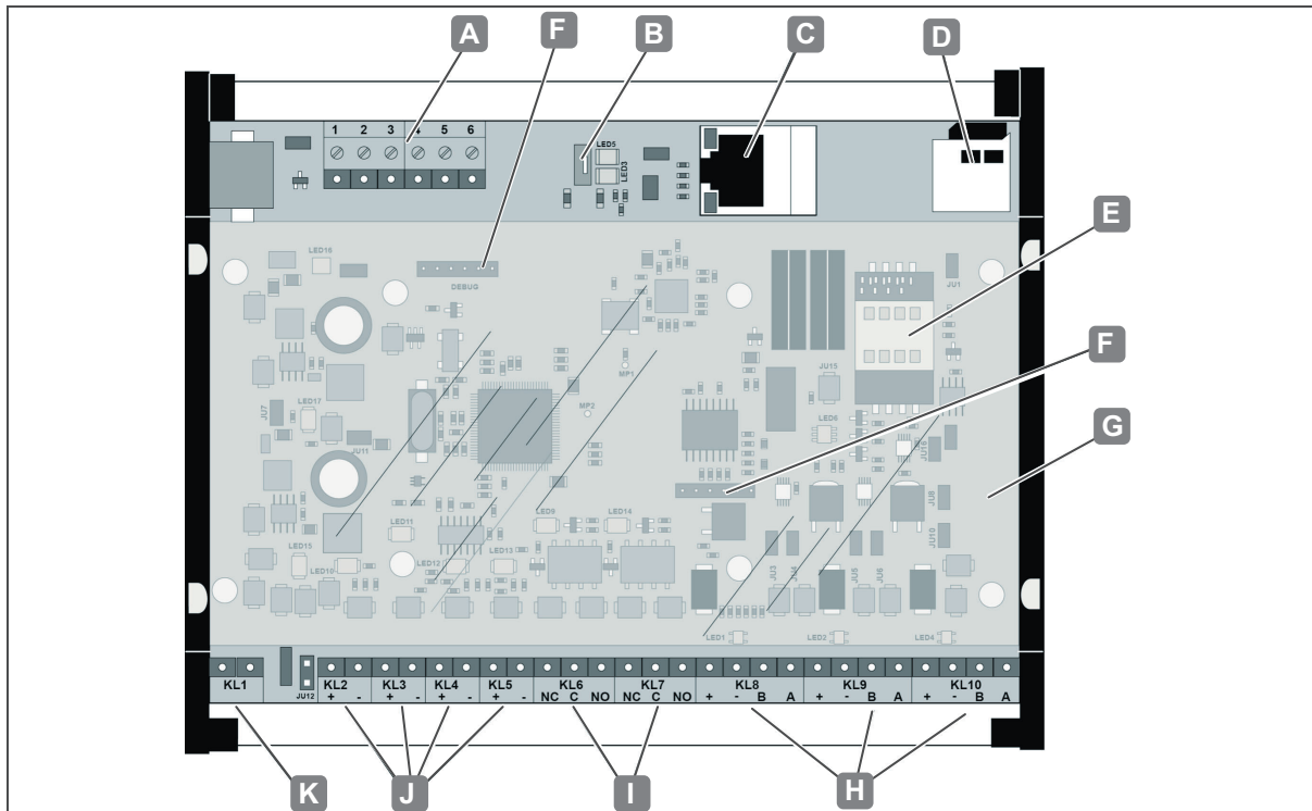
Ilustr. 14: Conexiones WTC 200
