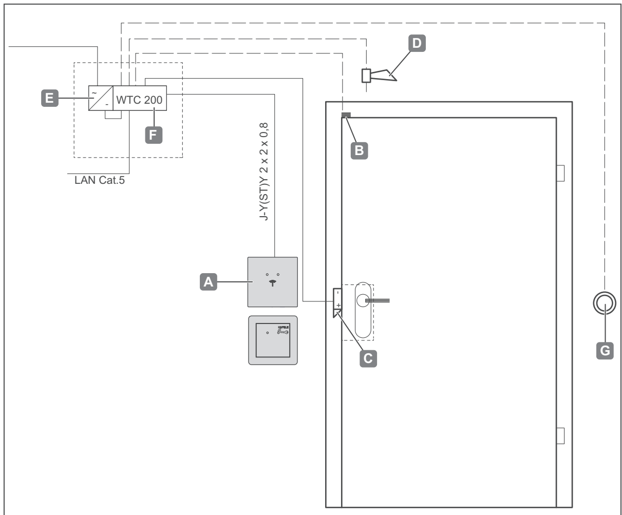
Fig. 25: Exemple d'installation 2 - Une porte avec un lecteur, un contact d'état de porte, une gâche électrique, un générateur de signal sonore, un bouton-poussoir d'ouverture de porte et un contrôleur
