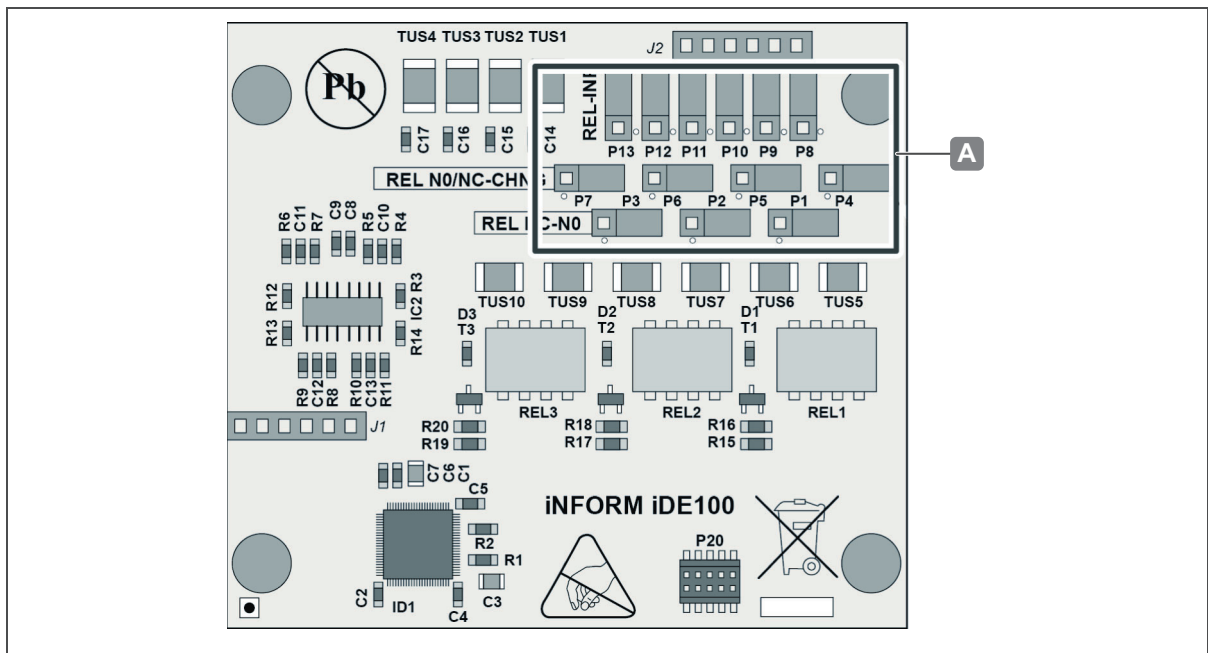
Ilustr. 18: I/O WTX 200 - Posición de los puentes en la aplicación para otras entradas analógicas/digitales
