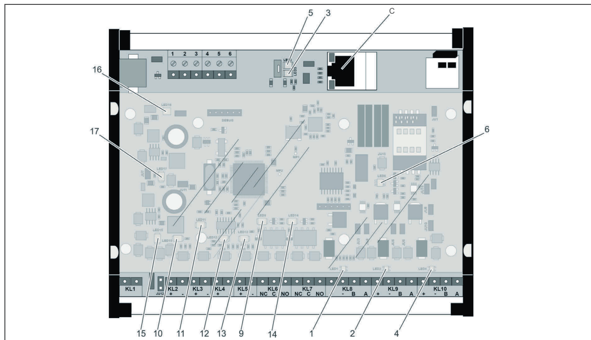
Ilustr. 12: Vista general de LEDs en el controlador WTC 200
