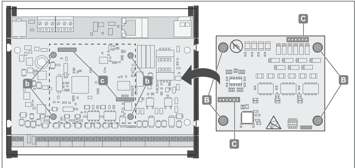
Ilustr. 9: Montaje I/O WTX 200 - I/O WTX 200 insertar en el controlador WTC 200
