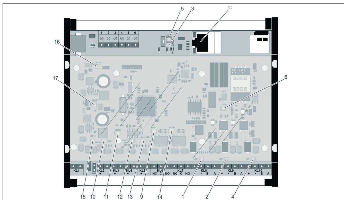
Fig. 12: Panoramica LED sul controller WTC 200
