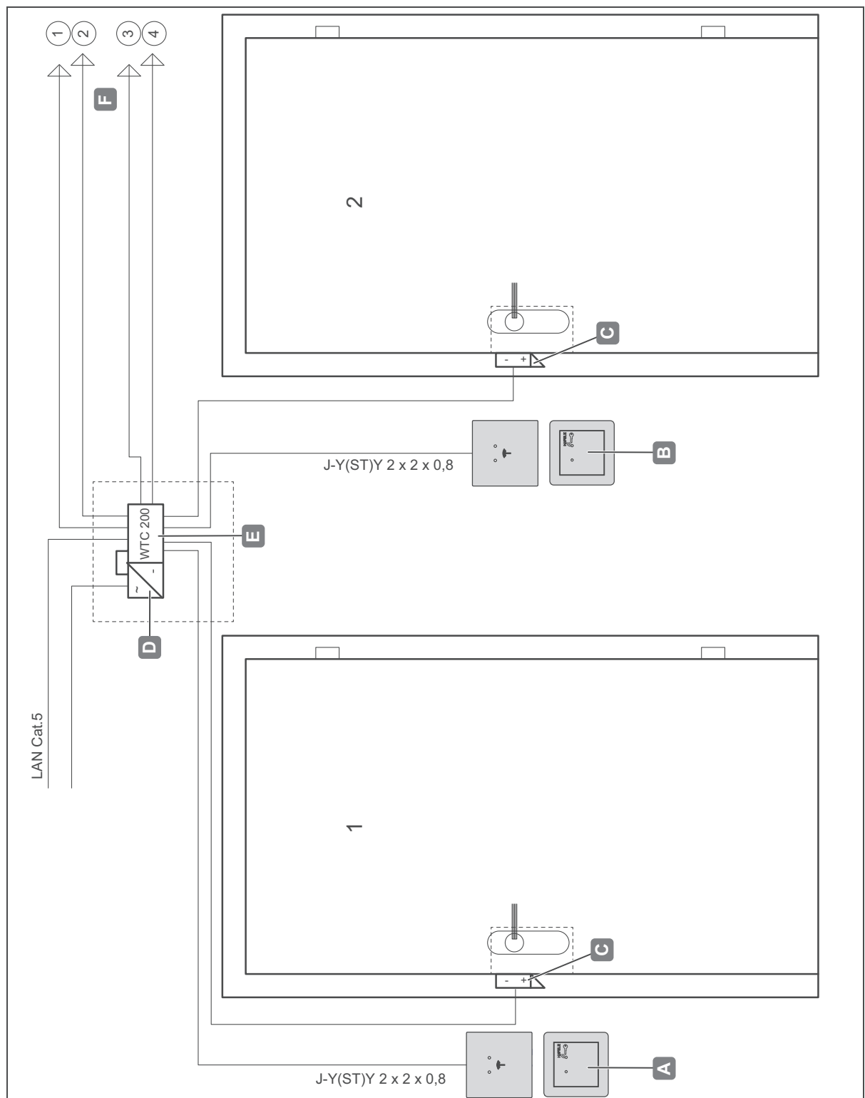
Fig. 31: Exemplo de instalação 5 – parte 1 – quatro portas com um leitor/testa elétrica e um controlador cada (incluindo módulo adicional)
