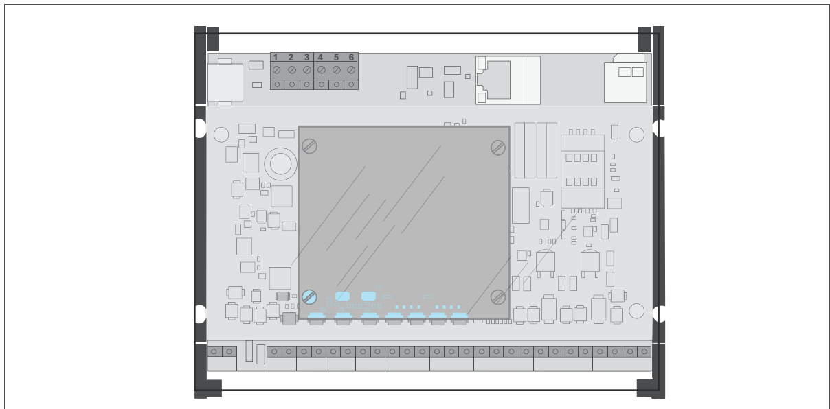
Fig. 3: I/O WTX 200 - fissato sul controller
