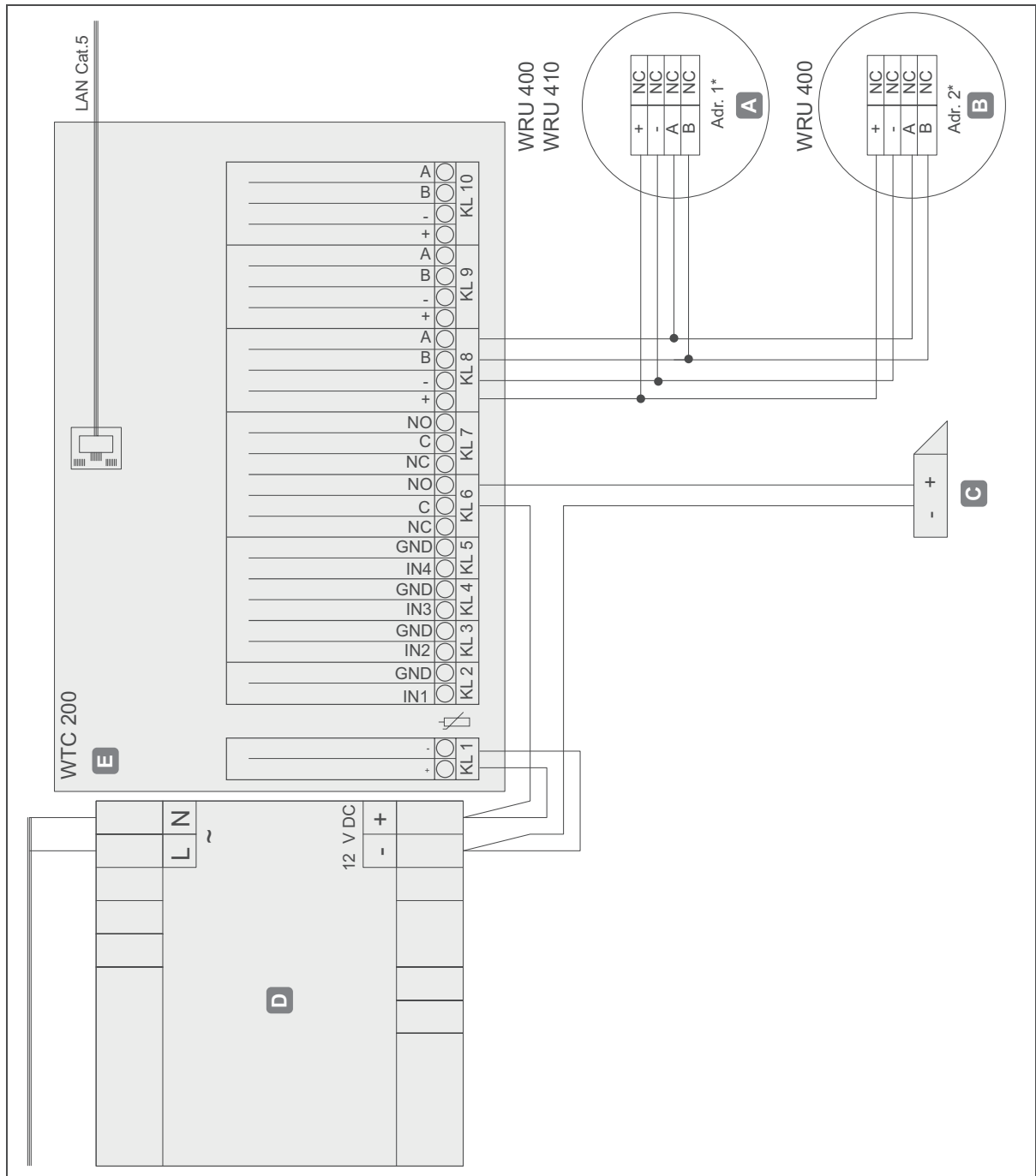
Fig. 28: Schéma de connexion pour l'exemple d'installation 3
