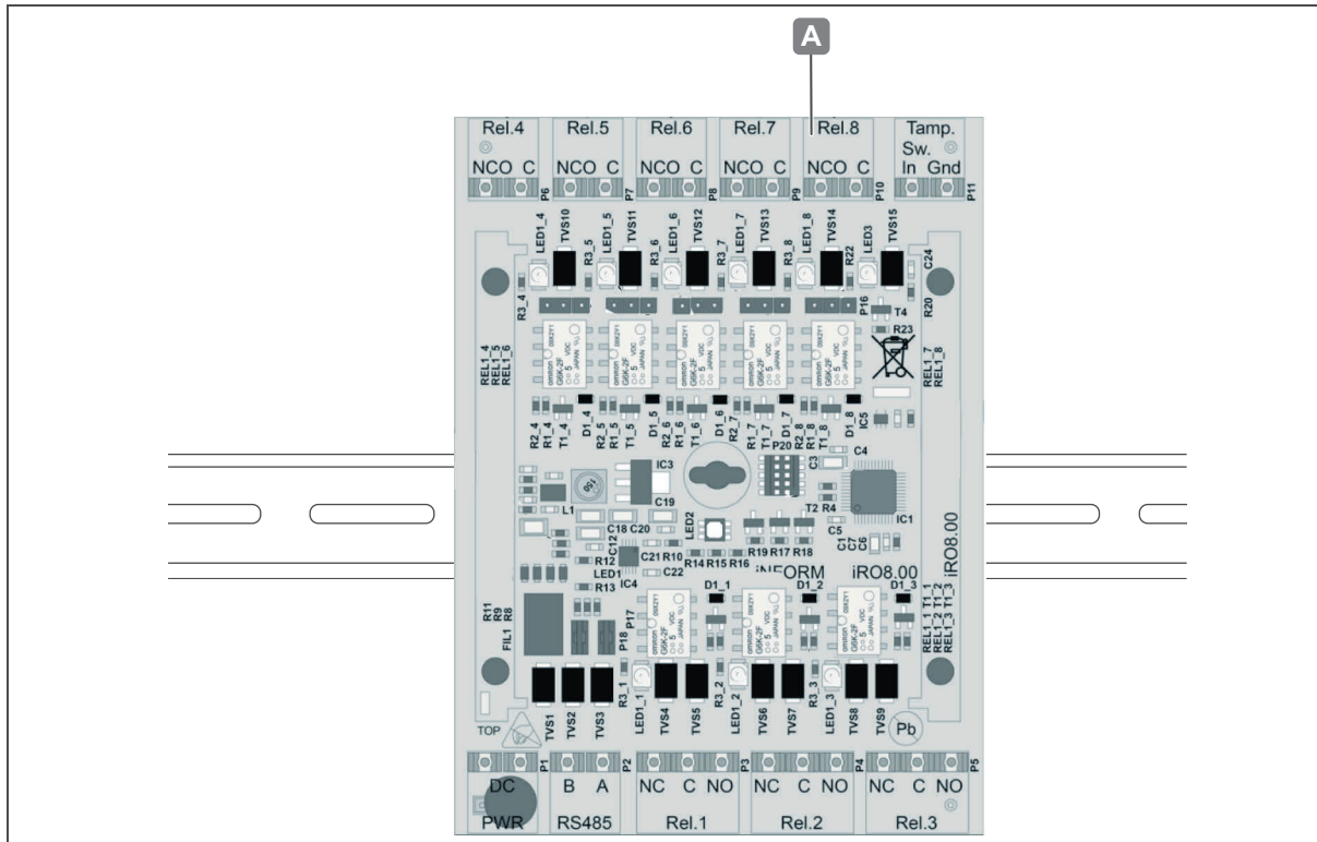
Ilustr. 11: Montaje WTX 201 en el carril de perfil
