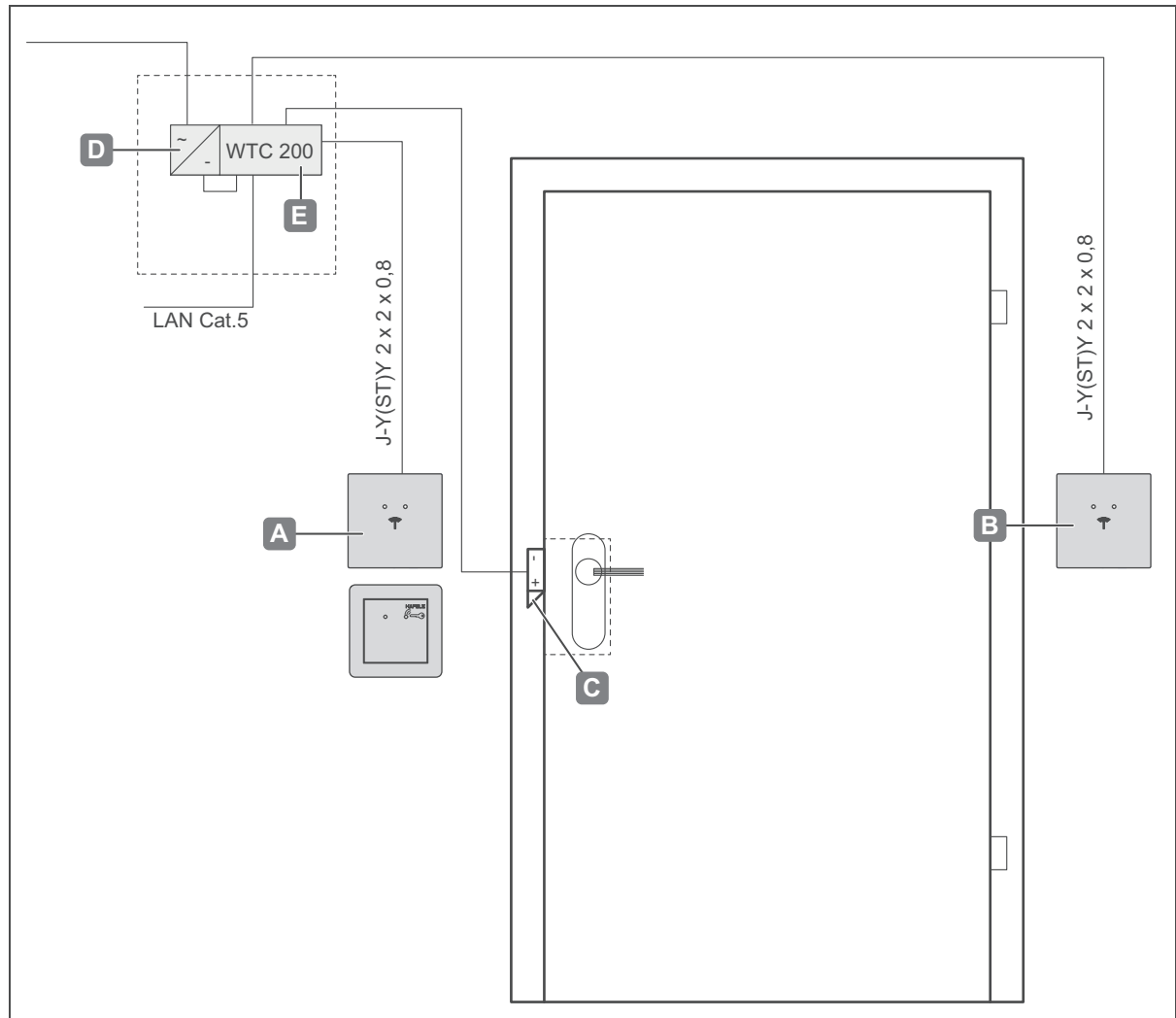
Fig. 27: Esempio di installazione 3 - Una porta con due lettori (ad es. interno ed esterno), apriporta e controller
