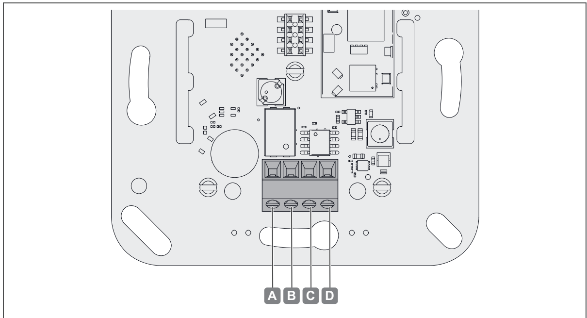
Fig. 13: Connessioni WRU 400 / WRU 410
