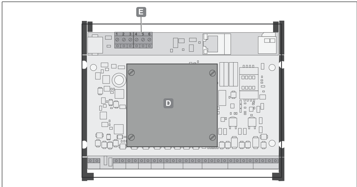
Abb. 10: Montage I/O WTX 200 - auf Controller aufgesteckt
