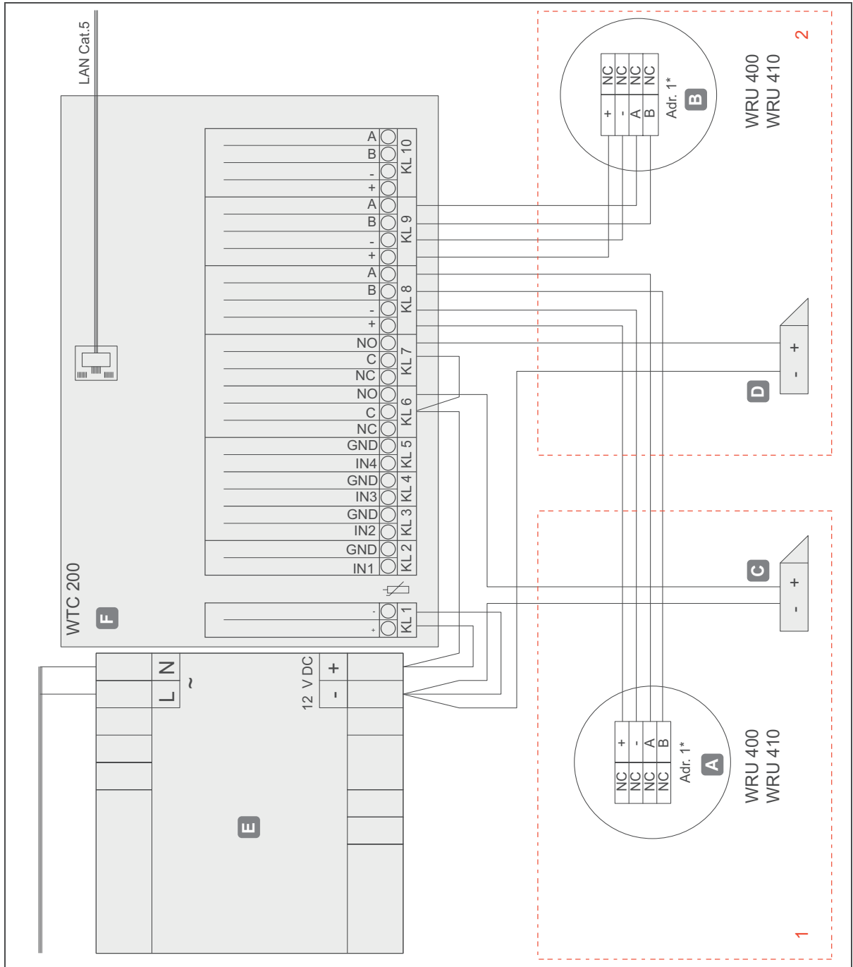
Ilustr. 30: Esquema de conexión para el ejemplo de instalación 4
