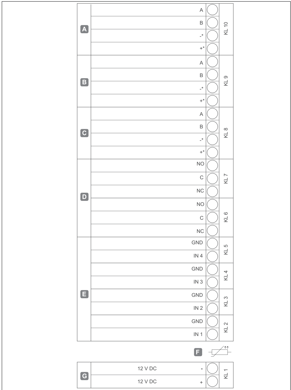
Ilustr. 21: Asignación de bornes controlador WTC 200
