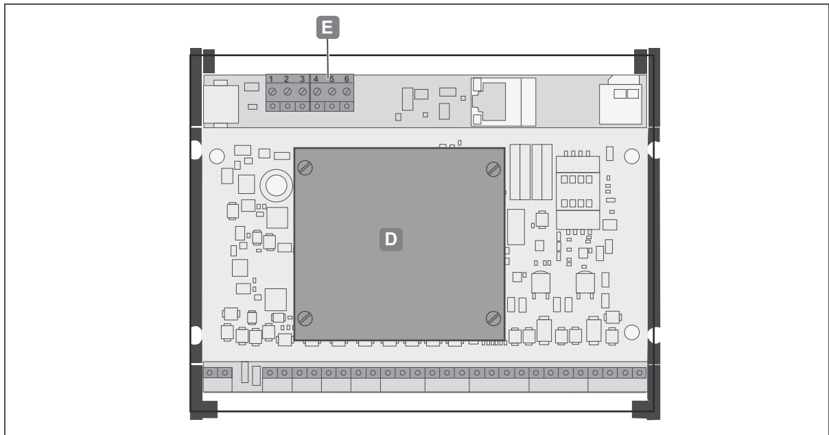
Fig. 10: Montage I/O WTX 200 - enfiché sur le contrôleur
