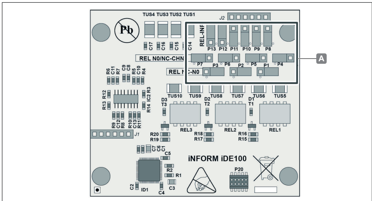
Abb. 19: I/O WTX 200 – Position der Jumper bei Verwendung für 2 weitere Relaisausgänge und 1 weiteren Analog-/Digitaleingang
