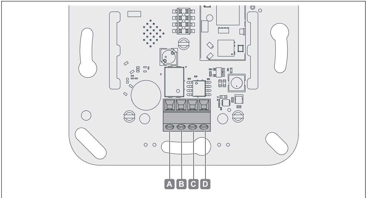
Fig. 13: Connexions WRU400 / WRU410
