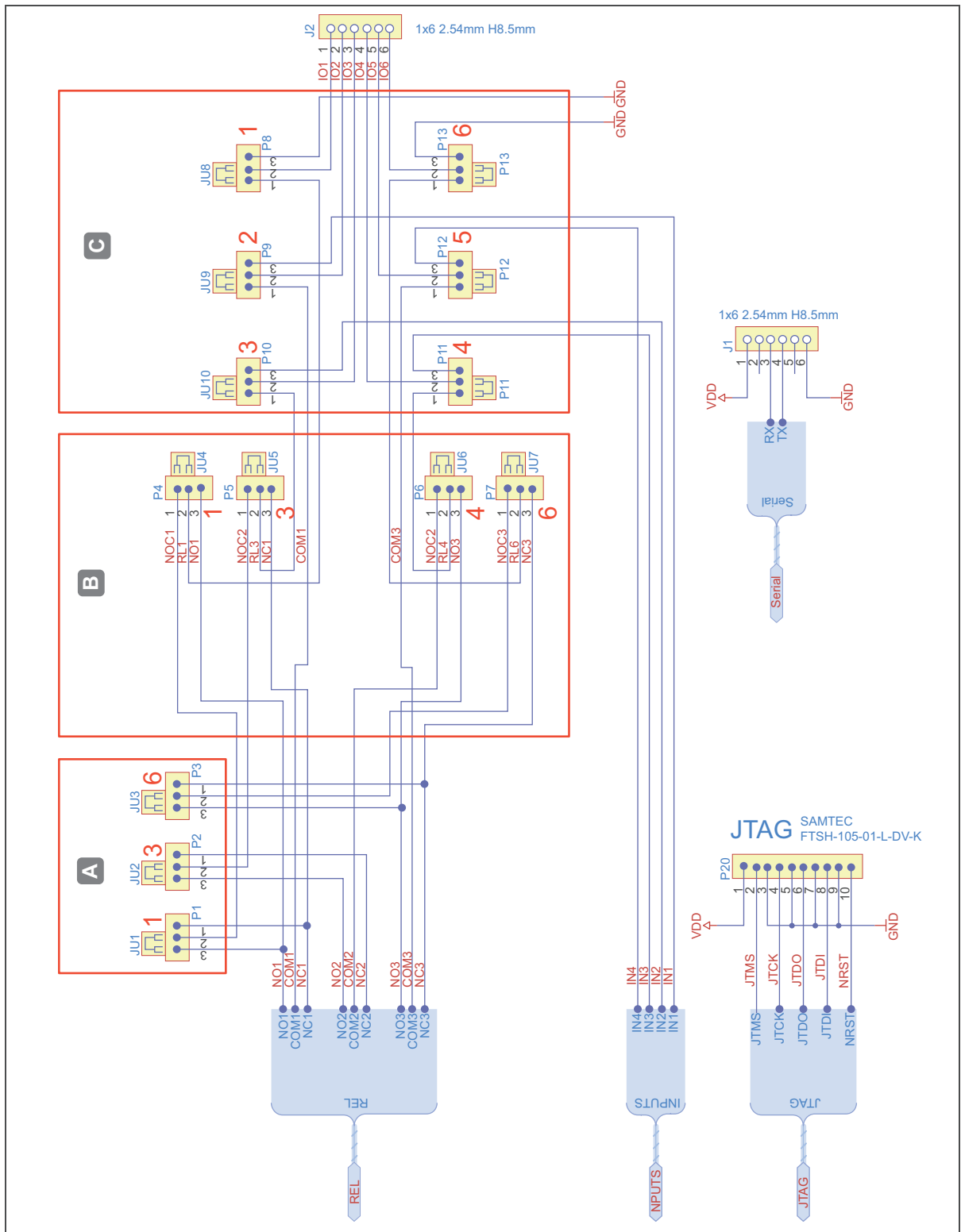
Abb. 16: Aufbau und Pin-Belegung des I/O WTX 200
