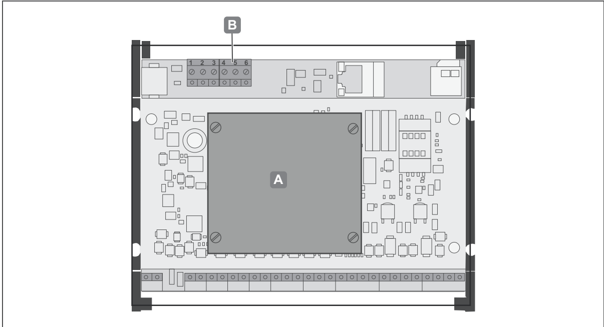
Ilustr. 15: Conexiones I/O WTX 200
