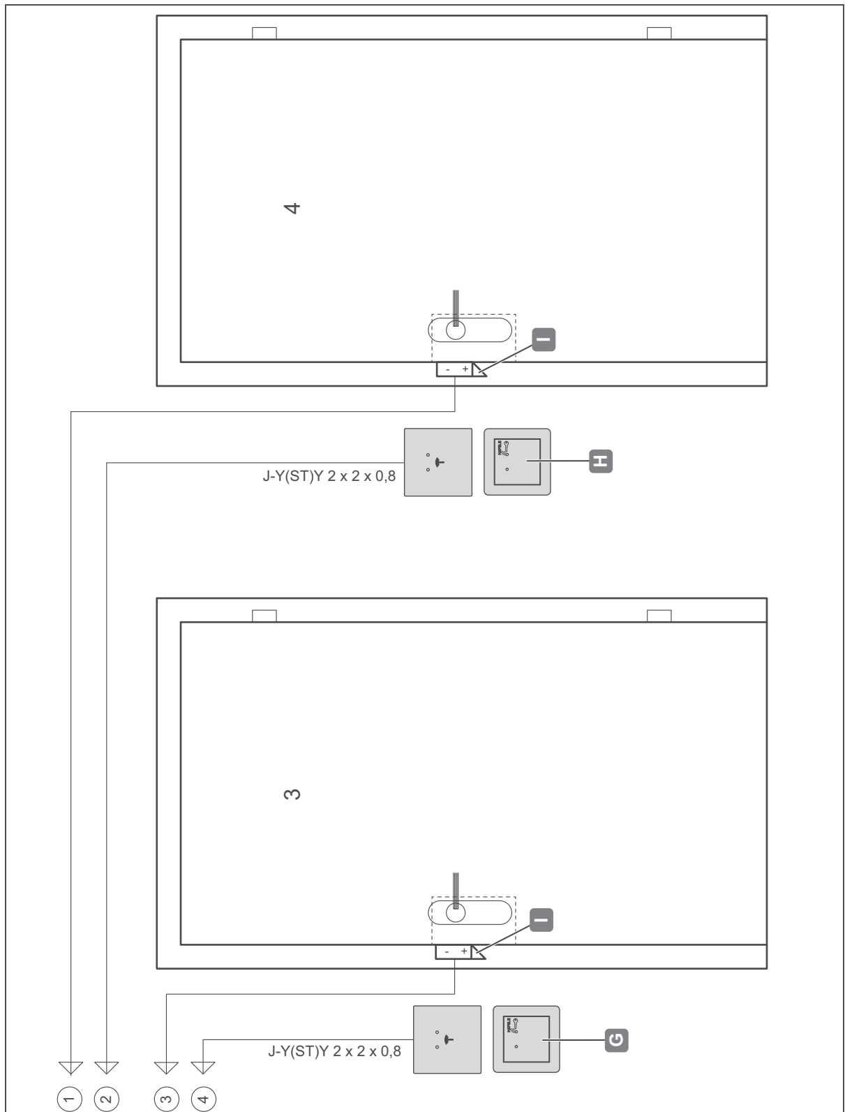
Ilustr. 32: Ejemplo de instalación 5 - parte 2 - Cuatro puertas con un lector cada una / abrepuertas y un controlador (incl. módulo adicional)
