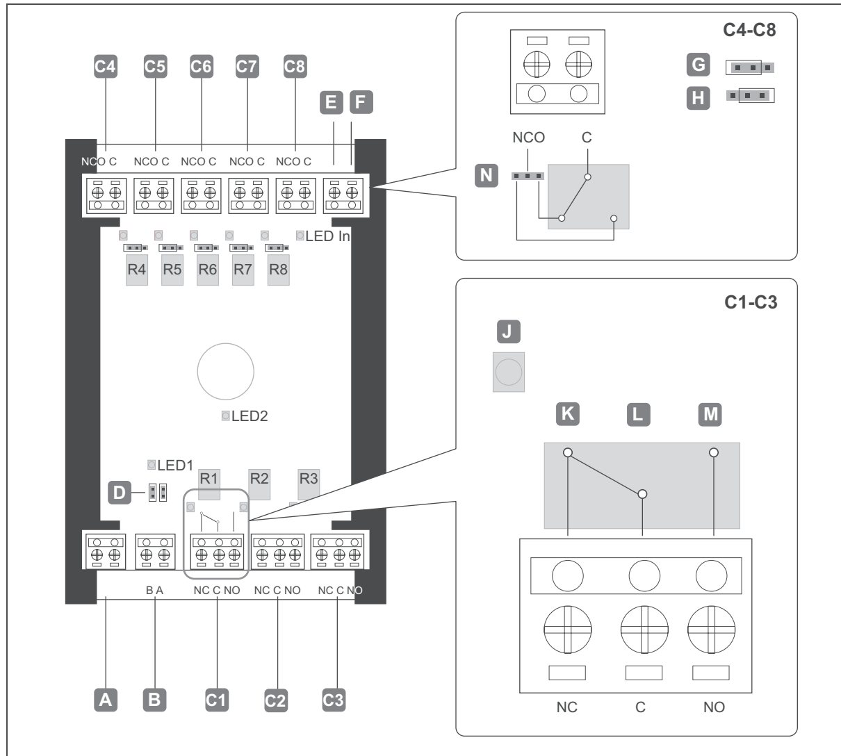
Fig. 22: Diagrama de ligação para o módulo de relé de 8 saídas WTX 201
