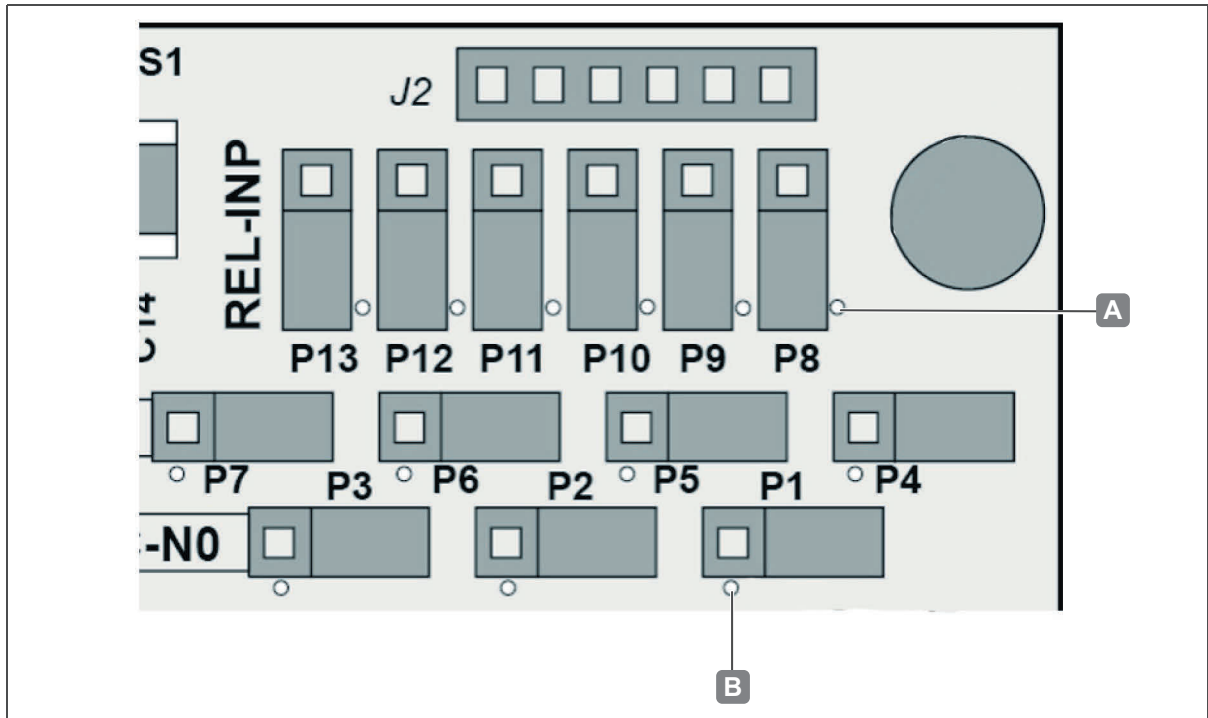
Abb. 17: Anschlüsse I/O WTX 200- Position Anschluss Nr. 1 (weißer Punkt)
