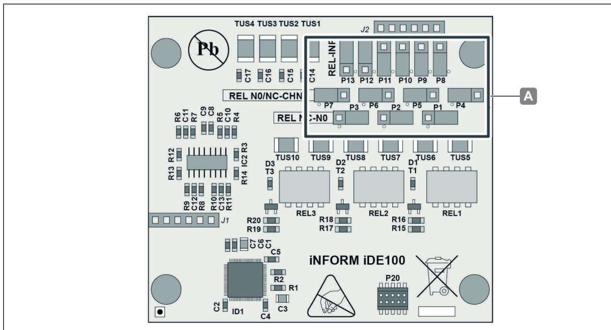
Fig. 19: I/O WTX 200 - Posizione dei ponticelli in caso di utilizzo per altre 2 uscite relè e 1 altri ingressi analogici/digitali
