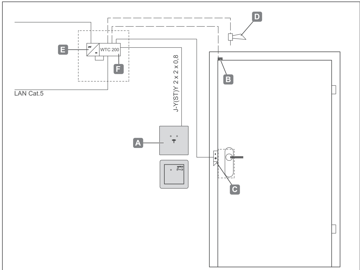
Abb. 23: Installationsbeispiel 1 - Eine Tür mit einem Leser, Türmeldekontakt, Türöffner, Signalgeber und Controller
