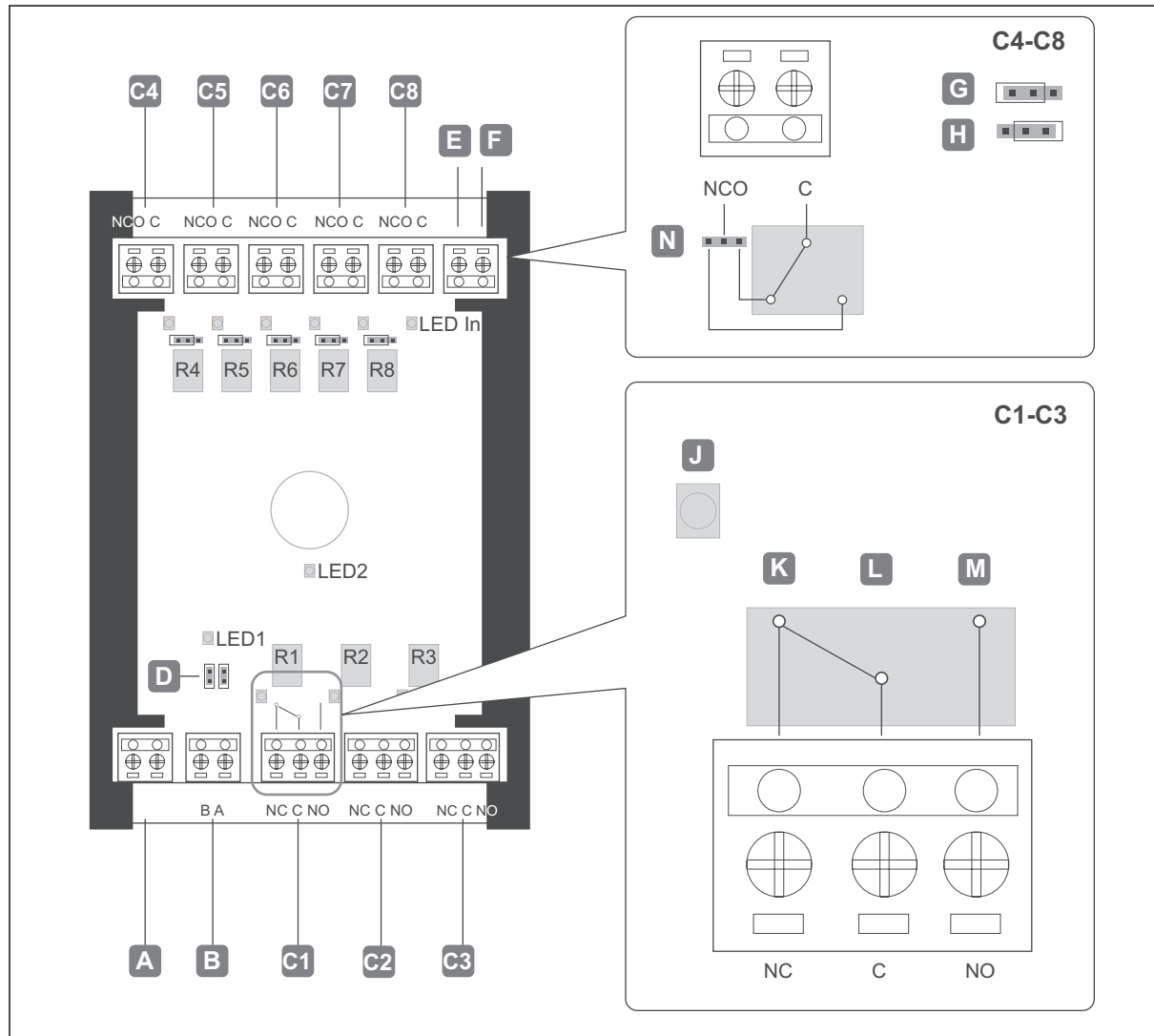
Abb. 22: Anschlussplan 8-fach-Relaismodul WTX 201
