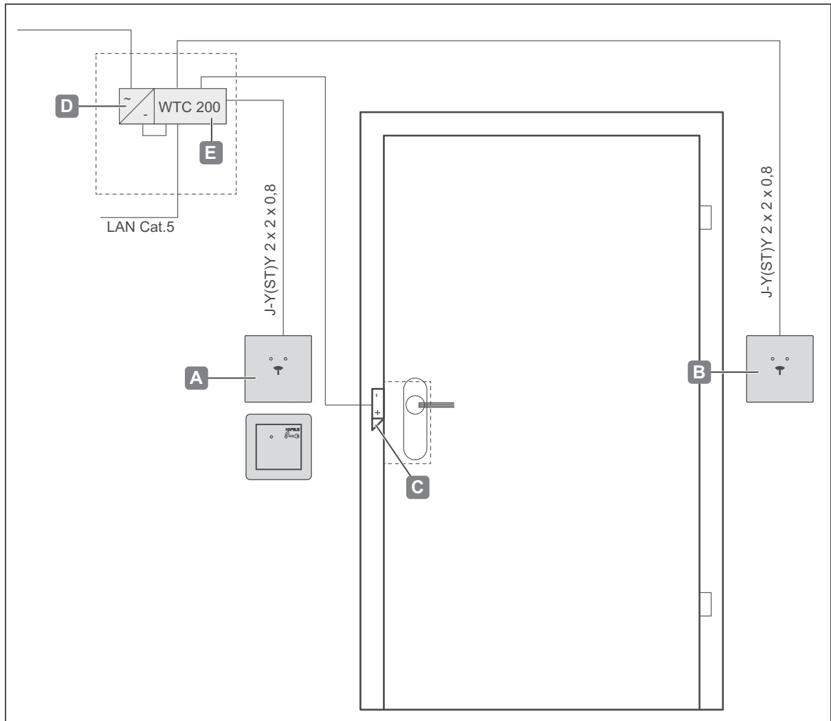
Ilustr. 27: Ejemplo de instalación 3 - Una puerta con dos lectores (p. ej. interior y exterior), abrepuertas y controlador
