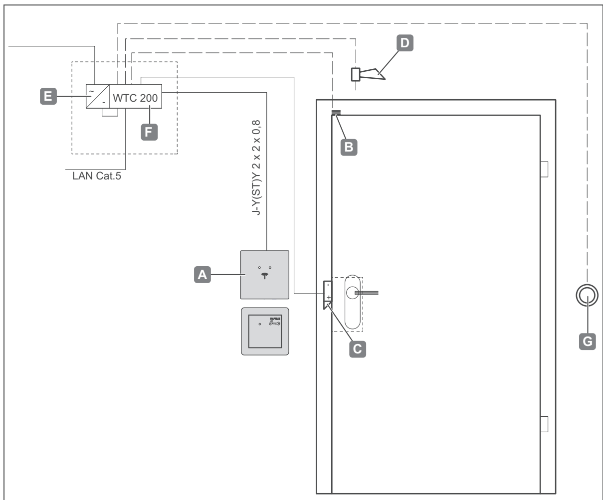
Ilustr. 25: Ejemplo de instalación 2 - Una puerta con un lector, contacto auxiliar de estado de puerta, abrepuertas, emisor de señal, pulsador para abridor de puerta y controlador
