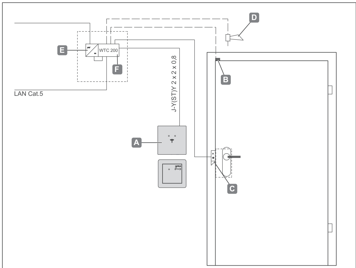
Fig. 23: Exemple d'installation 1 - Une porte avec un lecteur, un contact d'état de porte, une gâche électrique, un générateur de signal sonore et un contrôleur
