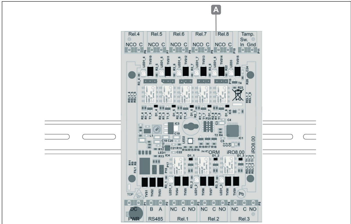
Fig. 11: Montage de WTX 201 sur le rail oméga
