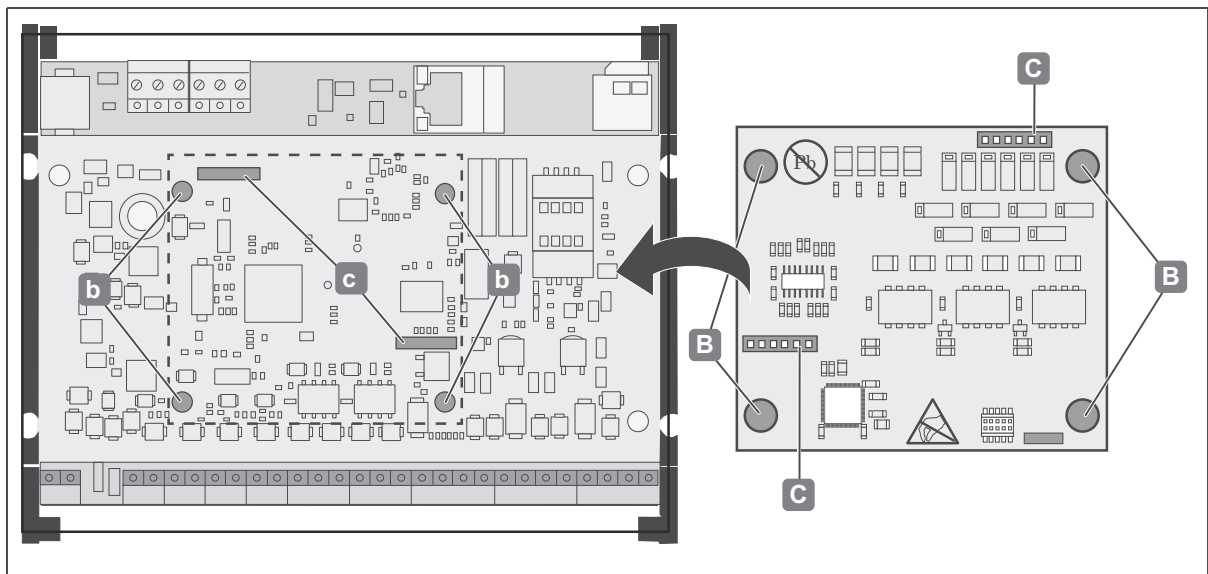
Fig. 9: Montaggio I/O WTX 200 - I/O WTX 200 inserire sul WTC 200 controller
