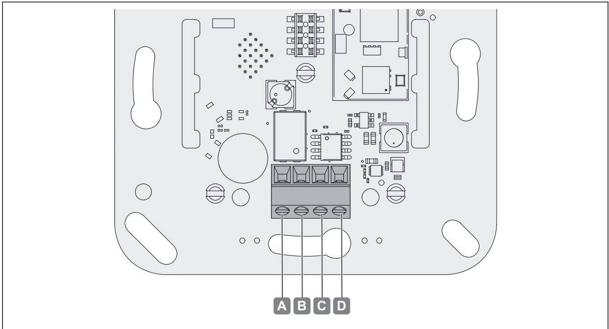
Ilustr. 13: Conexiones WRU 400 / WRU 410
