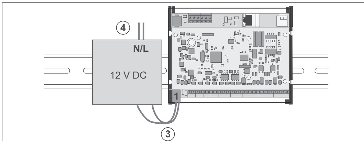
Fig. 6: Instalação do WTC 200
