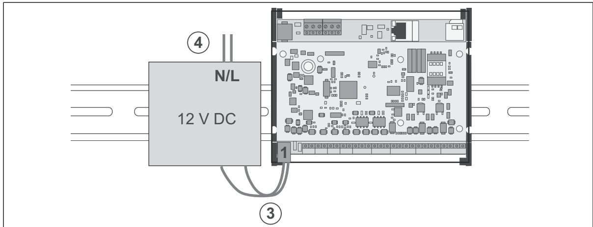
Fig. 6: Montaggio WTC 200
