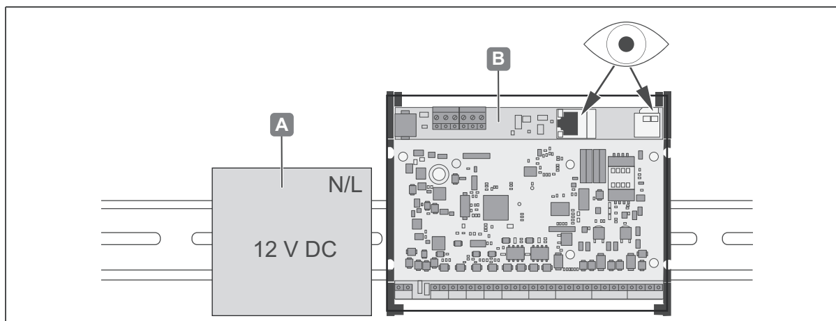
Ilustr. 5: Montaje WTC 200
