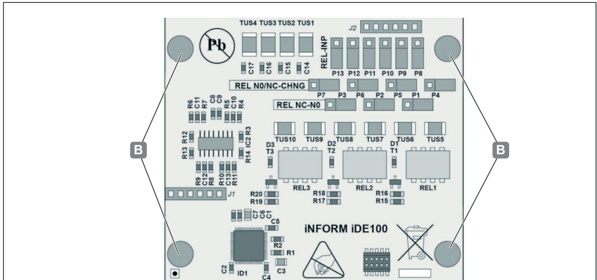
Ilustr. 8: Montaje I/O WTX 200 - montar el distanciador
