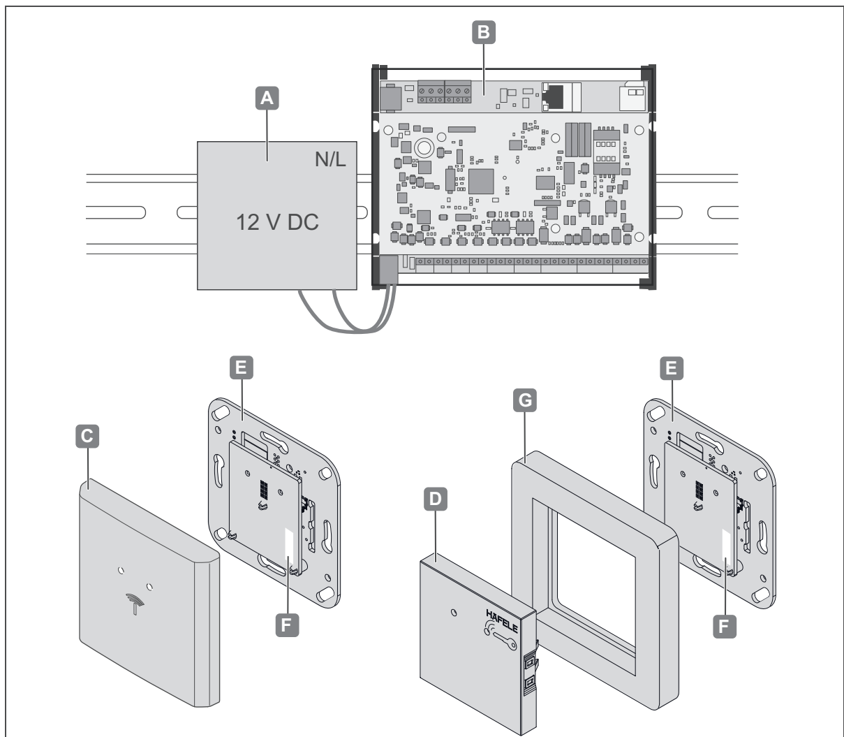
Fig. 1: Panoramica del sistema
