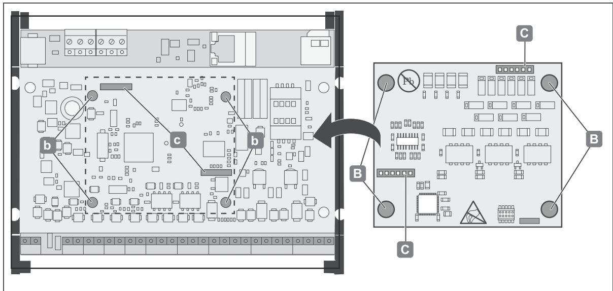
Abb. 9: Montage I/O WTX 200 - I/O WTX 200 auf Controller WTC 200 aufstecken
