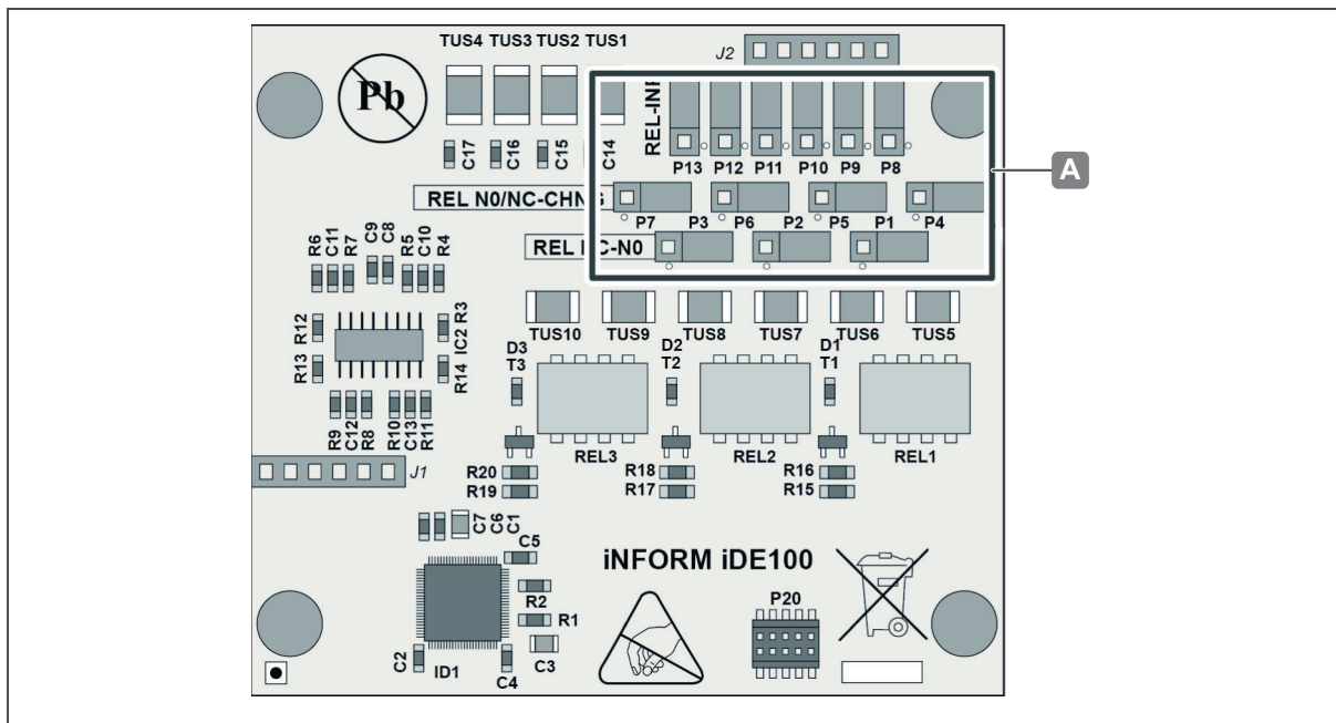
Fig. 18: I/O WTX 200 - Position des cavaliers en cas d'utilisation pour des entrées analogiques/numériques supplémentaires
