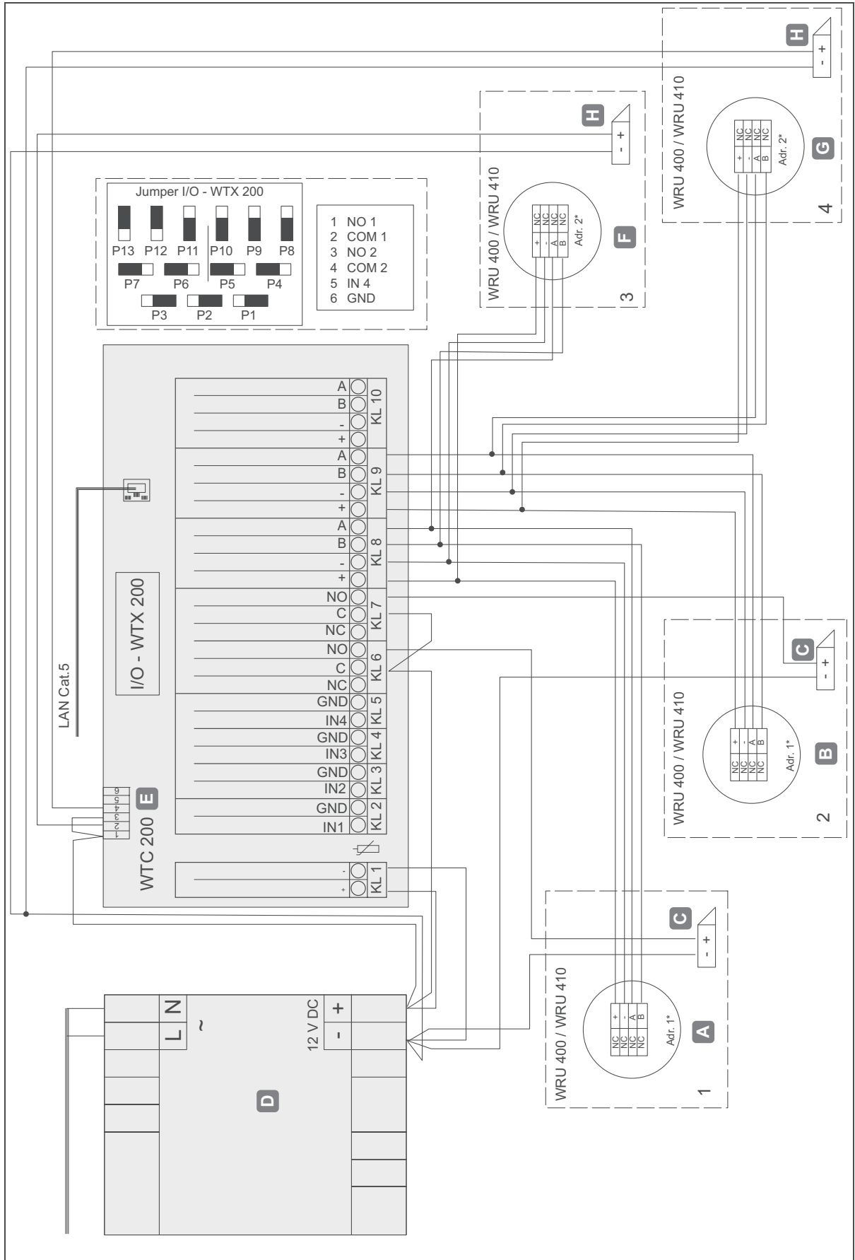
Fig. 33: Schema di cablaggio ad esempio di installazione 5
