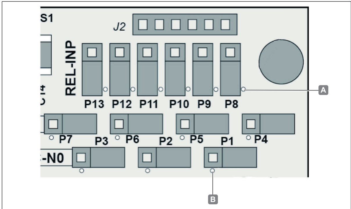
Ilustr. 17: Conexiones I/O WTX 200- posición conexión no. 1 (punto blanco)
