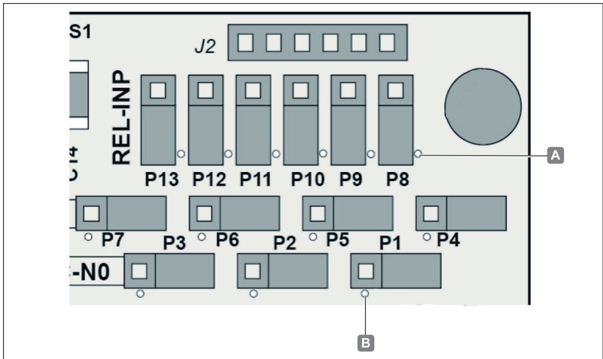
Fig. 17: Connessioni I/O WTX 200- Posizione connessione n° 1 (punto bianco)
