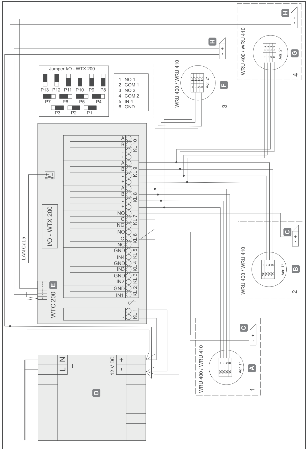
Fig. 33: Diagrama de circuito para o exemplo de instalação 5
