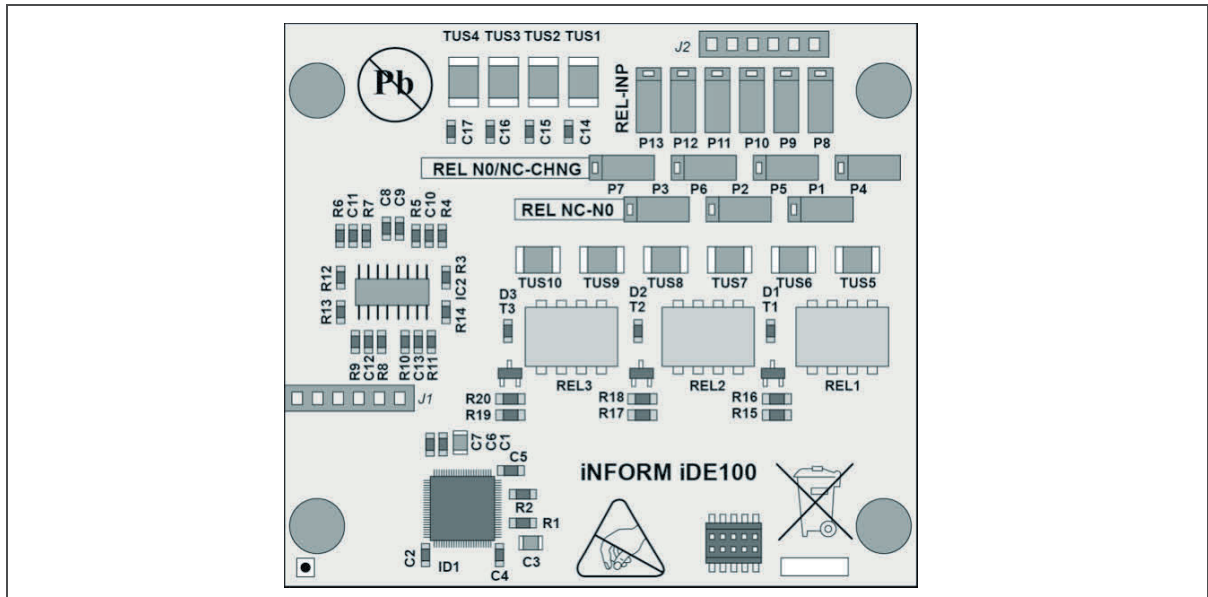
Ilustr. 2: I/O WTX 200
