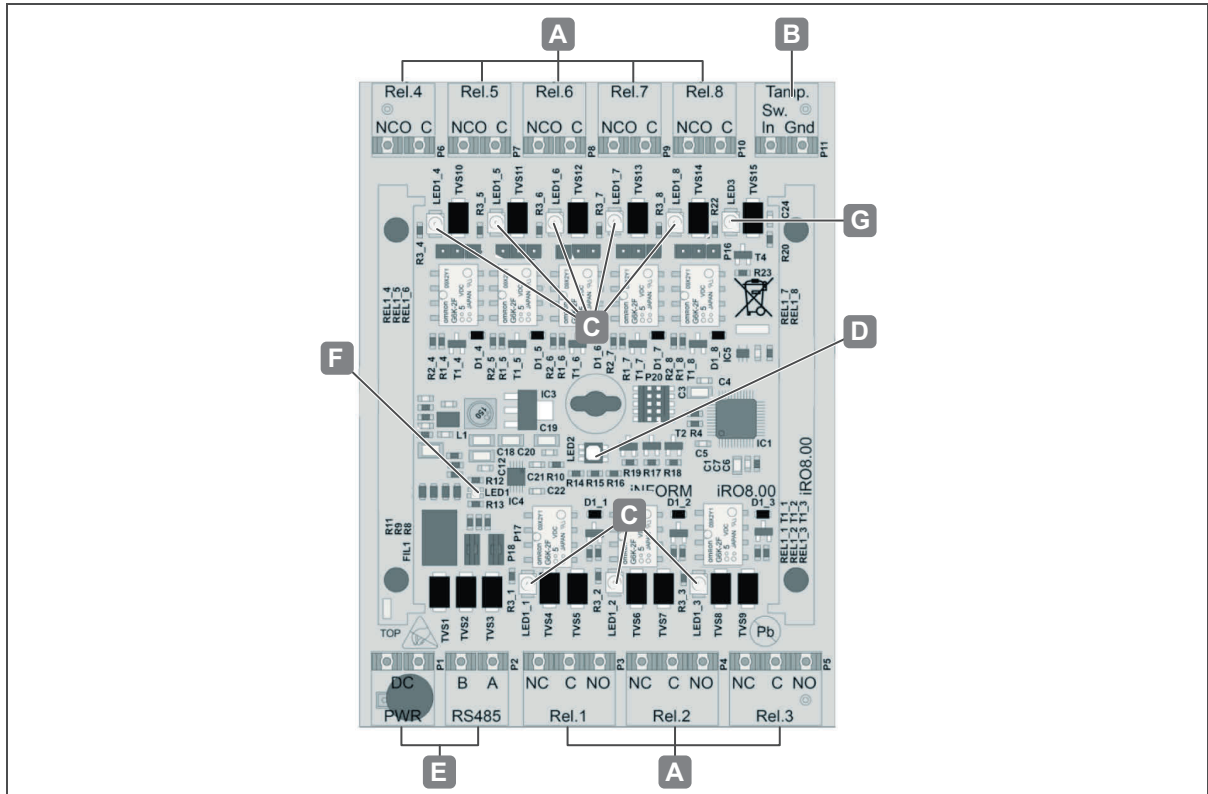
Fig. 20: Ligações com WTX 201
