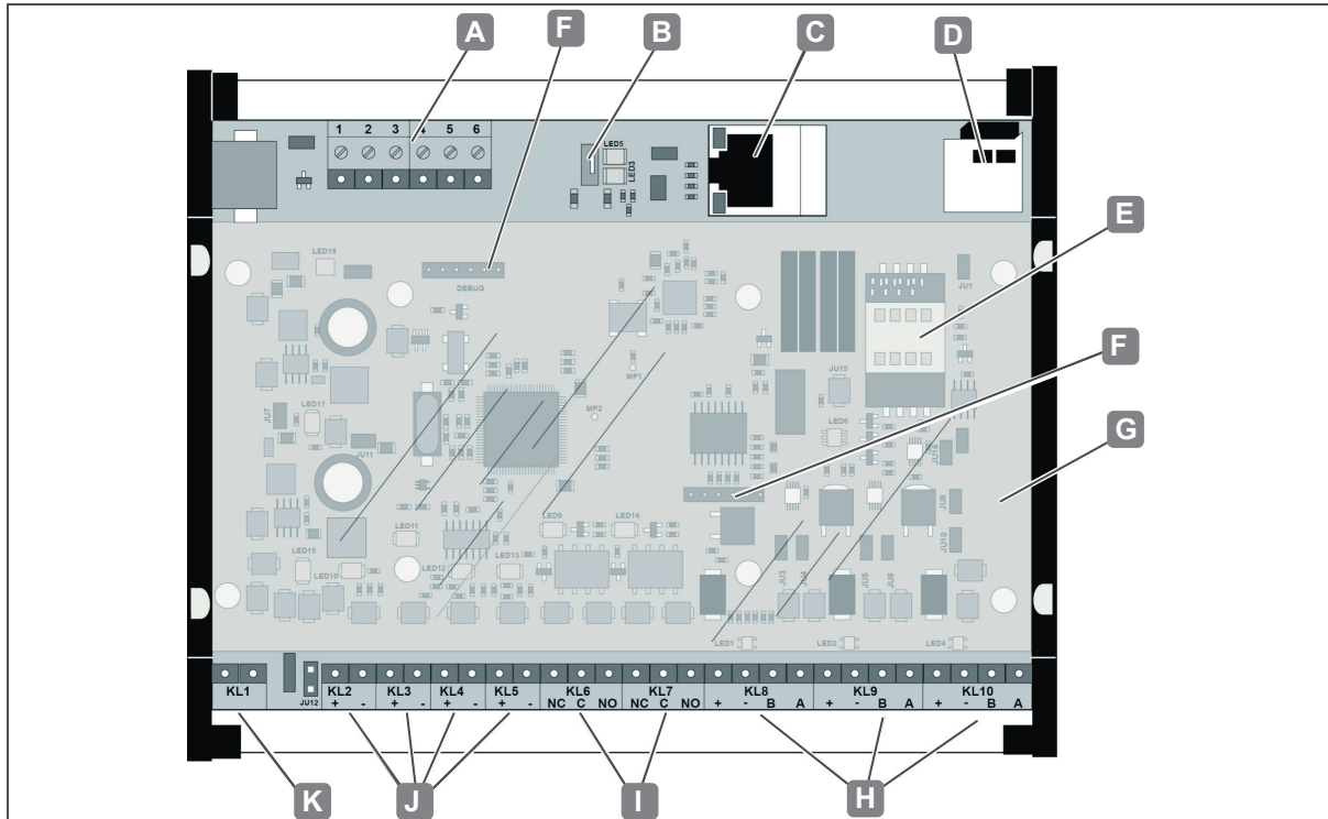
Fig. 14: Connessioni WTC 200
