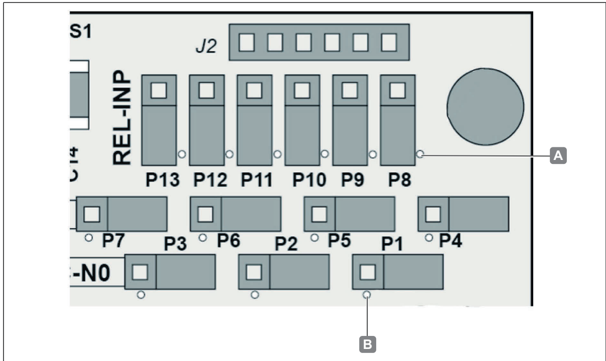
Fig. 17: Ligações no I/O WTX 200 - ligação da posição n.º 1 (ponto branco)
