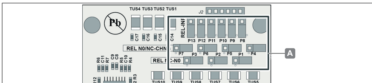
Fig. 7: Montage I/O WTX 200 - mise en place des cavaliers
