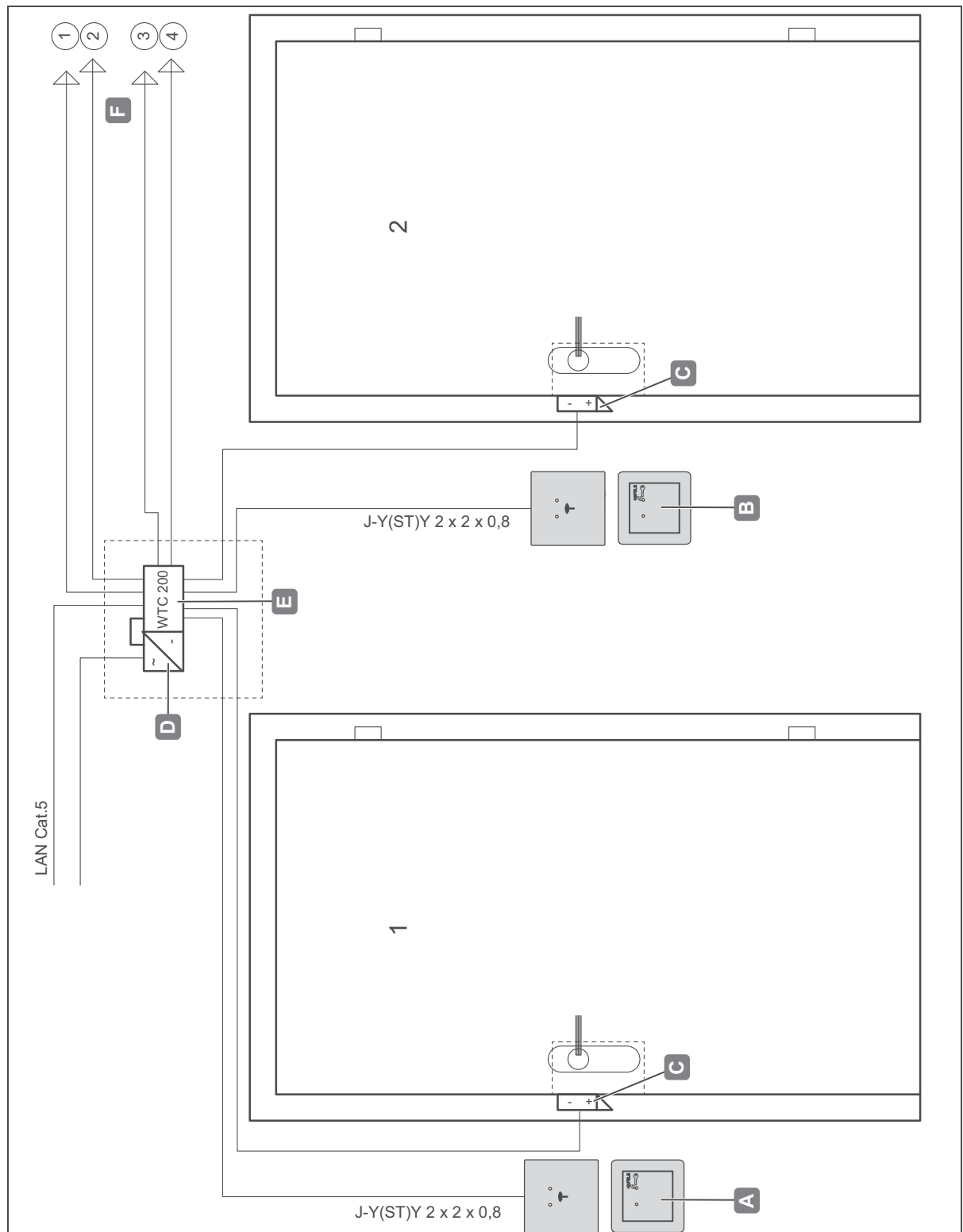
Ilustr. 31: Ejemplo de instalación 5 - parte 1 - Cuatro puertas con un lector cada una / abrepuertas y un controlador (incl. módulo adicional)
