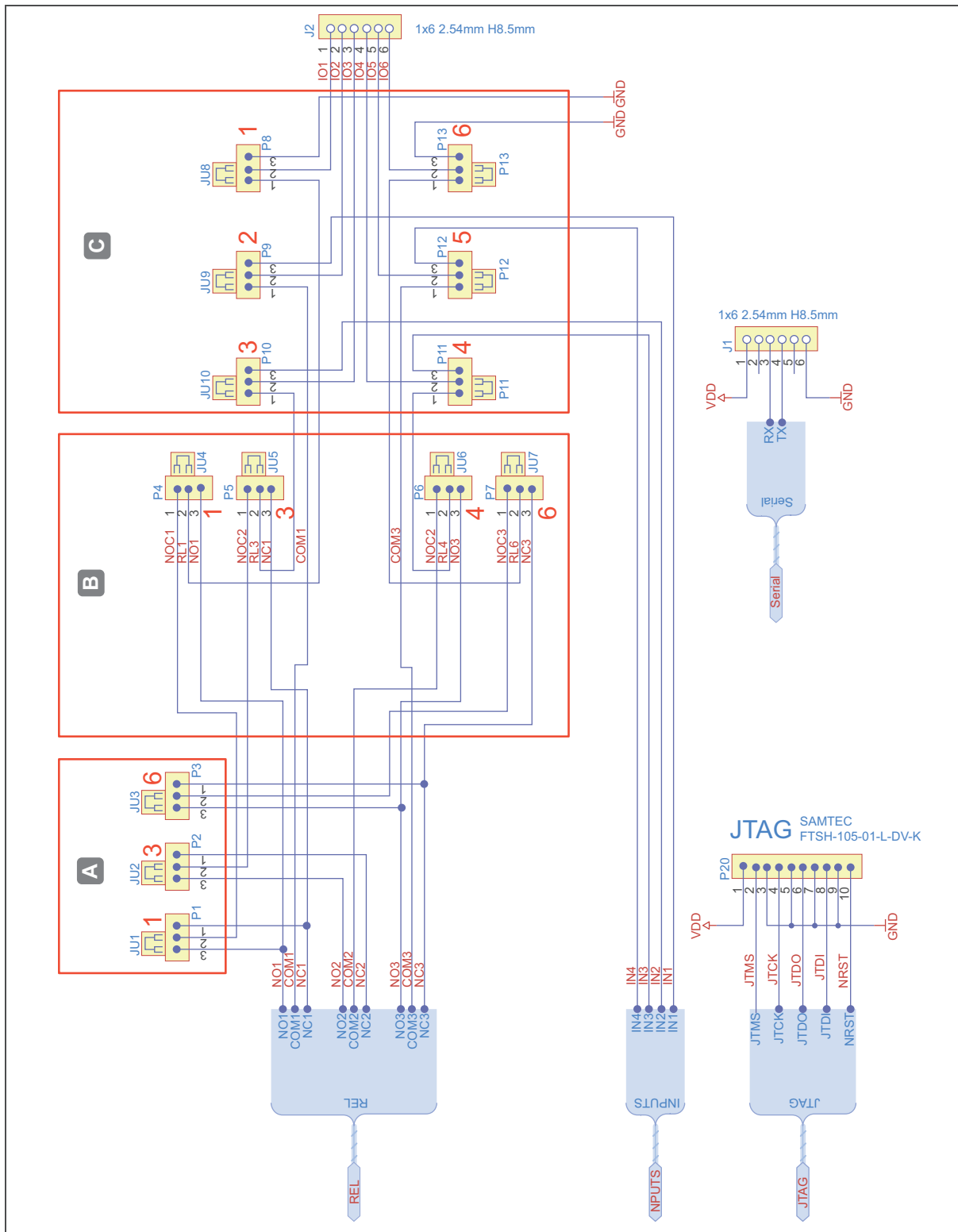
Ilustr. 16: Estructura y asignación de pin del I/O WTX 200
