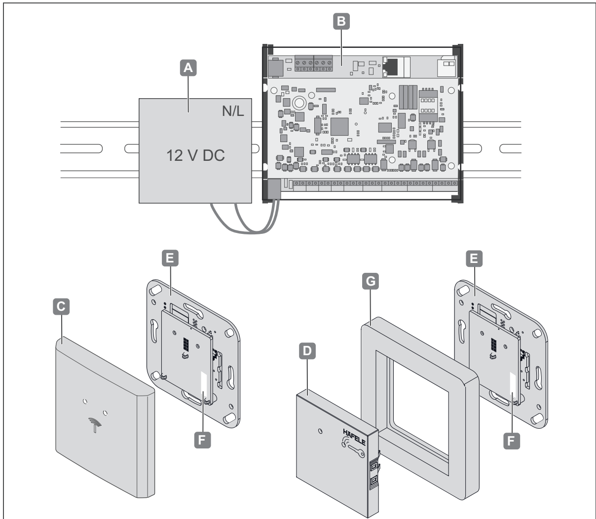
Fig. 1: Vue d'ensemble du système
