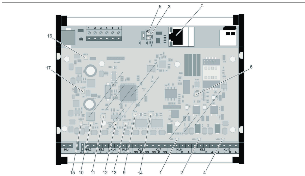
Fig. 12: Aperçu des LED du contrôleur WTC 200
