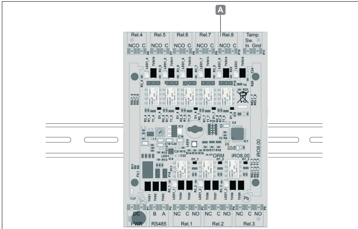
Abb. 11: Montage WTX 201 au Hutschiene
