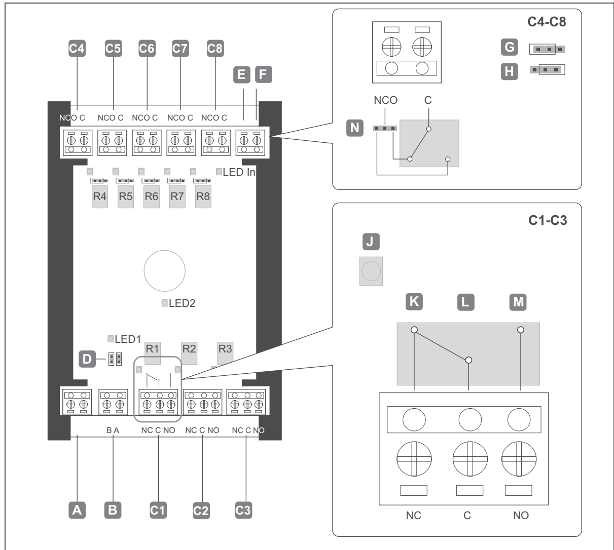
Ilustr. 22: Esquema de conexión módulo de relé óctuple WTX 201
