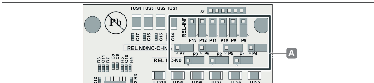
Ilustr. 7: Montaje I/O WTX 200 - conectar los puentes
