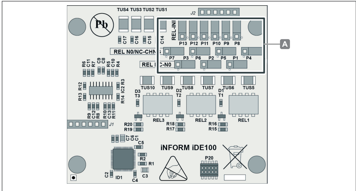
Fig. 18: I/O WTX 200 - posição dos conectores quando utilizado para portas de entrada analógicas/digitais
