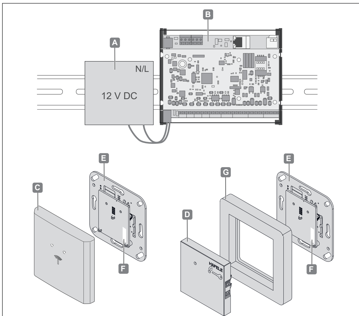
Fig. 1: Visão geral do sistema
