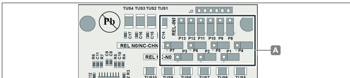
Fig. 7: Instalação do I/O WTX 200 – configuração do conector
