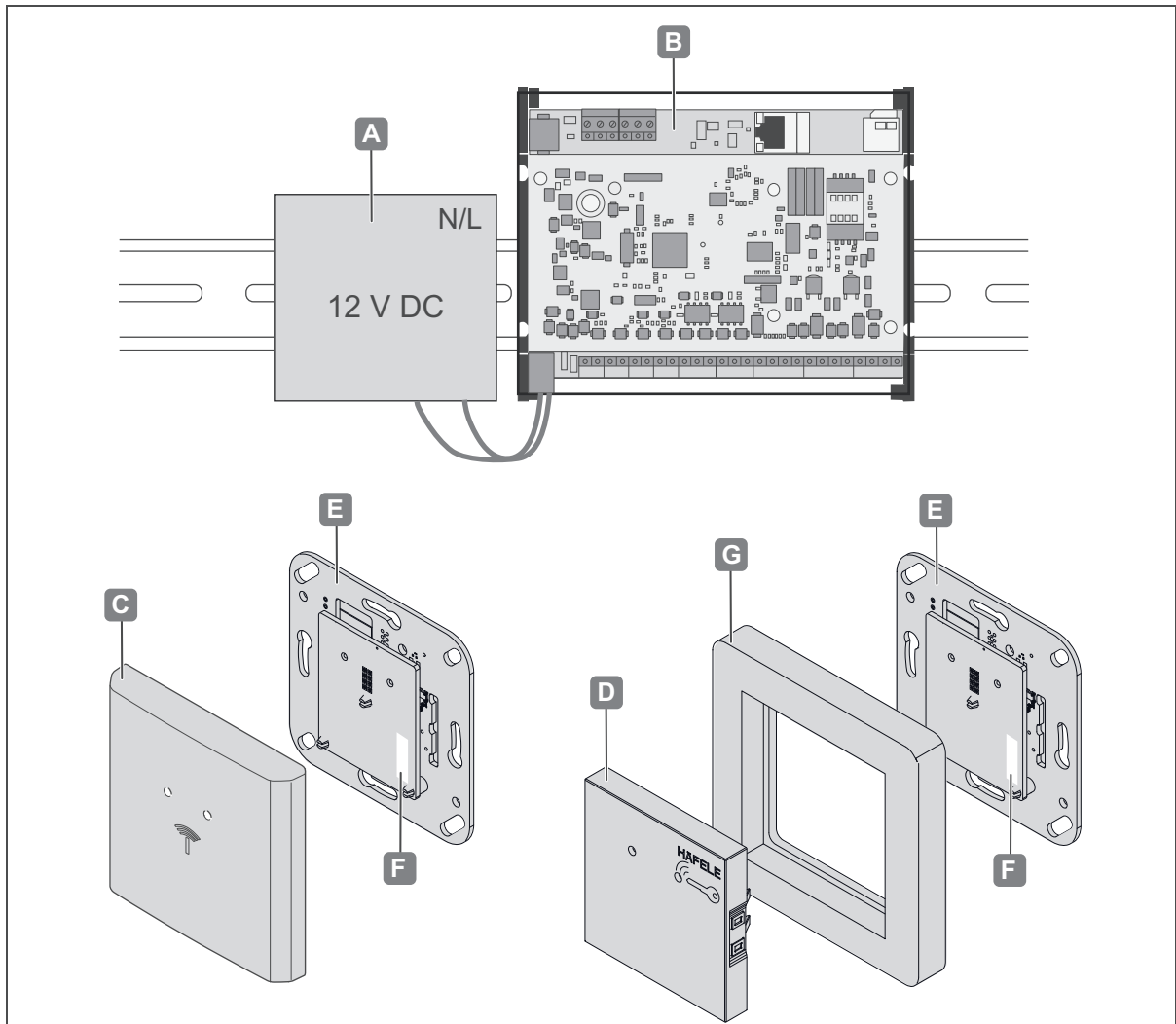
Abb. 1: Systemübersicht
