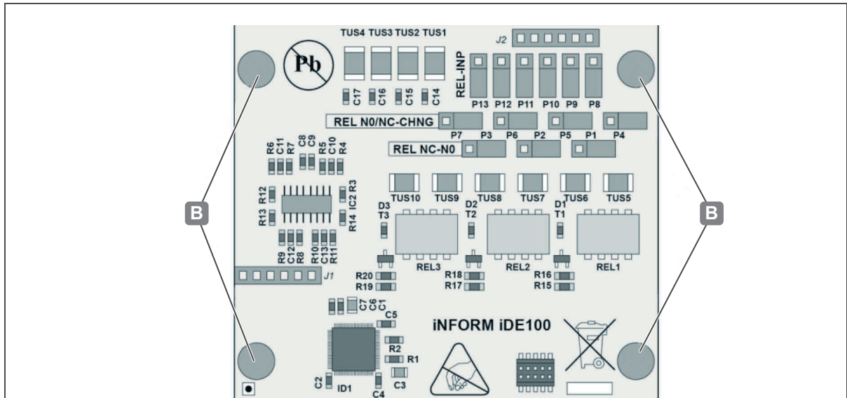
Abb. 8: Montage I/O WTX 200 - Abstandshalter anbringen
