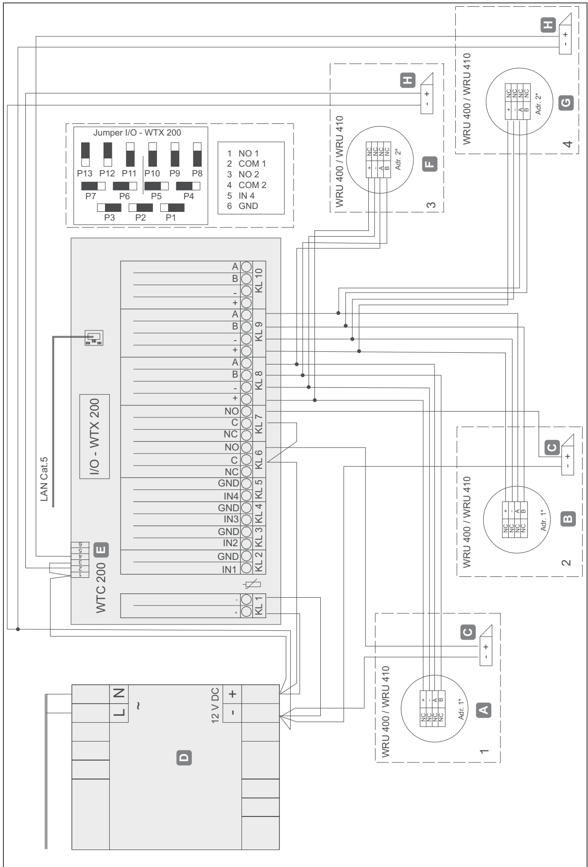
Fig. 33: Schéma de connexions pour l'exemple d'installation 5
