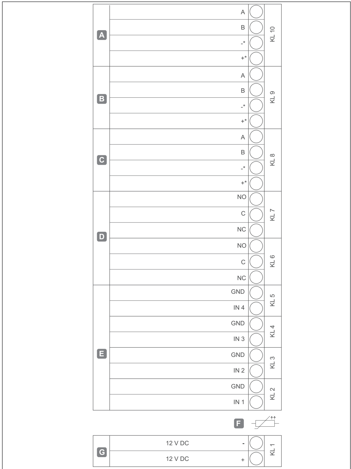
Fig. 21: Affectation des bornes du contrôleur WTC 200
