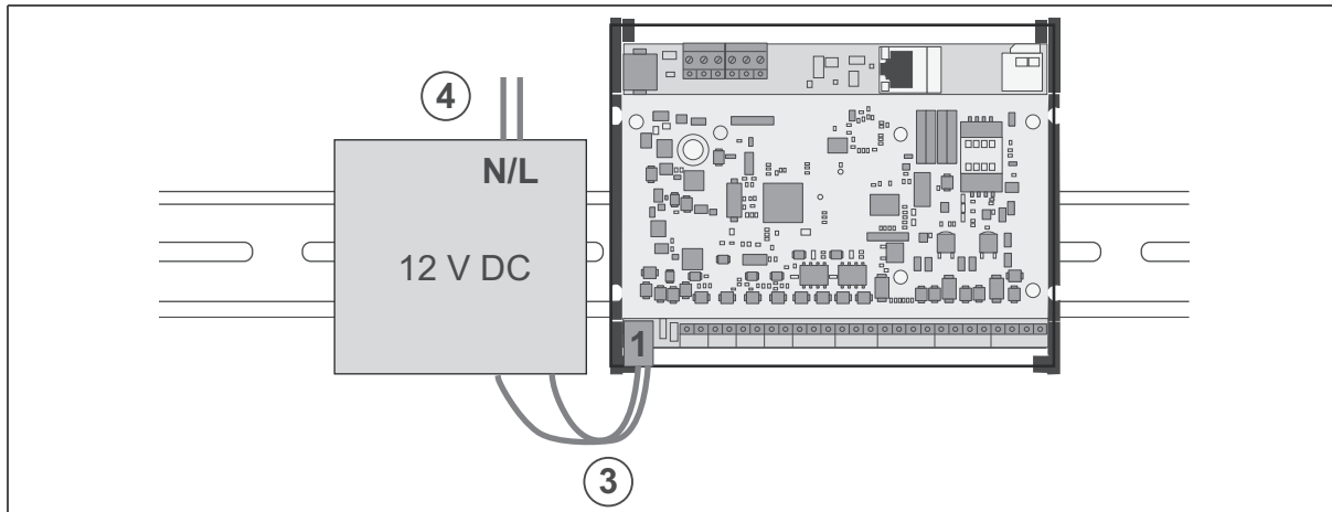
Ilustr. 6: Montaje WTC 200
