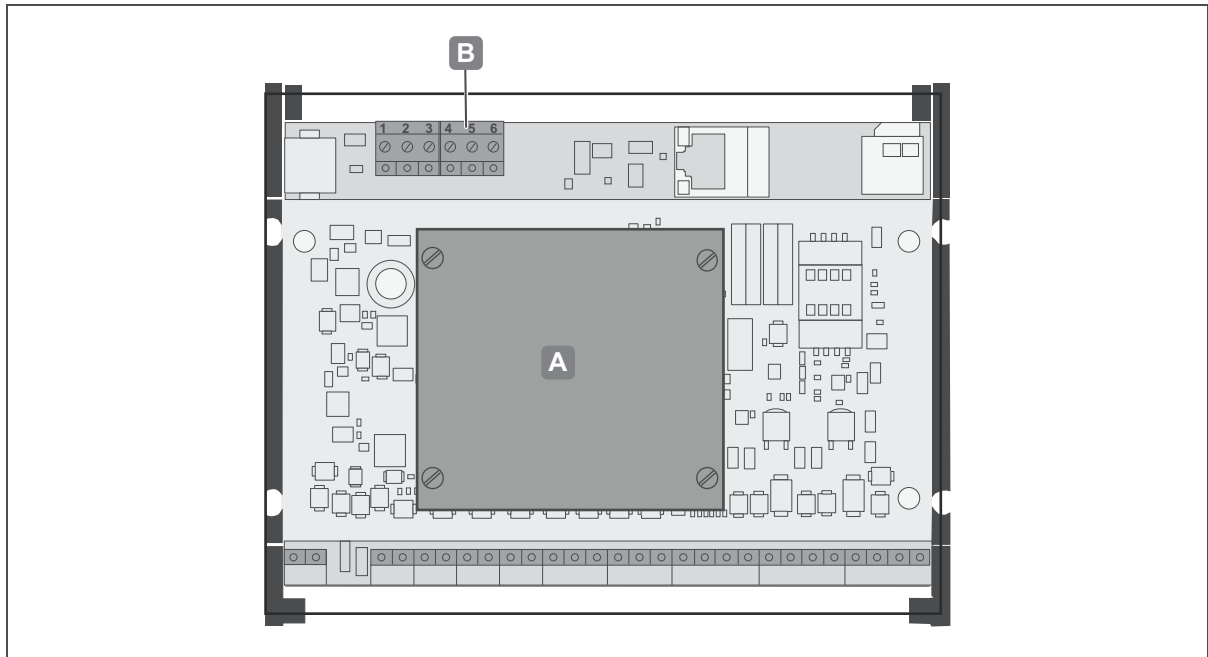
Fig. 15: Connessioni I/O WTX 200
