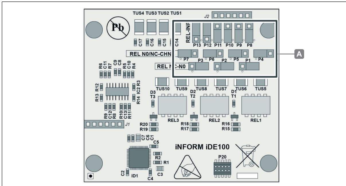
Fig. 19: I/O WTX 200 - Position des cavaliers en cas d'utilisation pour 2 sorties relais supplémentaires et 1 entrée analogique/numérique supplémentaire
