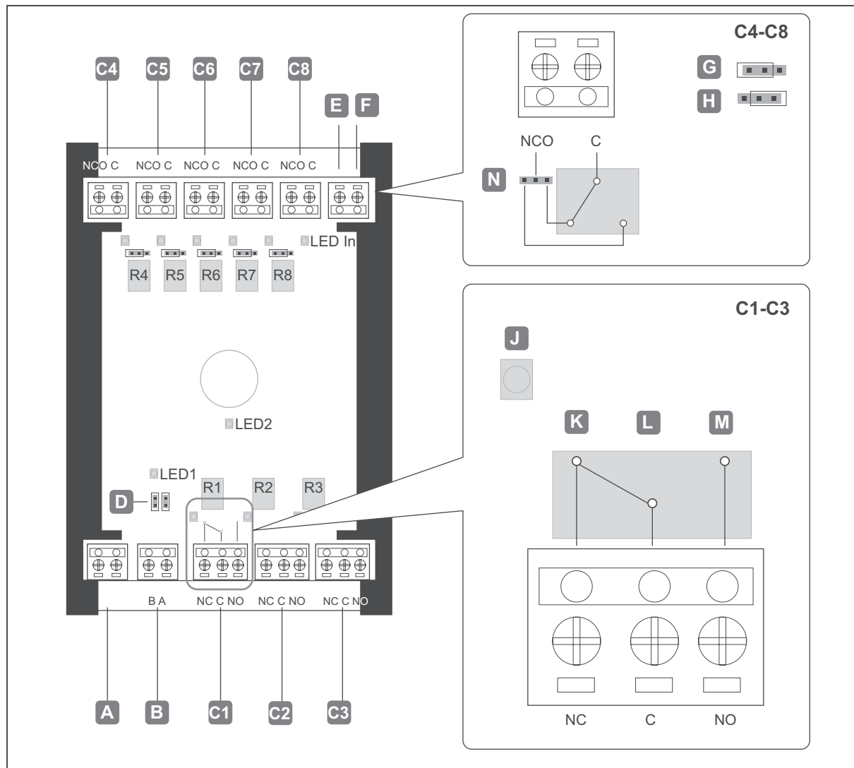
Fig. 22: Schema di collegamento modulo relè a 8 vie WTX 201
