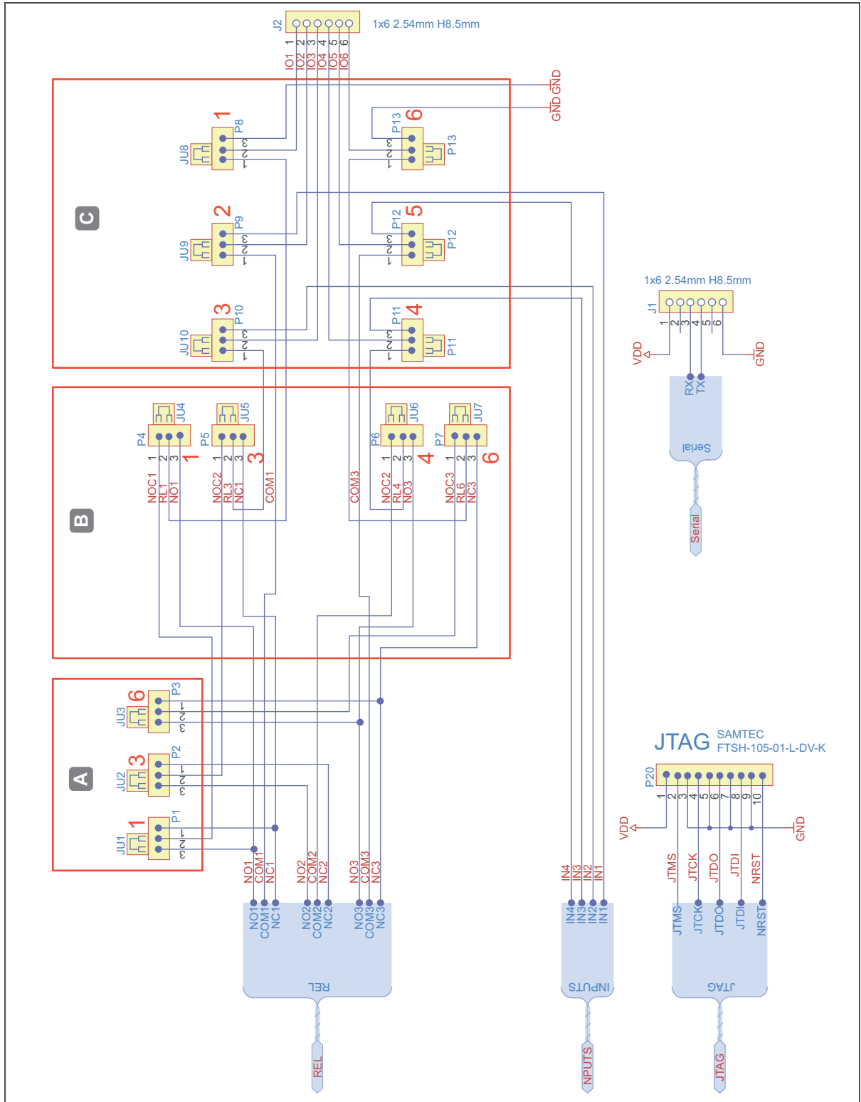
Fig. 16: Struttura e assegnazione pin del I/O WTX 200
