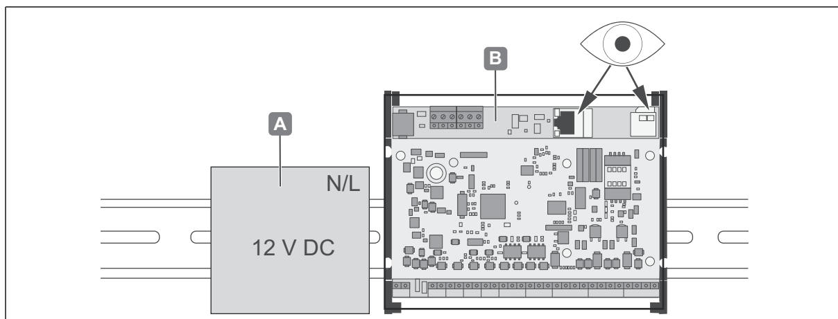
Fig. 5: Instalação do WTC 200
