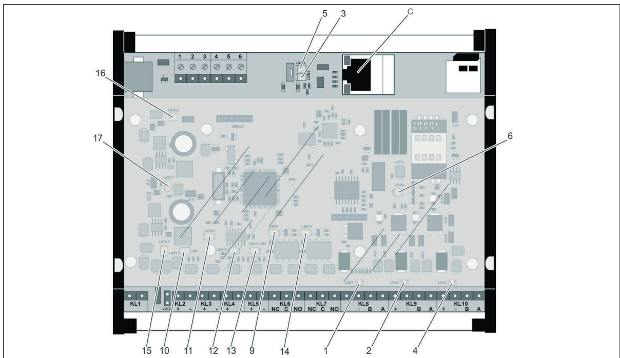
Abb. 12: Übersicht LEDs am Controller WTC 200
