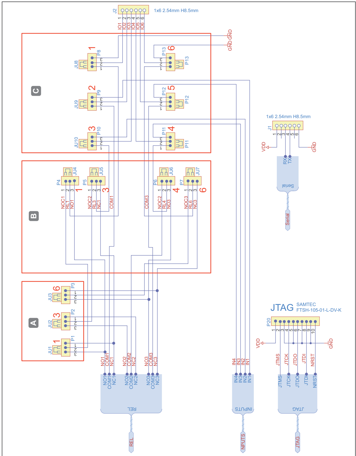
Fig. 16: Estrutura e atribuição de pinos do I/O WTX 200
