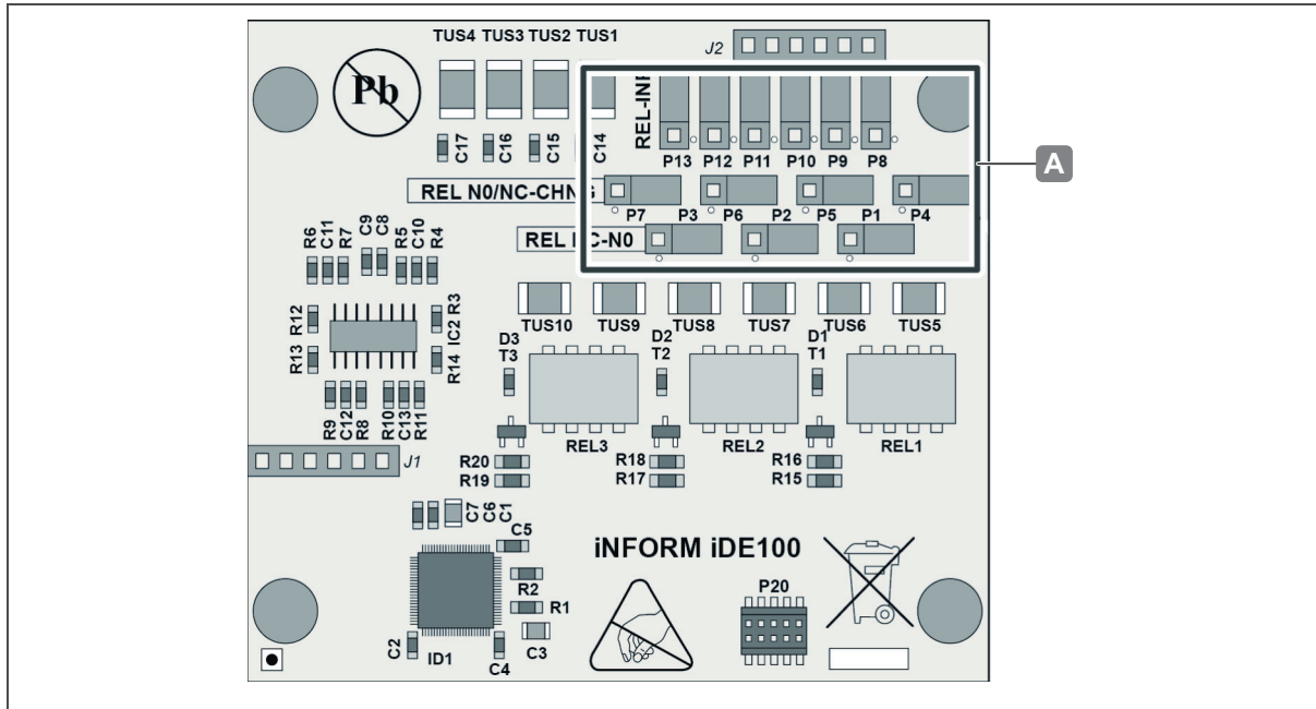
Fig. 18: I/O WTX 200 - Posizione dei ponticelli in caso di utilizzo per altri ingressi analogici/digitali
