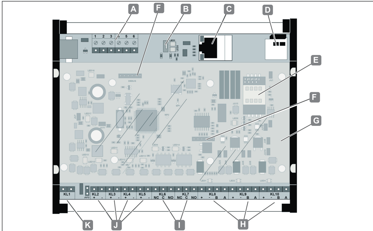
Fig. 14: Ligações no WTC 200
