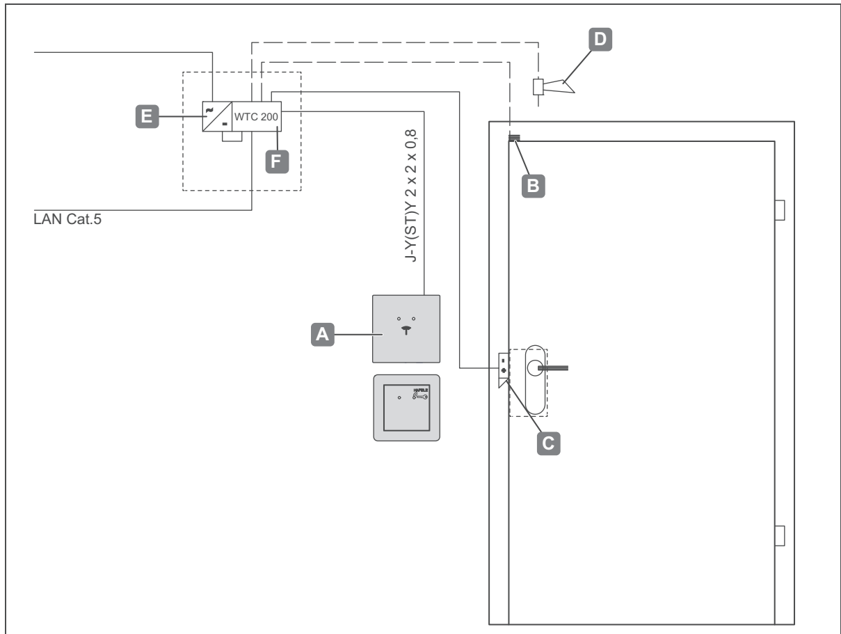
Ilustr. 23: Ejemplo de instalación 1 - Una puerta con un lector, contacto auxiliar de estado de puerta, abrepuertas, emisor de señal y controlador
