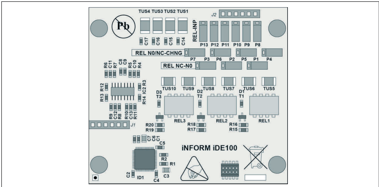
Abb. 2: I/O WTX 200
