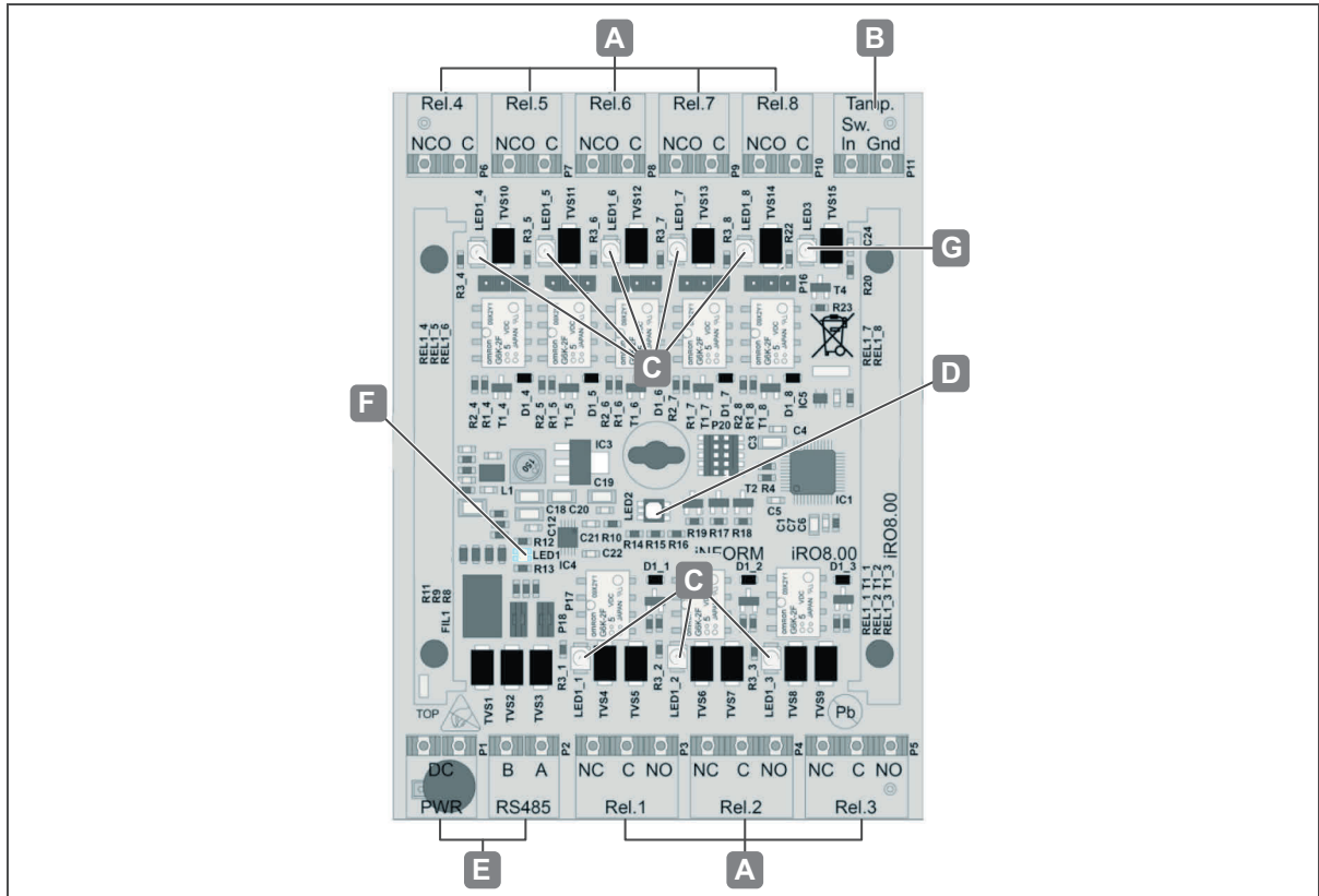
Fig. 20: Connessioni WTX 201
