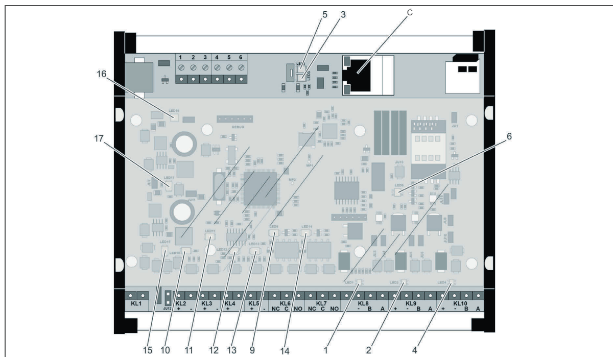
Fig. 12: Visão geral dos LED no controlador WTC 200
