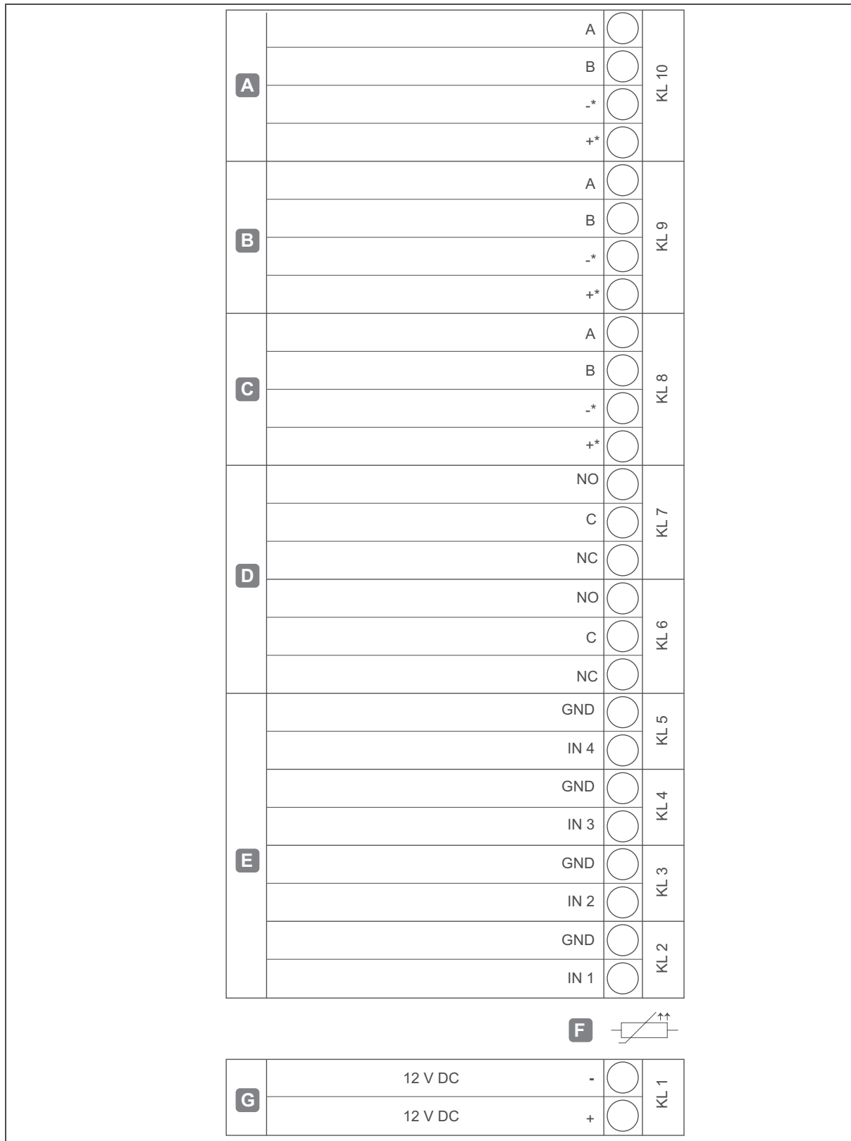
Abb. 21: Klemmenbelegung Controller WTC 200
