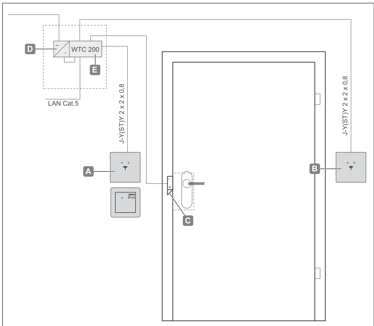
Fig. 27: Exemple d'installation 3 - Une porte avec deux lecteurs (par ex. intérieur et extérieur), gâche électrique et contrôleur
