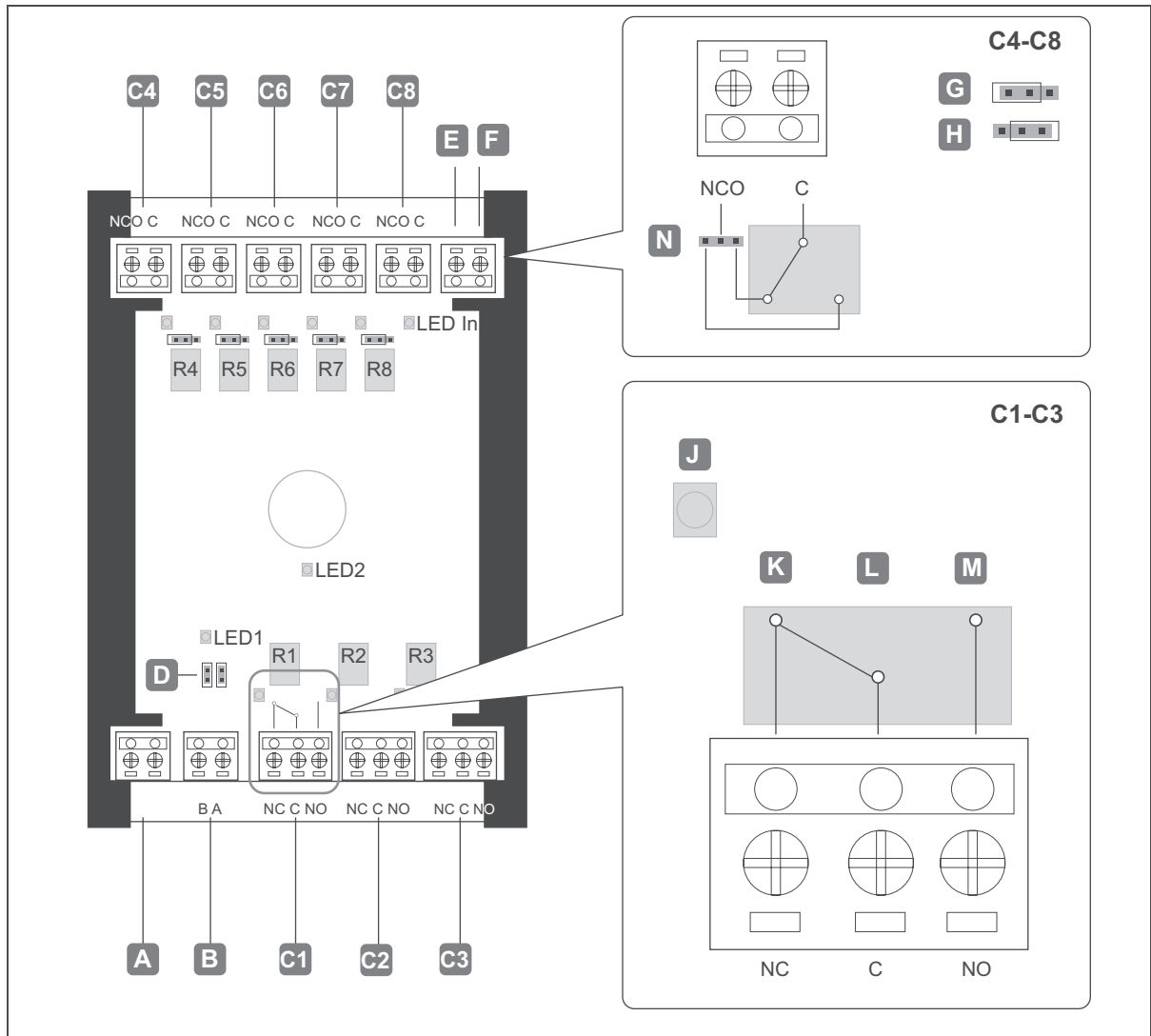
Fig. 22: Plan de raccordement du module relais à 8 voies WTX 201
