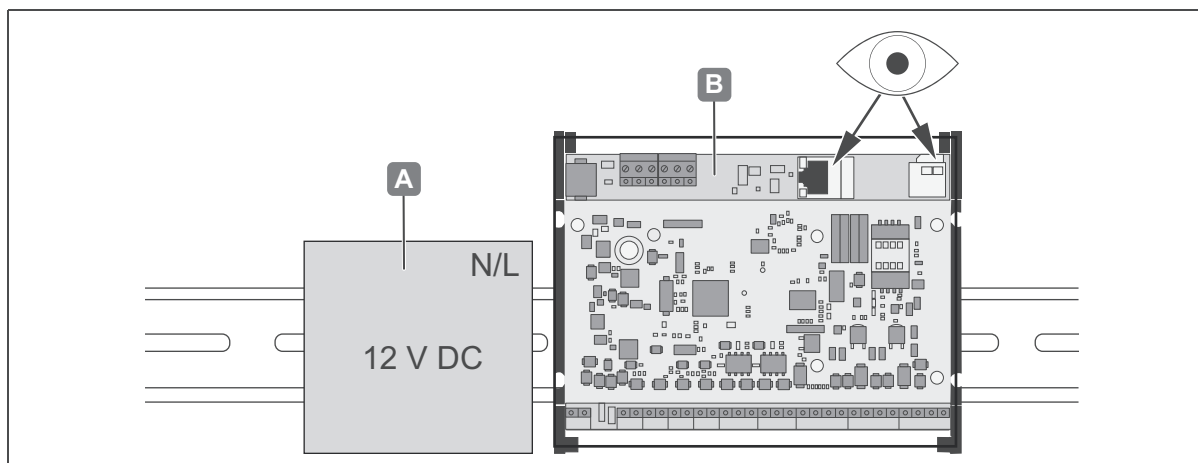
Fig. 5: Montaggio WTC 200
