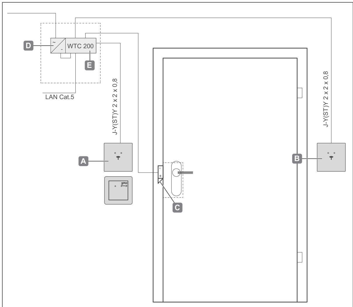
Fig. 27: Exemplo de instalação 3 – porta com dois leitores (por ex., no interior e no exterior), testa elétrica e controlador
