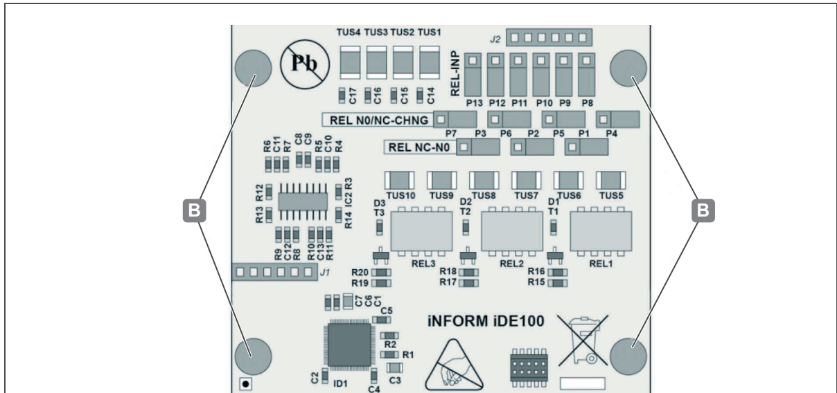
Fig. 8: Instalação do I/O WTX 200 – instalação de espaçadores
