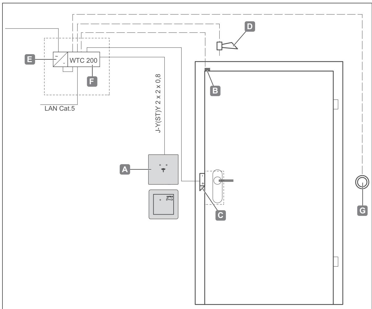
Abb. 25: Installationsbeispiel 2 - Eine Tür mit einem Leser, Türmeldekontakt, Türöffner, Signalgeber, Türöffnertaster und Controller
