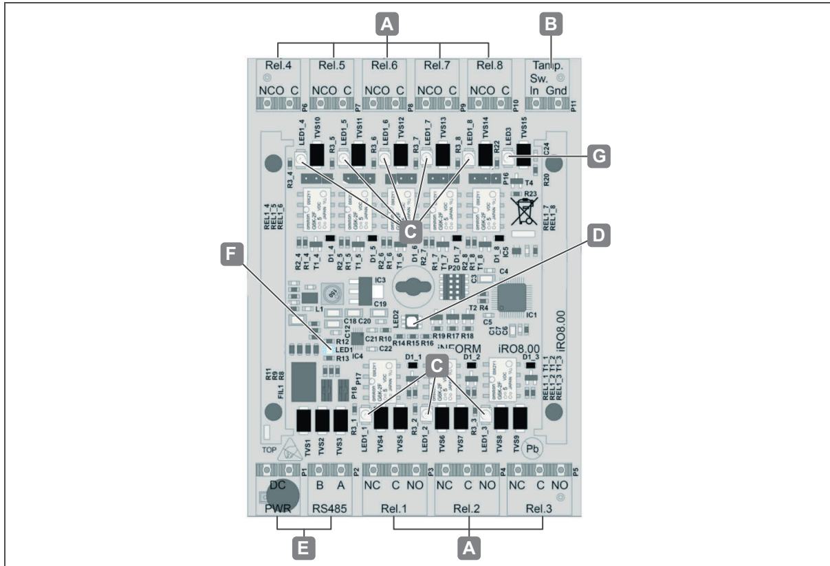
Ilustr. 20: Conexiones WTX 201
