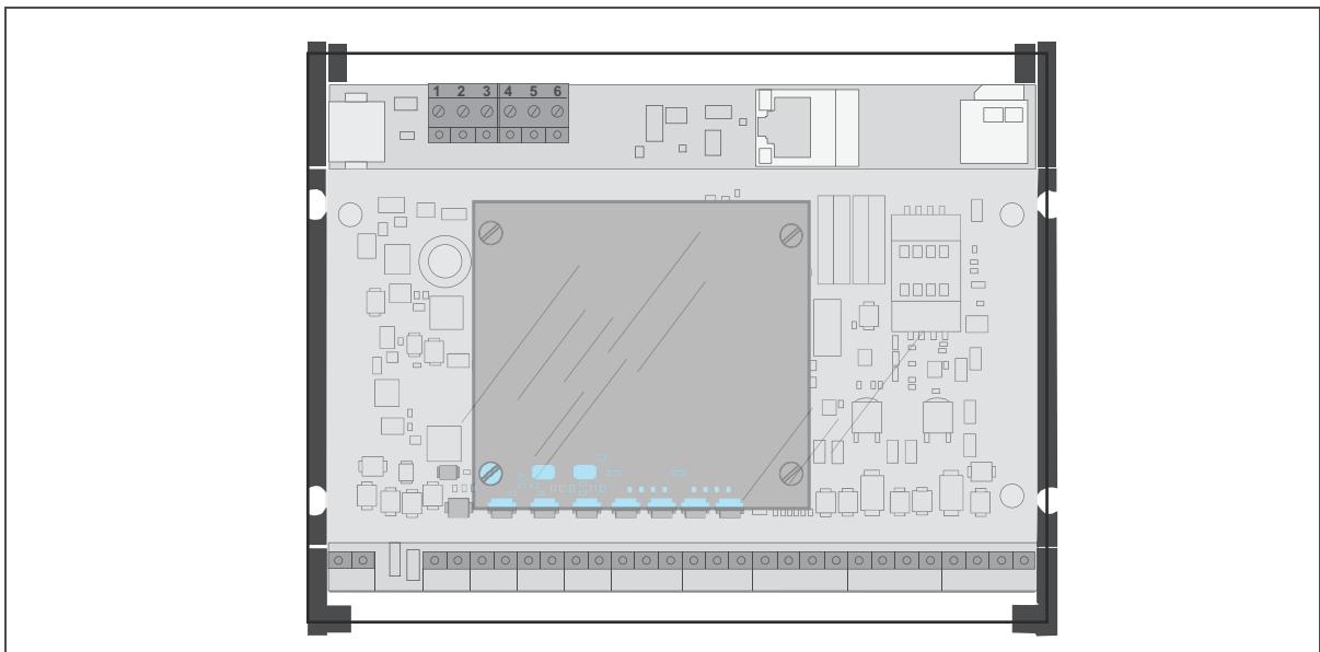
Abb. 3: I/O WTX 200 - auf Controller aufgesteckt
