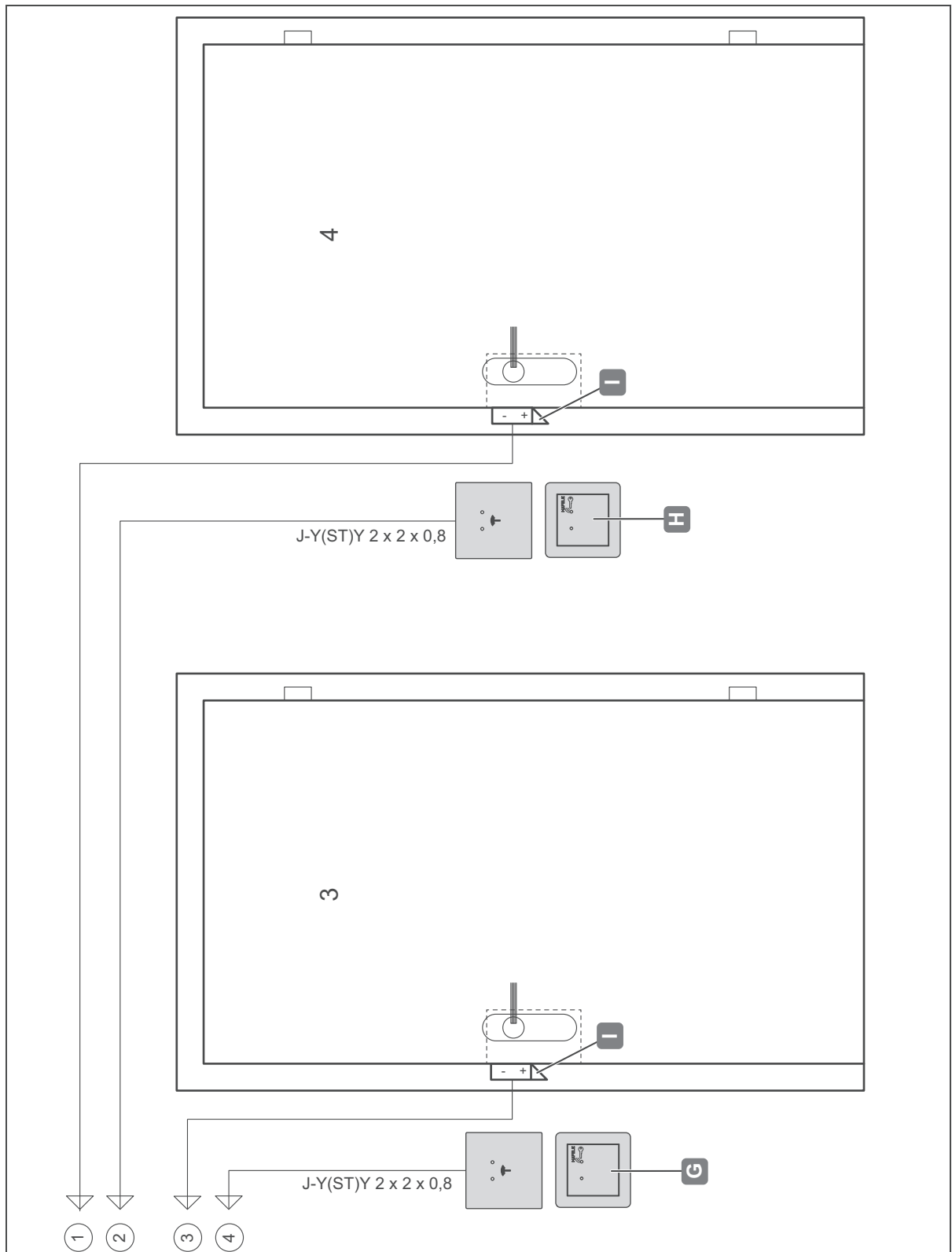
Fig. 32: Exemplo de instalação 5 – parte 2 – quatro portas com um leitor/testa elétrica e um controlador cada (incluindo módulo adicional)
