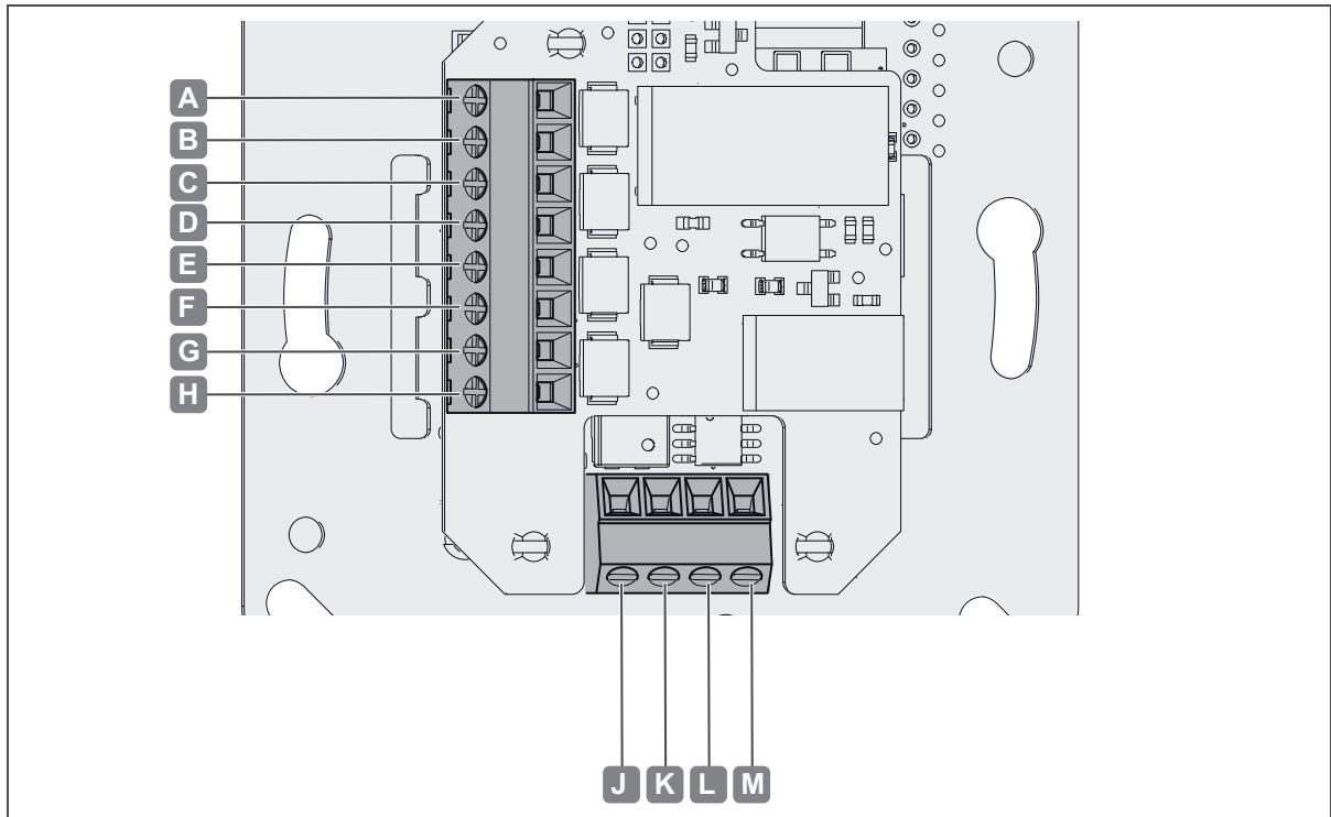
Fig. 2: Ligações
