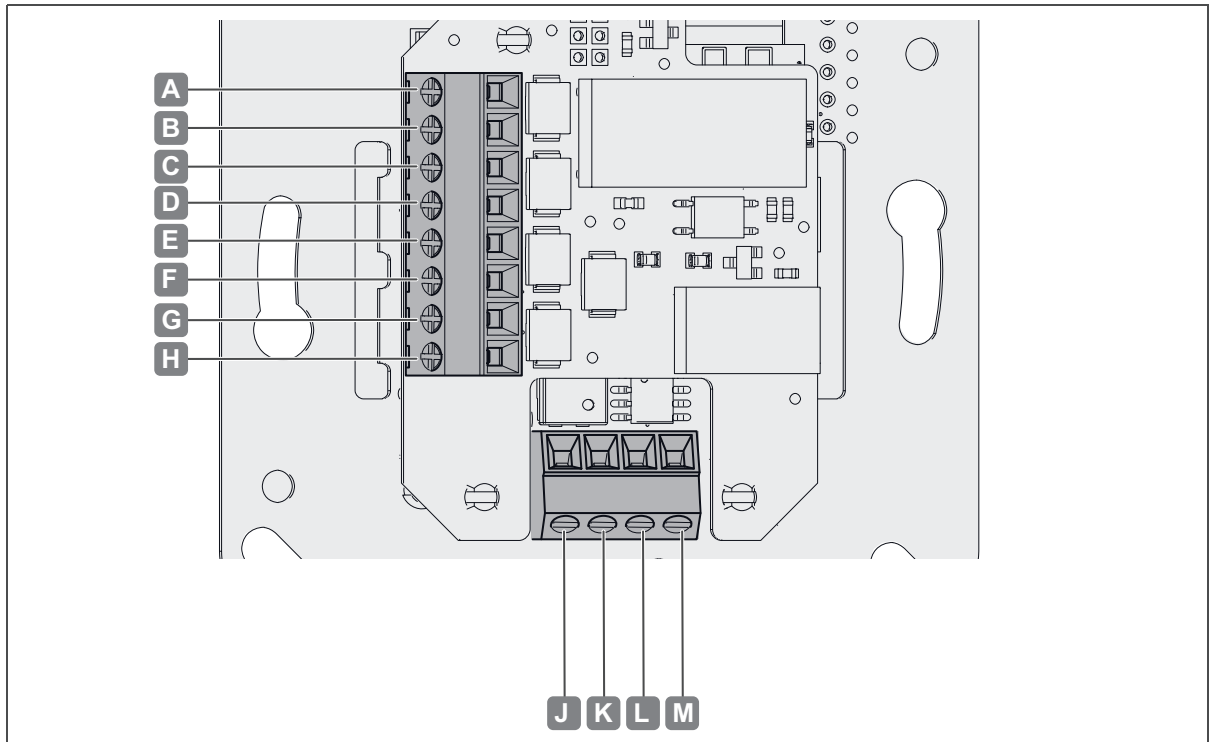
Fig. 2: Connessioni
