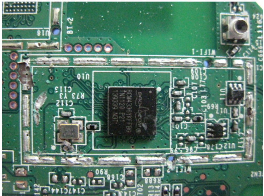
(3) EUT Photo
