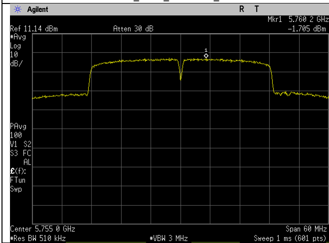
5755MHz_151_40MHz_n-mode
