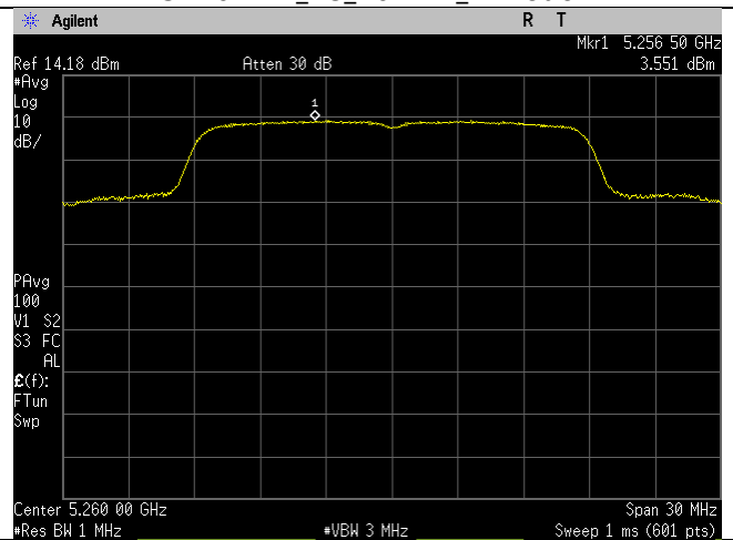
5260MHz_52_20MHz_n-mode
