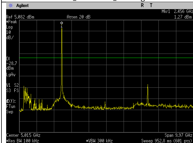
WIFI_High Ch_2462MHz_20MHz BW_ax-mode_-30dBc_30MHz-10GHz_Port 1.gif
