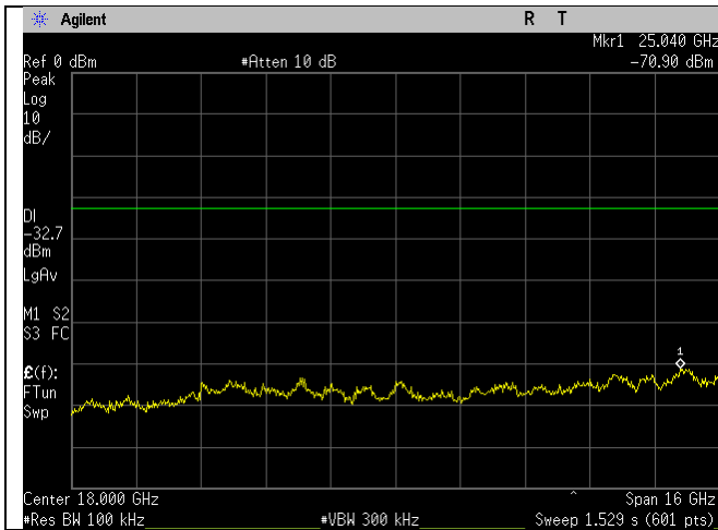
WIFI_Low Ch_2412MHz_20MHz BW_g-mode_- 30dBc_10-26GHz_Port 1.gif
