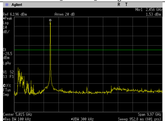
WIFI_High Ch_2462MHz_20MHz BW_ax-mode_-30dBc_30MHz-10GHz_Port 2.gif
