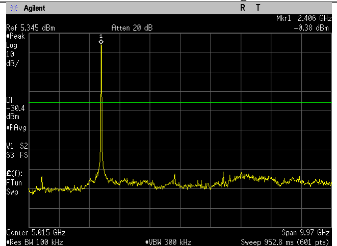
WIFI_Low Ch_2412MHz_20MHz BW_g-mode_- 30dBc_30MHz-10GHz_Port 2.gif
