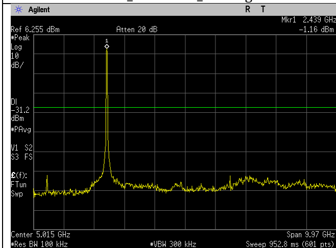
WIFI_Mid Ch_2437MHz_40MHz BW_ax-mode_- 30dBc_30MHz-10GHz_Port 2.gif
