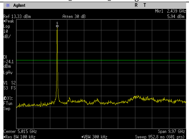
WIFI_Mid Ch_2437MHz_20MHz BW_g-mode_-30dBc_30MHz-10GHz_Port 2.gif
