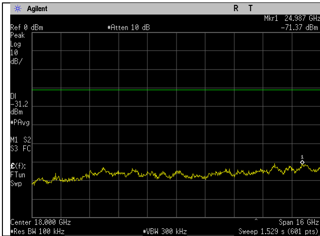
WIFI_Mid Ch_2437MHz_40MHz BW_ax-mode_- 30dBc_10-26GHz_Port 2.gif
