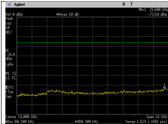
WIFI_High Ch_2462MHz_20MHz BW_b-mode_- 30dBc_10-26GHz_Port 1.gif
