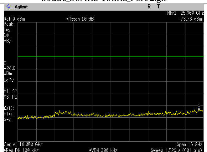
WIFI_Low Ch_2412MHz_20MHz BW_ax-mode_-30dBc_10-26GHz_Port 2.gif
