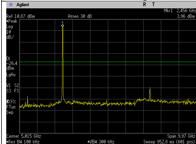
WIFI_High Ch_2462MHz_20MHz BW_b-mode_- 30dBc_30MHz-10GHz_Port 1.gif
