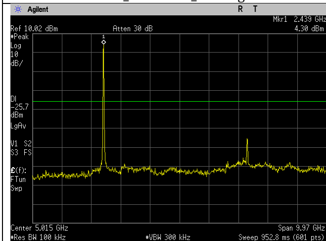
WIFI_Mid Ch_2437MHz_20MHz BW_g-mode_-30dBc_30MHz-10GHz_Port 1.gif
