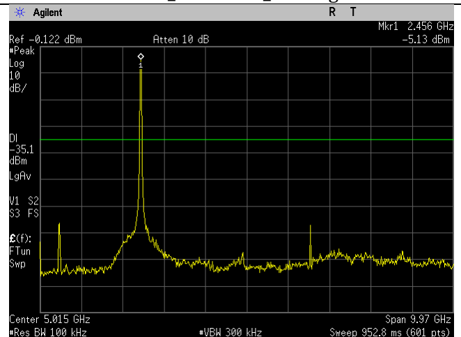
WIFI_High Ch_2452MHz_40MHz BW_n-mode- 30dBc_30MHz-10GHz_Port 2.gif
