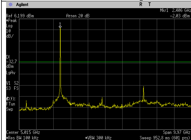
WIFI_Low Ch_2412MHz_20MHz BW_g-mode_- 30dBc_30MHz-10GHz_Port 1.gif
