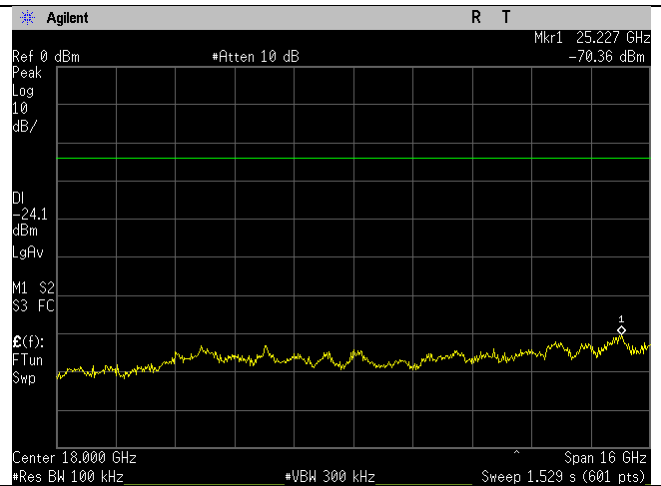
WIFI_Mid Ch_2437MHz_20MHz BW_g-mode_-30dBc_10-26GHz_Port 2.gif
