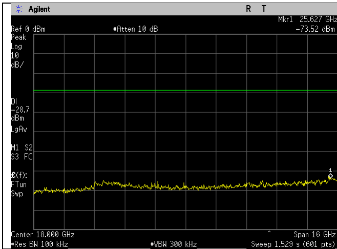
WIFI_High Ch_2462MHz_20MHz BW_ax-mode_-30dBc_10-26GHz_Port 1.gif
