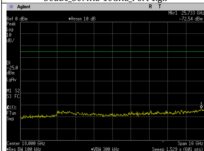
WIFI_Low Ch_2412MHz_20MHz BW_ax-mode_-30dBc_10-26GHz_Port 1.gif
