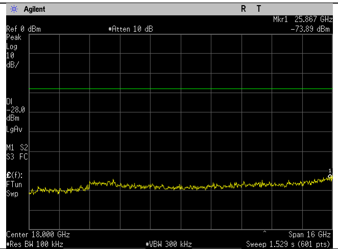
WIFI_High Ch_2462MHz_20MHz BW_b-mode_- 30dBc_10-26GHz_Port 2.gif
