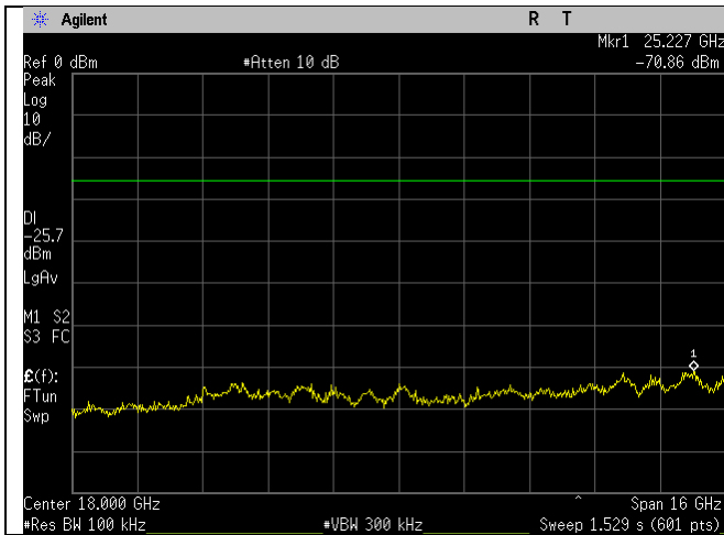
WIFI_Mid Ch_2437MHz_20MHz BW_g-mode_-30dBc_10-26GHz_Port 1.gif
