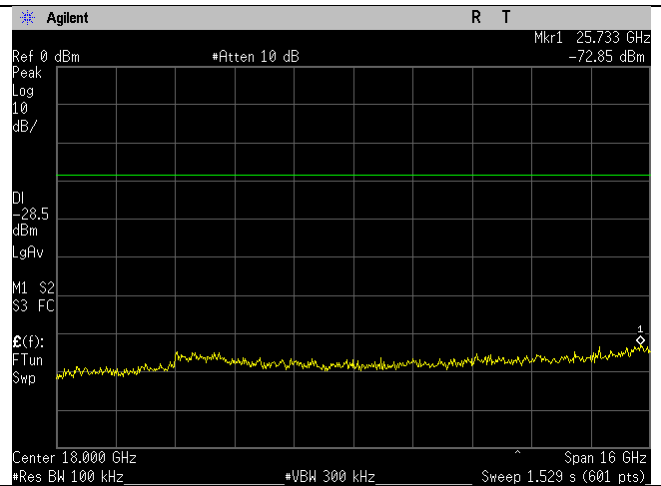
WIFI_High Ch_2462MHz_20MHz BW_ax-mode_-30dBc_10-26GHz_Port 2.gif
