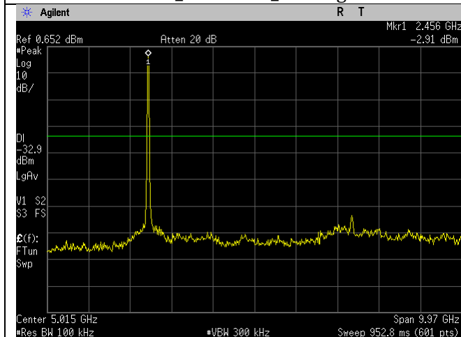
WIFI_High Ch_2452MHz_40MHz BW_n-mode- 30dBc_30MHz-10GHz_Port 1.gif
