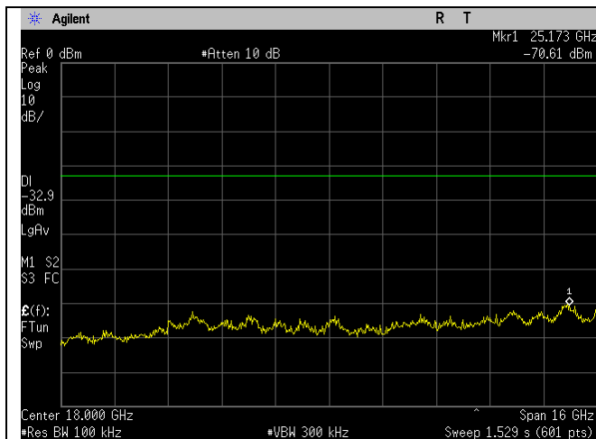
WIFI_High Ch_2452MHz_40MHz BW_n-mode- 30dBc_10-26GHz_Port 1.gif
