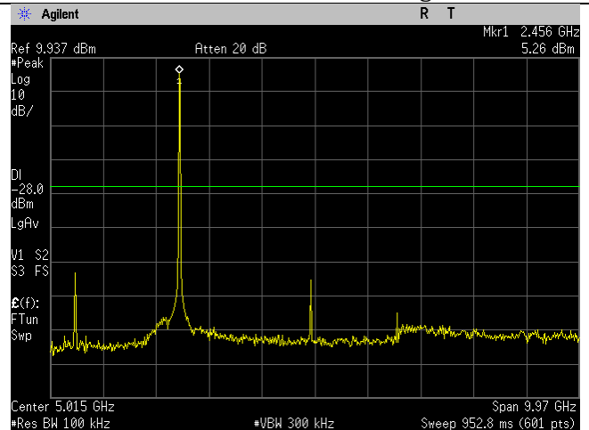
WIFI_High Ch_2462MHz_20MHz BW_b-mode_- 30dBc_30MHz-10GHz_Port 2.gif
