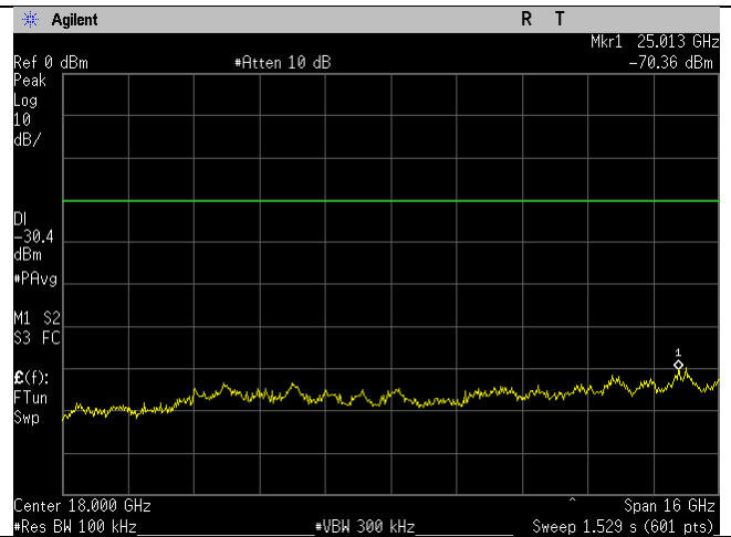
WIFI_Low Ch_2412MHz_20MHz BW_g-mode_- 30dBc_10-26GHz_Port 2.gif
