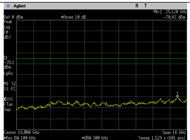
WIFI_High Ch_2452MHz_40MHz BW_n-mode- 30dBc_10-26GHz_Port 2.gif
