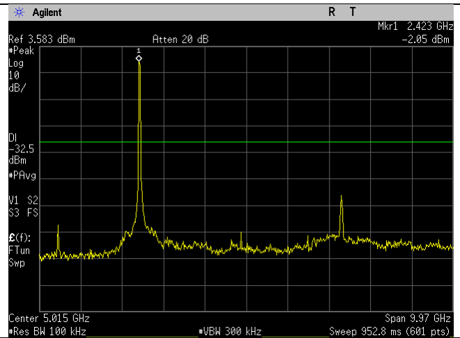
WIFI_Mid Ch_2437MHz_40MHz BW_ax-mode_- 30dBc_30MHz-10GHz_Port 1.gif
