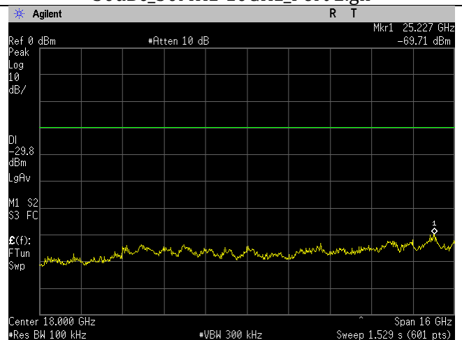
WIFI_Low Ch_2412MHz_20MHz BW_n-mode_-
