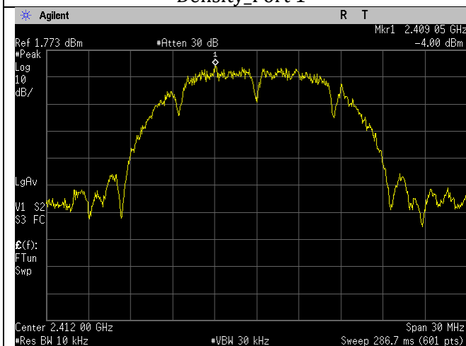
Low Ch_2412MHz_20MHz BW_b-mode_Spectral
