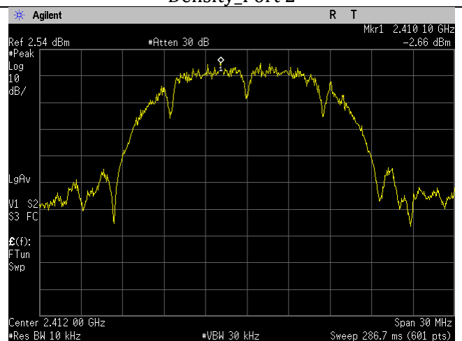
Low Ch_2412MHz_20MHz BW_b-mode_Spectral
