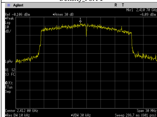
Low Ch_2412MHz_20MHz BW_ax-mode_Spectral
