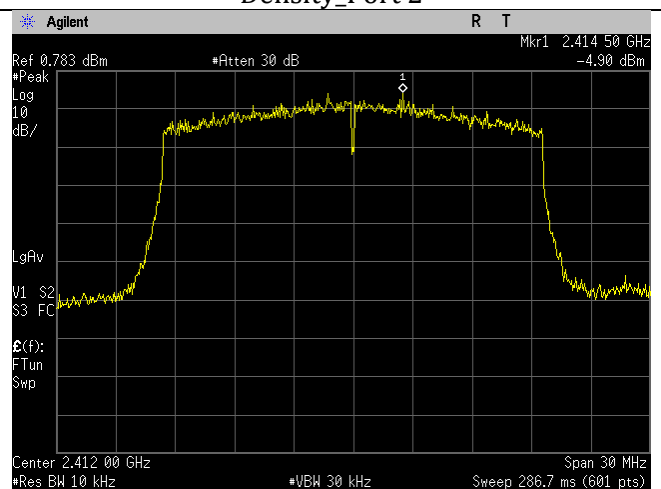
Low Ch_2412MHz_20MHz BW_ax-mode_Spectral
