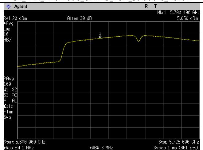
Ch_144_n40mode_UNII-2C_PSD_Straddle_Port 2
