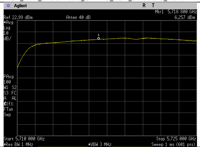
Ch_144_n20mode_UNII-2C_PSD_Straddle_Port 2
