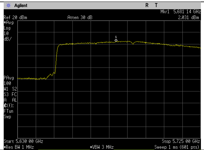
Ch_144_ax80mode_UNII-2C_PSD_Straddle_Port 2
