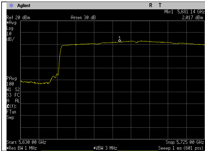
Ch_144_ax80mode_UNII-2C_PSD_Straddle_Port 1
