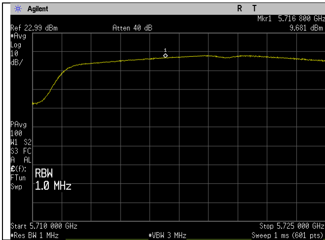
Ch_144_amode_UNII-2C_PSD_Straddle_Port 1
