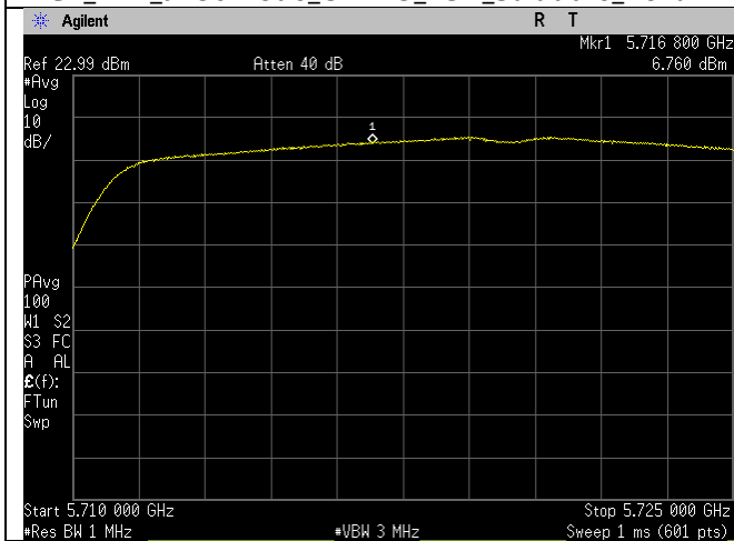
Ch_144_n20mode_UNII-2C_PSD_Straddle_Port 1
