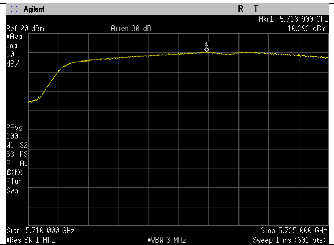
Ch_144_amode_UNII-2C_PSD_Straddle_Port 2
