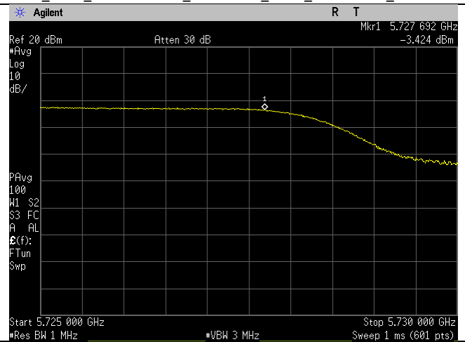
Ch_144_ac80mode_UNII-3_PSD_Straddle_Port 2
