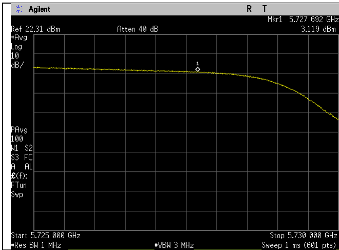
Ch_144_n20mode_UNII-3_PSD_Straddle_Port 1
