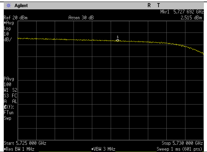
Ch_144_ax20mode_UNII-3_PSD_Straddle_Port 2
