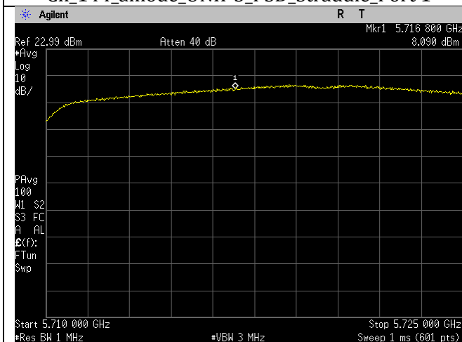
Ch_144_ax20mode_UNII-2C_PSD_Straddle_Port 1
