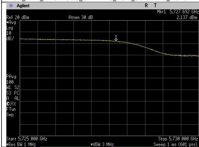
Ch_144_n40mode_UNII-3_PSD_Straddle_Port 1
