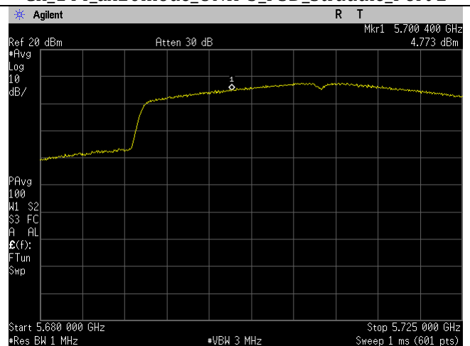
Ch_144_ax40mode_UNII-2C_PSD_Straddle_Port 2
