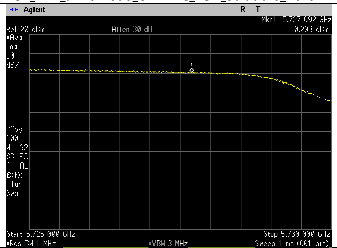
Ch_144_ax40mode_UNII-3_PSD_Straddle_Port 2
