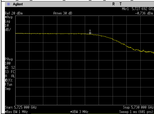
Ch_144_ac80mode_UNII-3_PSD_Straddle_Port 1
