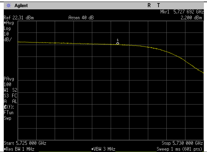
Ch_144_n20mode_UNII-3_PSD_Straddle_Port 2
