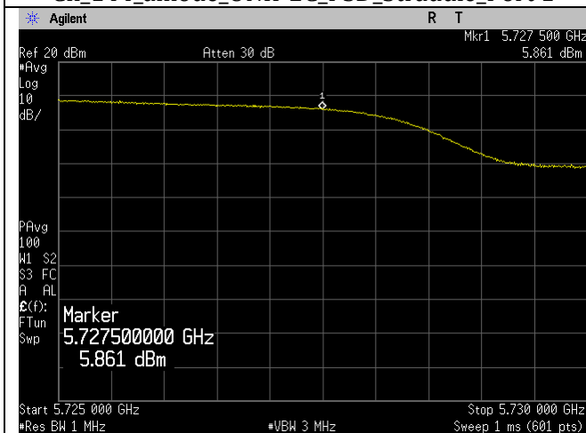
Ch_144_amode_UNII-3_PSD_Straddle_Port 1
