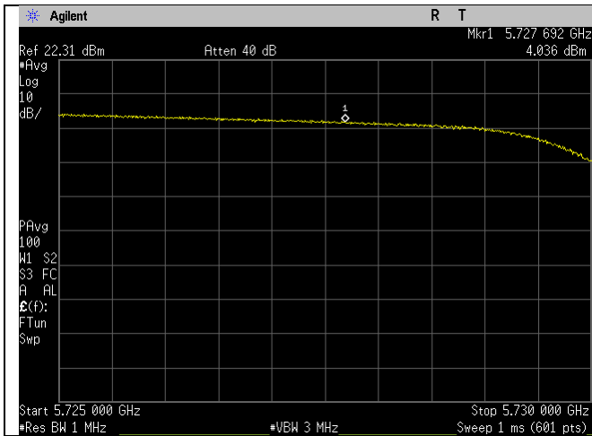
Ch_144_ax20mode_UNII-3_PSD_Straddle_Port 1
