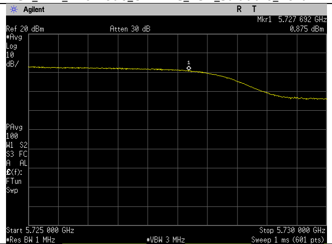
Ch_144_n40mode_UNII-3_PSD_Straddle_Port 2
