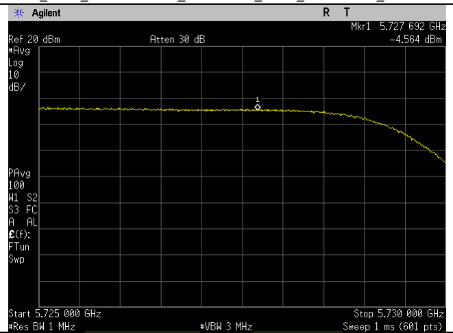
Ch_144_ax80mode_UNII-3_PSD_Straddle_Port 2
