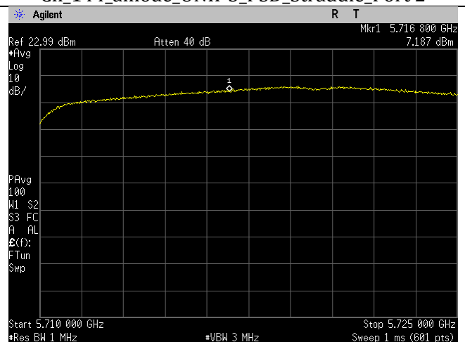
Ch_144_ax20mode_UNII-2C_PSD_Straddle_Port 2
