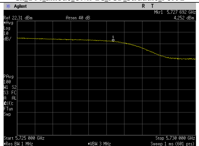
Ch_144_amode_UNII-3_PSD_Straddle_Port 2
