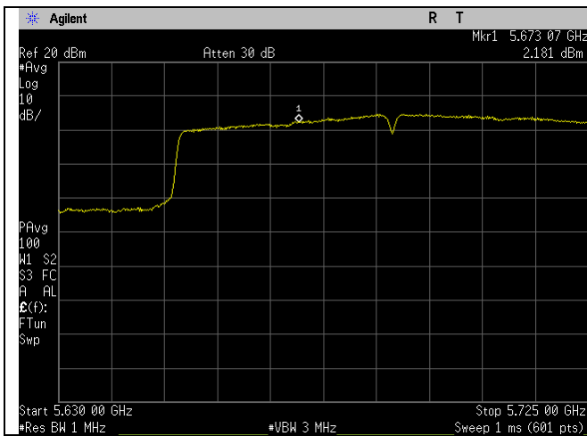
Ch_144_ac80mode_UNII-2C_PSD_Straddle_Port 1
