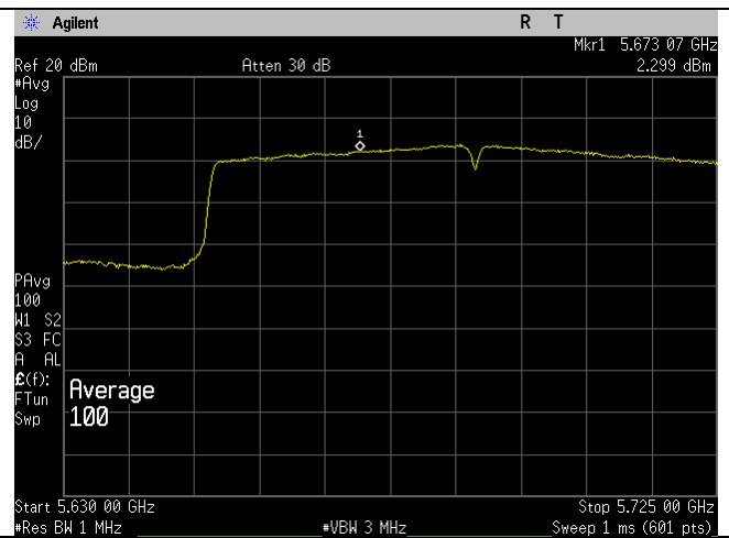
Ch_144_ac80mode_UNII-2C_PSD_Straddle_Port 2
