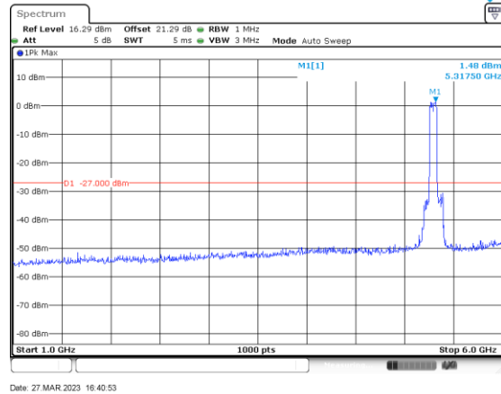
ac80_5290_1000-6000_Ant B
