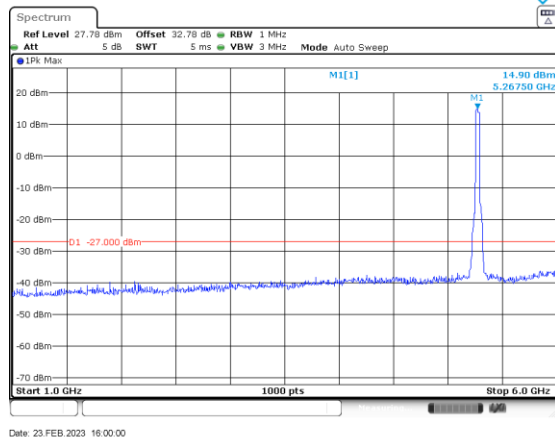
ac/n40_5270_1000-6000_Ant A
