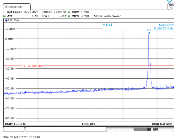
ac/n40_5270_1000-6000_Ant B
