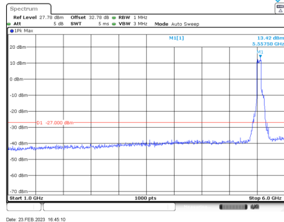
ac80_5530_1000-6000_Ant A
