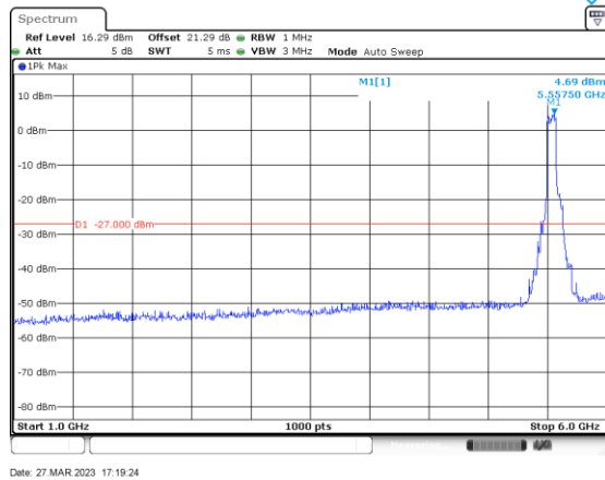
ac80_5530_1000-6000_Ant B
