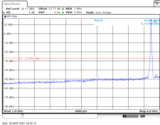
ac/n20_5720_1000-6000_Ant B
