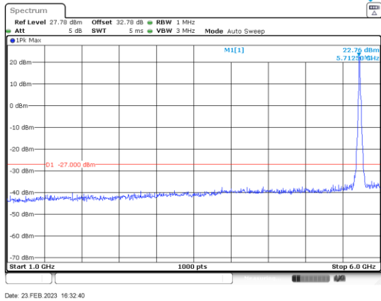
ac/n20_5720_1000-6000_Ant A
