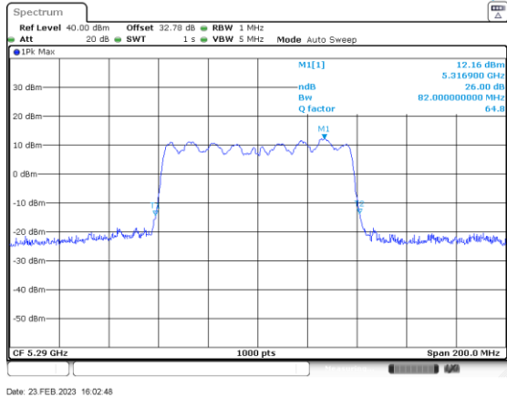
ac80_5290_Ant A
