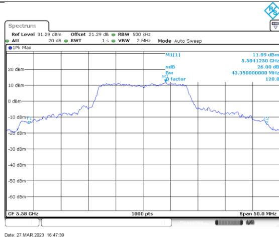
a_5580_Ant B
