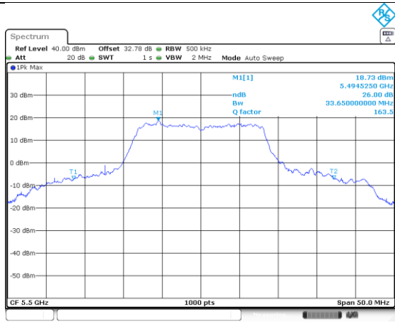
a_5500_Ant A
