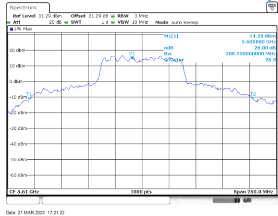
ac80_5610_Ant B
