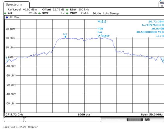
ac/n20_5720_Ant A
