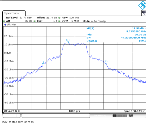
a_5720_Ant B
