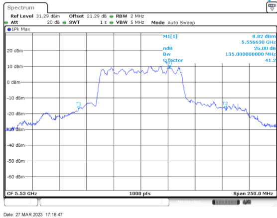
ac80_5530_Ant B
