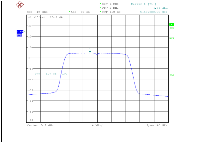
n/ac20_5700_Ant A
