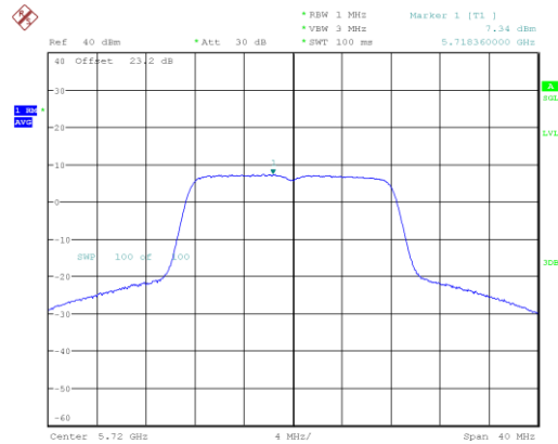
a_5720_Ant A
