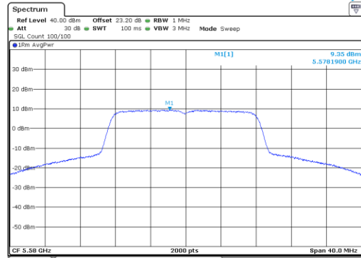
a_5580_Ant B
