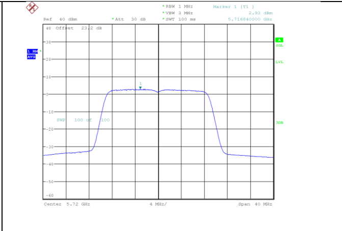
n/ac20_5720_Ant A
