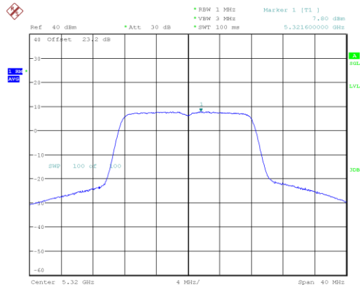
a_5320_Ant A
