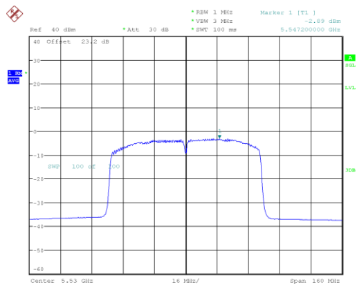
ac80_5530_Ant A
