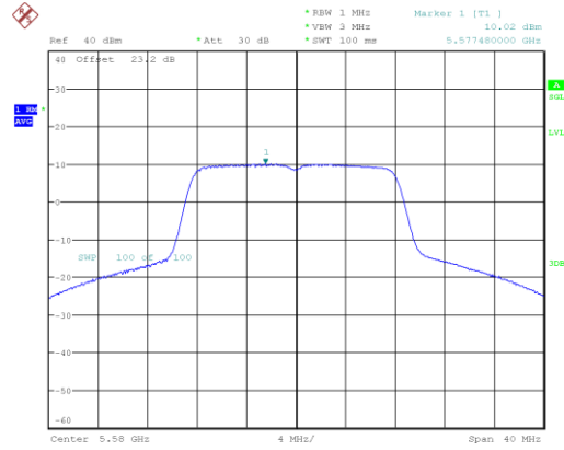
a_5580_Ant A
