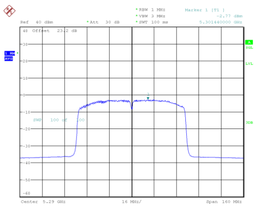
ac80-5290_Ant B
