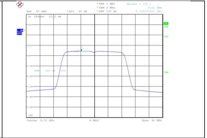
n/ac20_5720_Ant B
