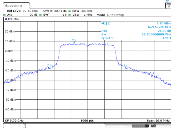
a_5720_Ant A
