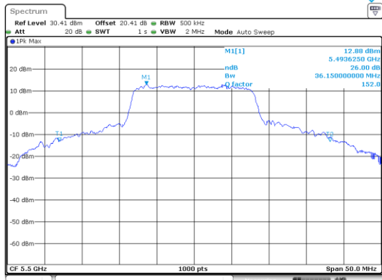
a_5500_Ant B
