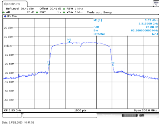
ac80_5530_Ant A
