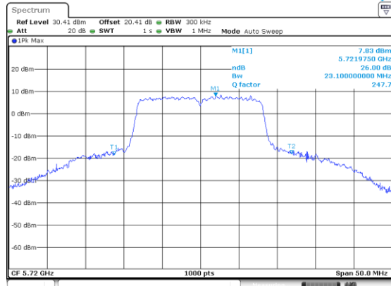
a_5720_Ant B
