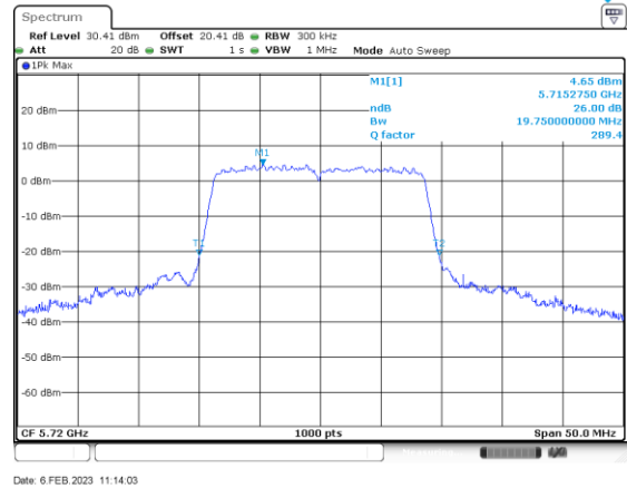
n/ac20_5720_Ant B
