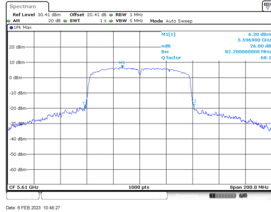
ac80_5610_Ant A
