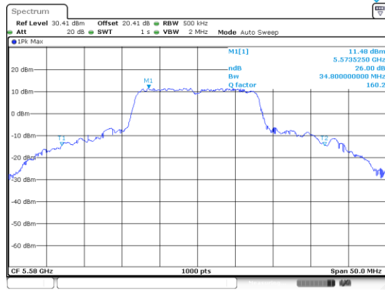
a_5580_Ant A
