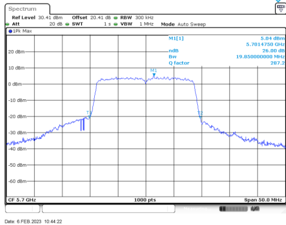
n/ac20_5700_Ant A
