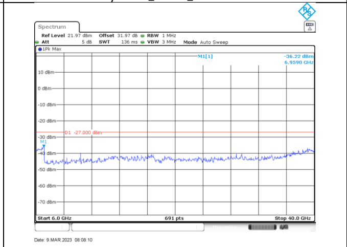
n/ac20_5720_6000-40000
