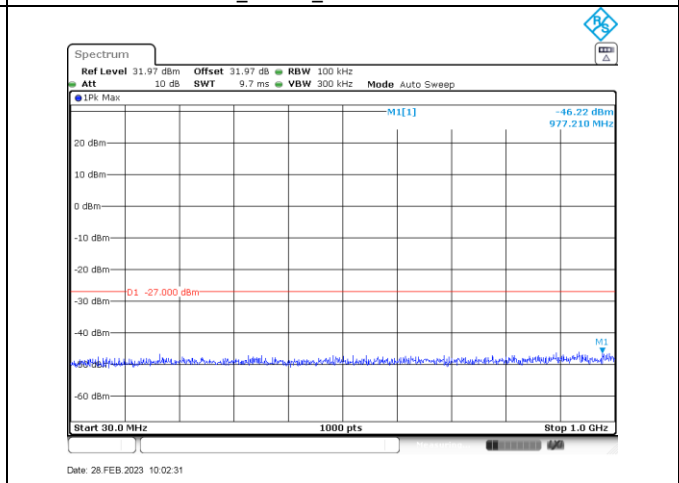
a_5280_30-1000
