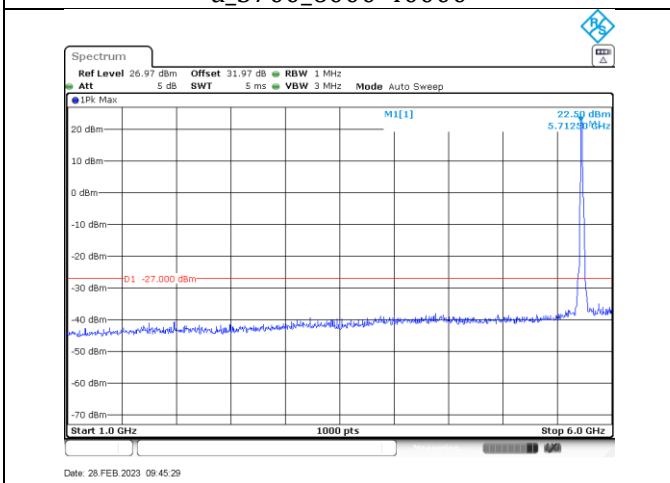
a_5720_1000-6000
