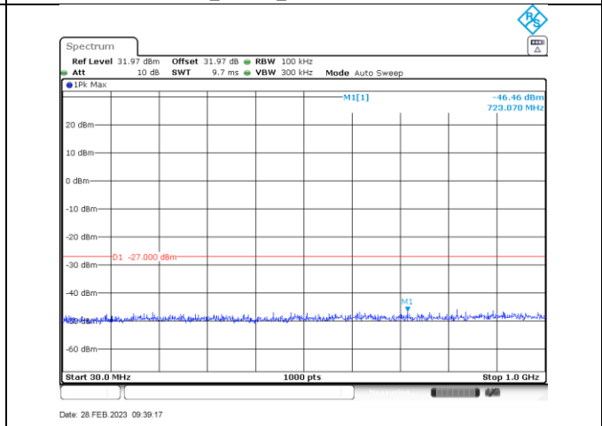
a_5580_30-1000
