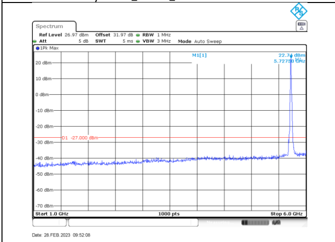
n/ac20_5720_1000-6000
