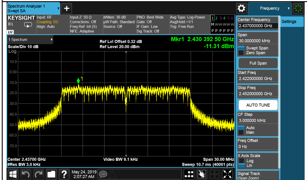
802.11n-HT20 2437MHz
