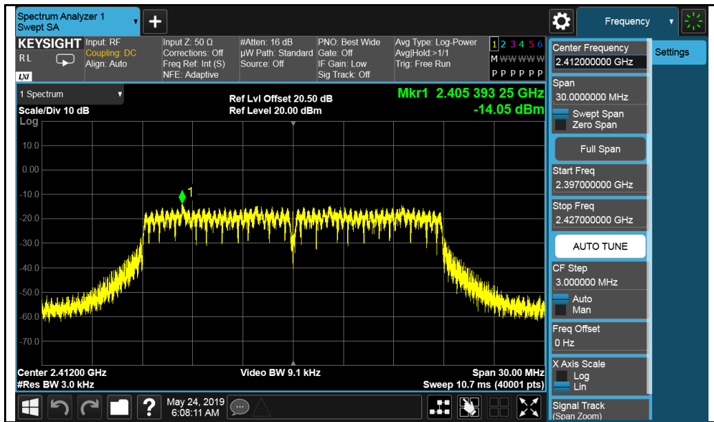
802.11n-HT20 2412MHz
