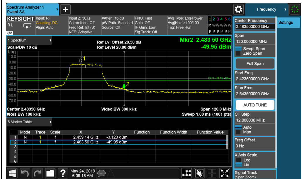
802.11n-HT20-2462MHz
