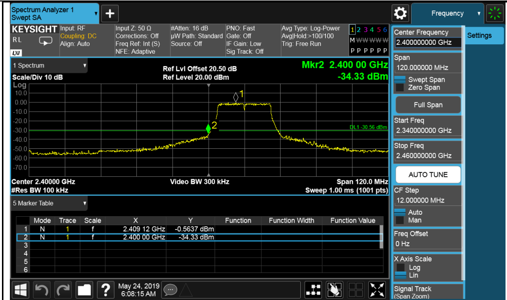
802.11n-HT20-2412MHz
