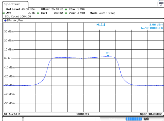
a_5700_Ant B
