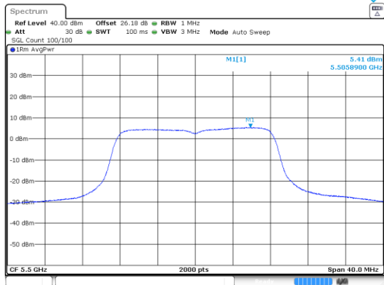
a_5500_Ant B
