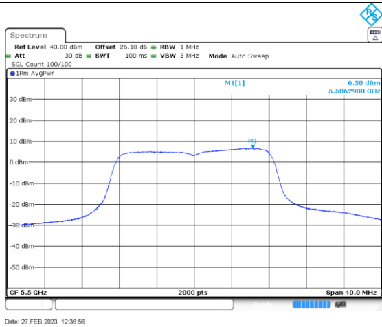
a_5500_Ant A
