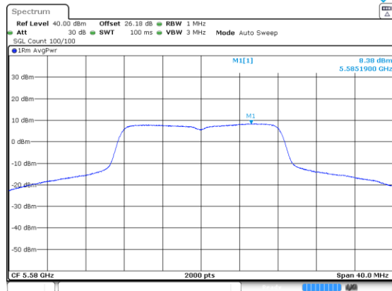
a_5580_Ant B
