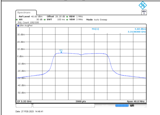
a_5320_Ant A
