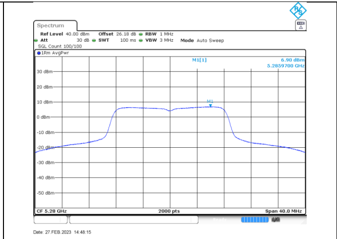
a_5280_Ant A
