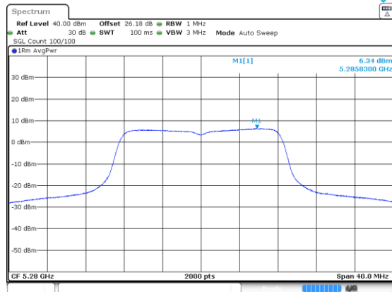
a_5280_Ant B
