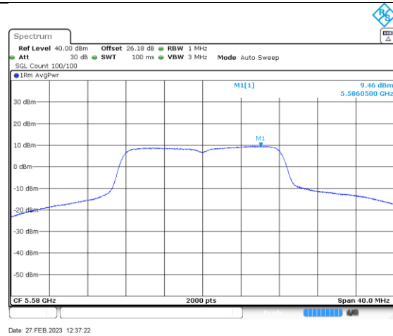
a_5580_Ant A
