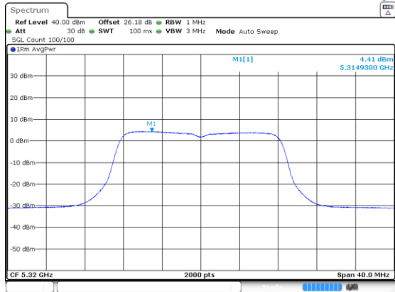
a_5320_Ant B
